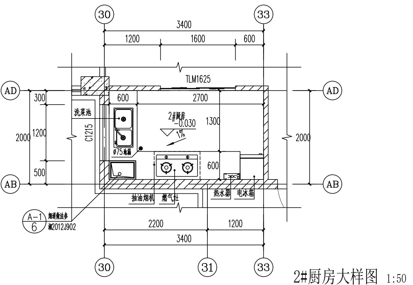
2#厨房大样图 1:50
