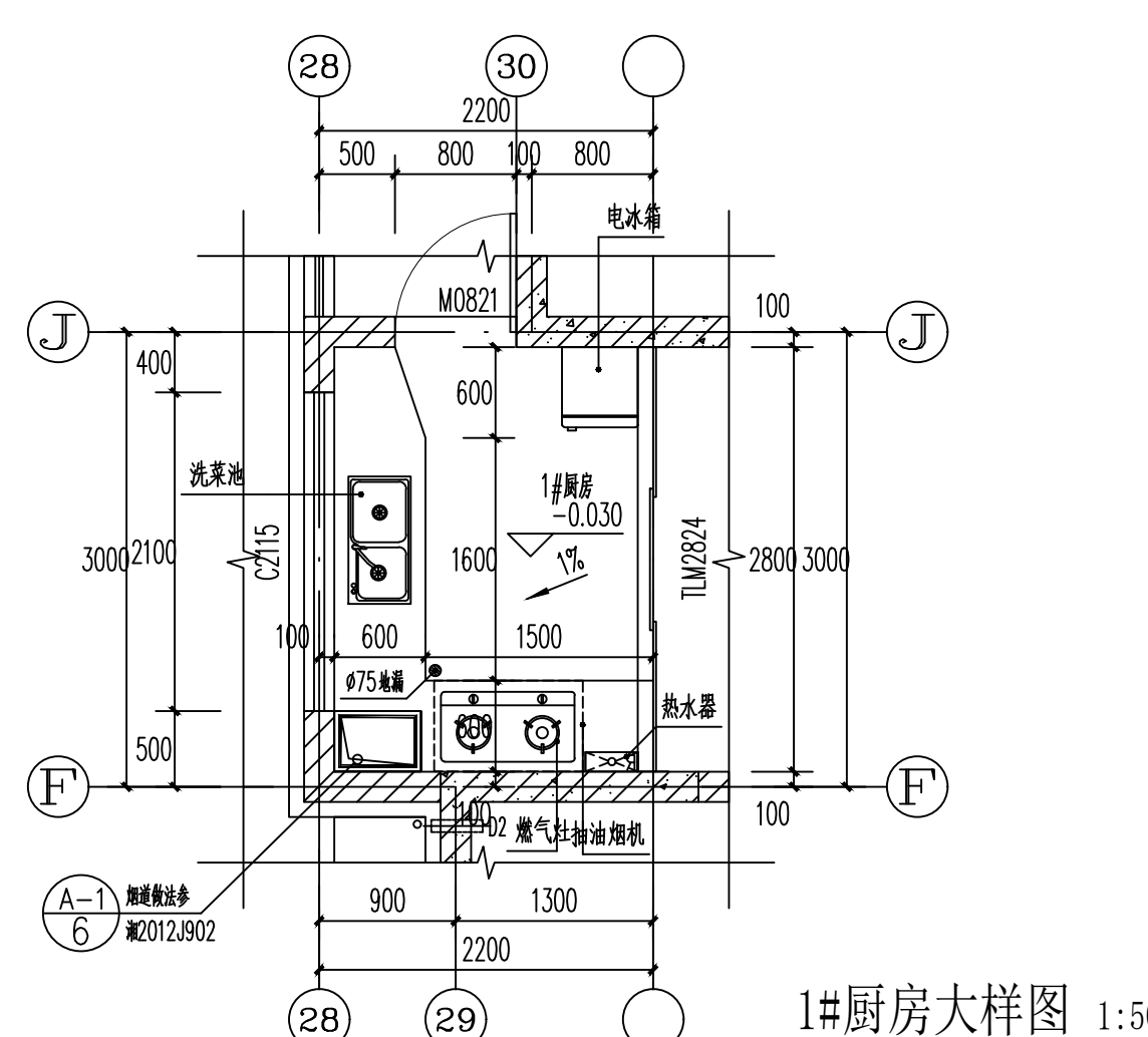
1#厨房大样图 1:50
