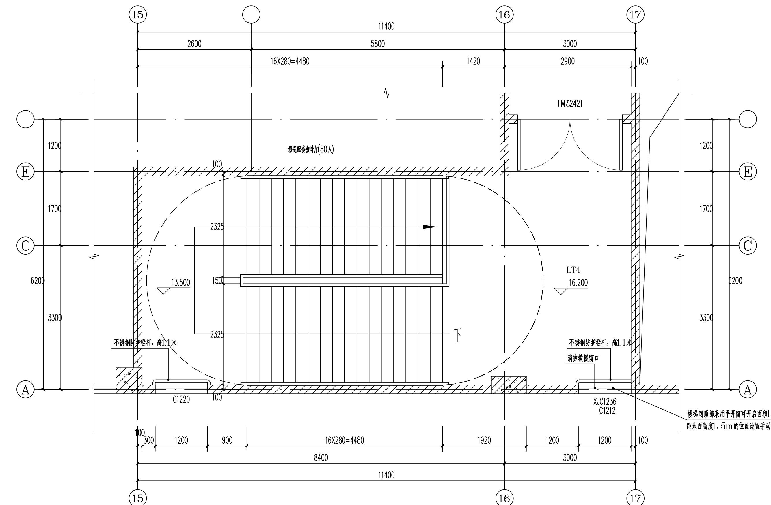
LT4楼梯间四层平面图 1:50
