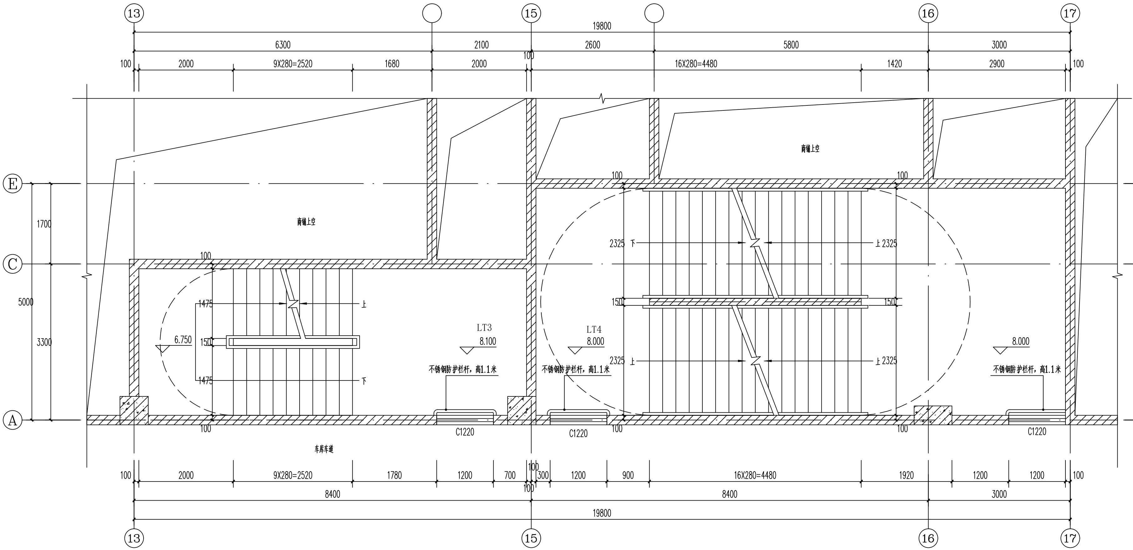
LT3、LT4楼梯间H=8.100处平面图 1:50
