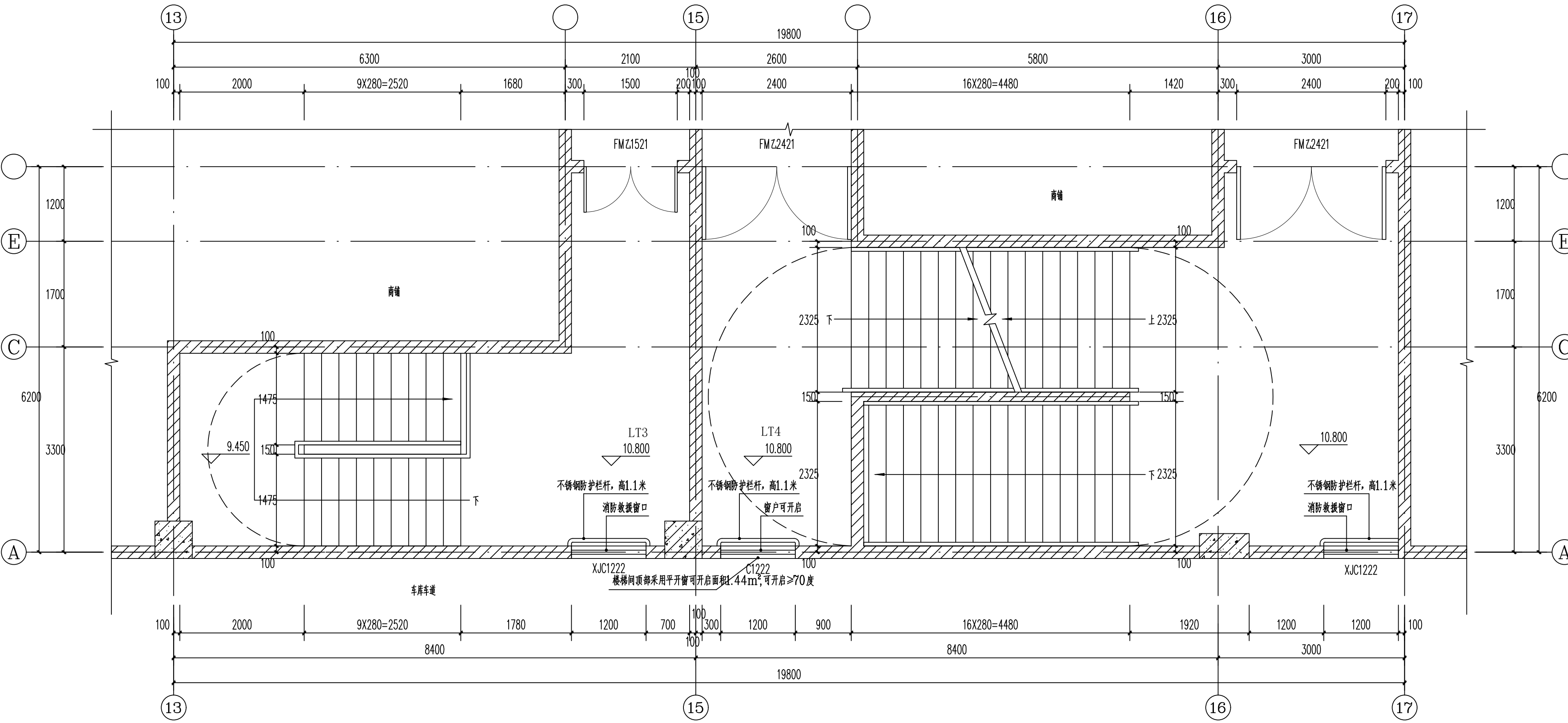
LT3、LT4楼梯间三层平面图 1:50
