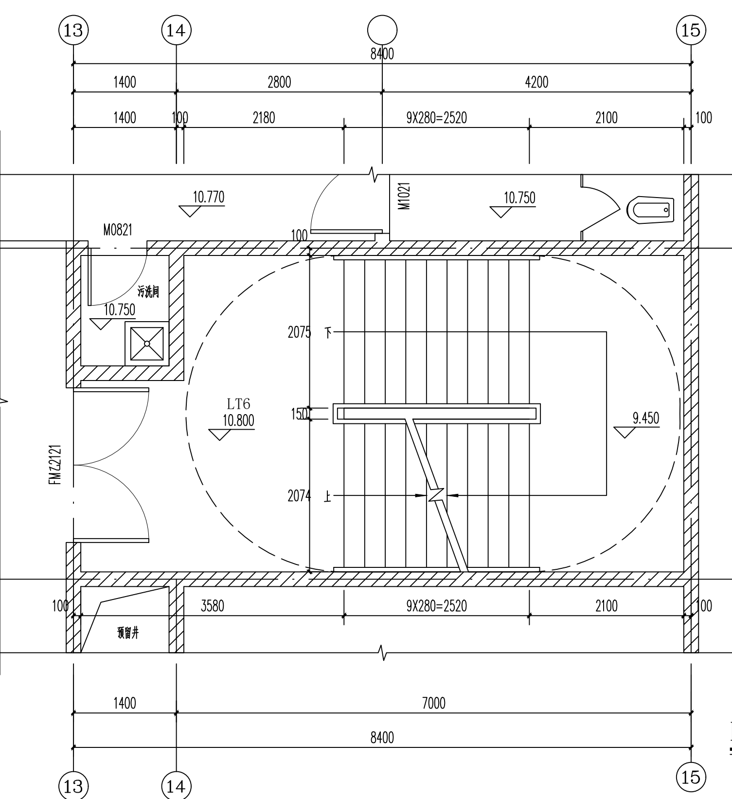
LT6楼梯间三层平面图 1:50
