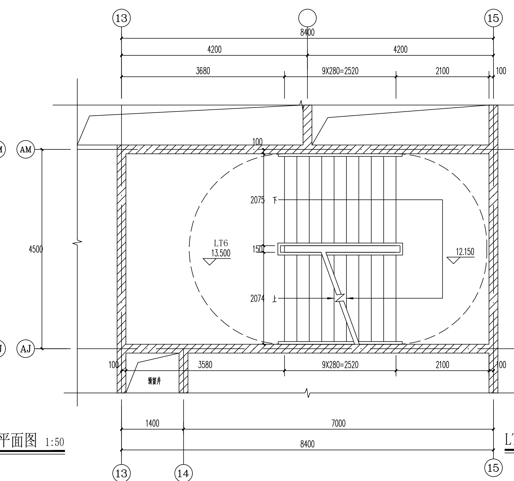
LT6楼梯间屋顶风井平面图 1:50
