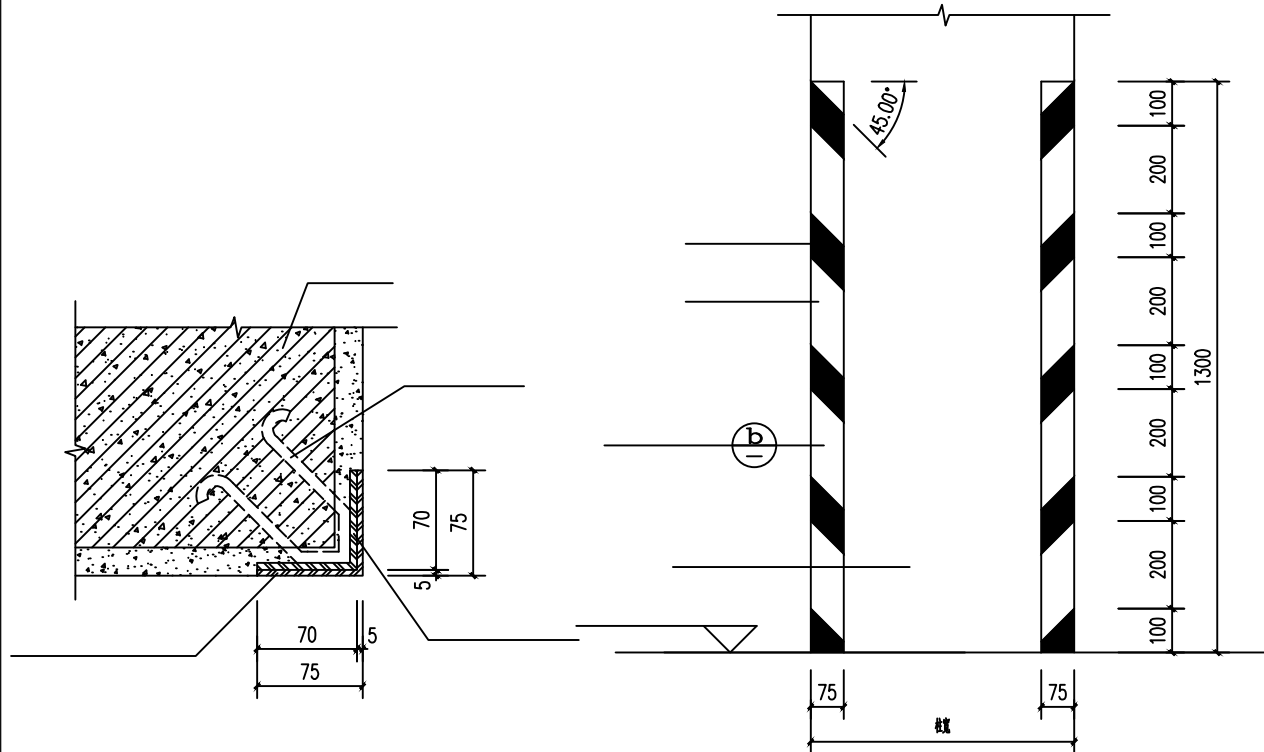
⑤ 车库墙柱防撞保护节点 1:5
