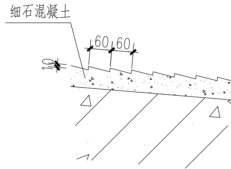
⑥ 车道防滑礅碯详图 1:5
