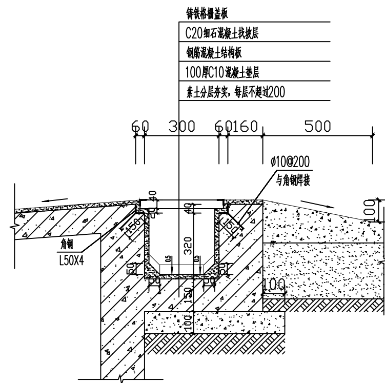
① 车道室外地面截水沟大样 1:25
