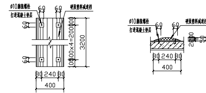
④ 塑料减速档 1:25
