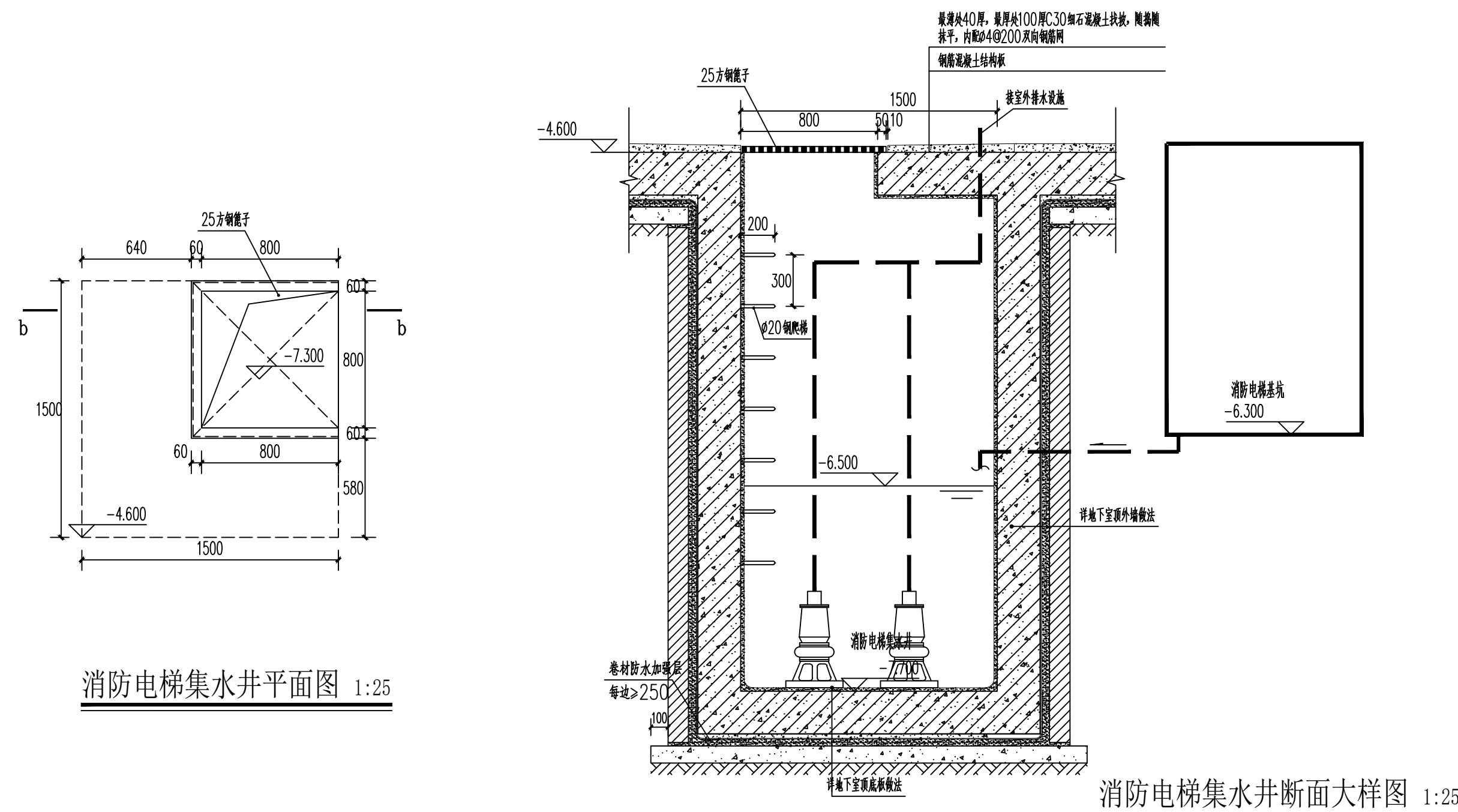
⑩消防电梯集水井大样图 1:25
