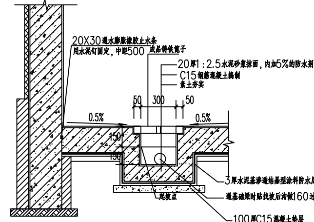
③ 300宽排水沟大样 1:25
