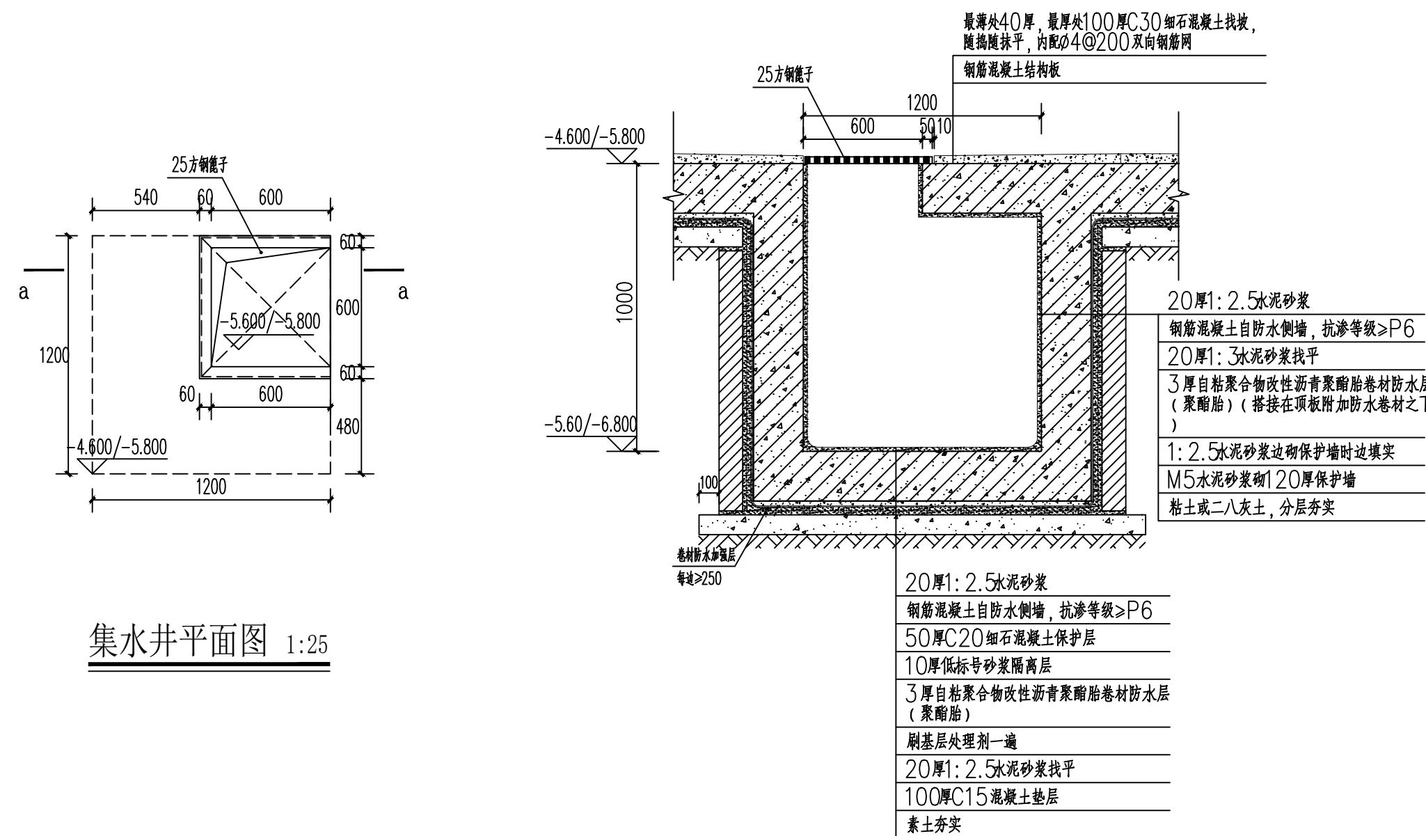
⑨ 集水井大样图 1:25
