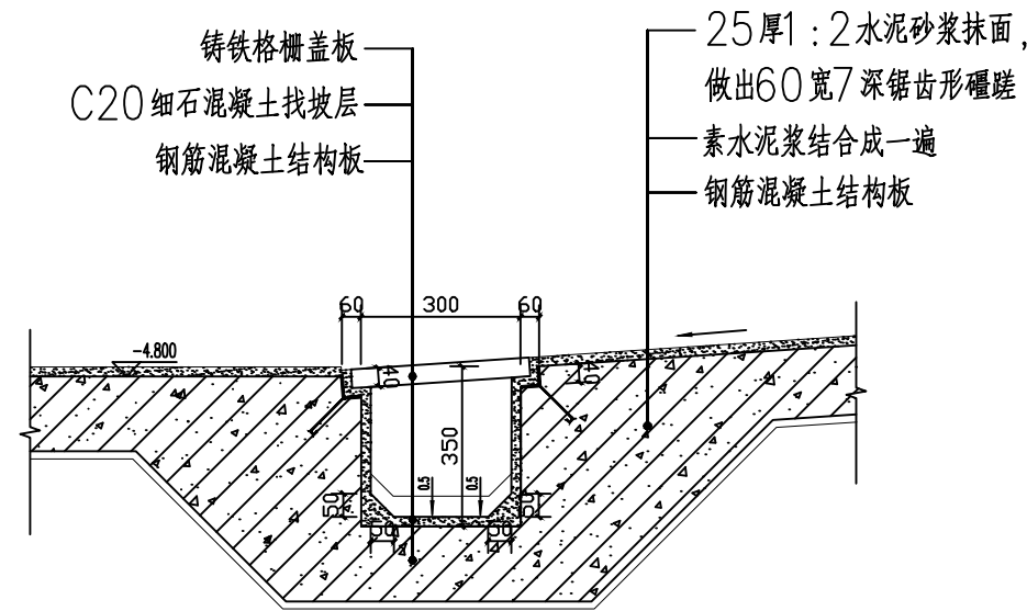
② 车道室内地面截水沟大样 1:25
