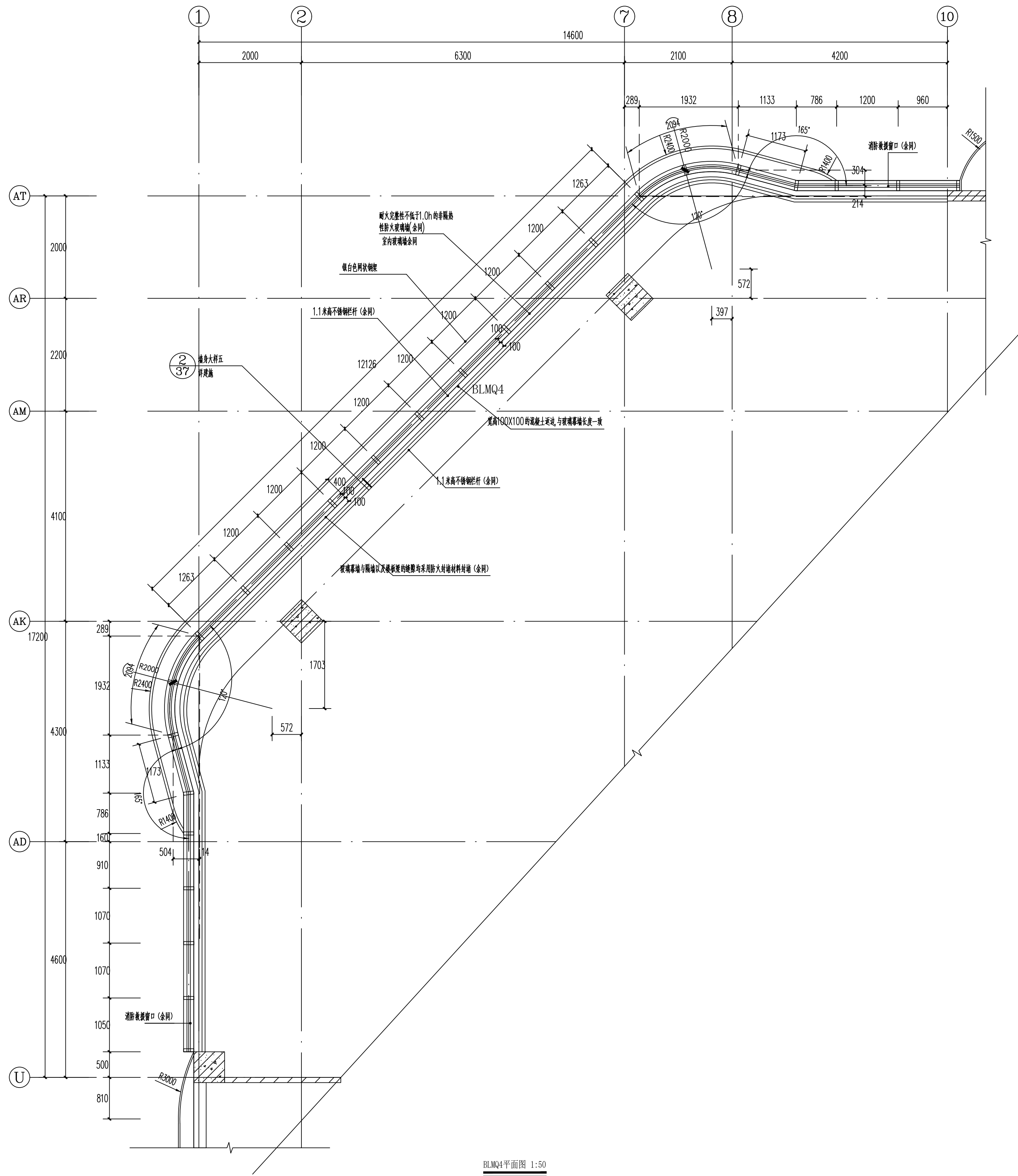
BLMQ4平面图 1:50
