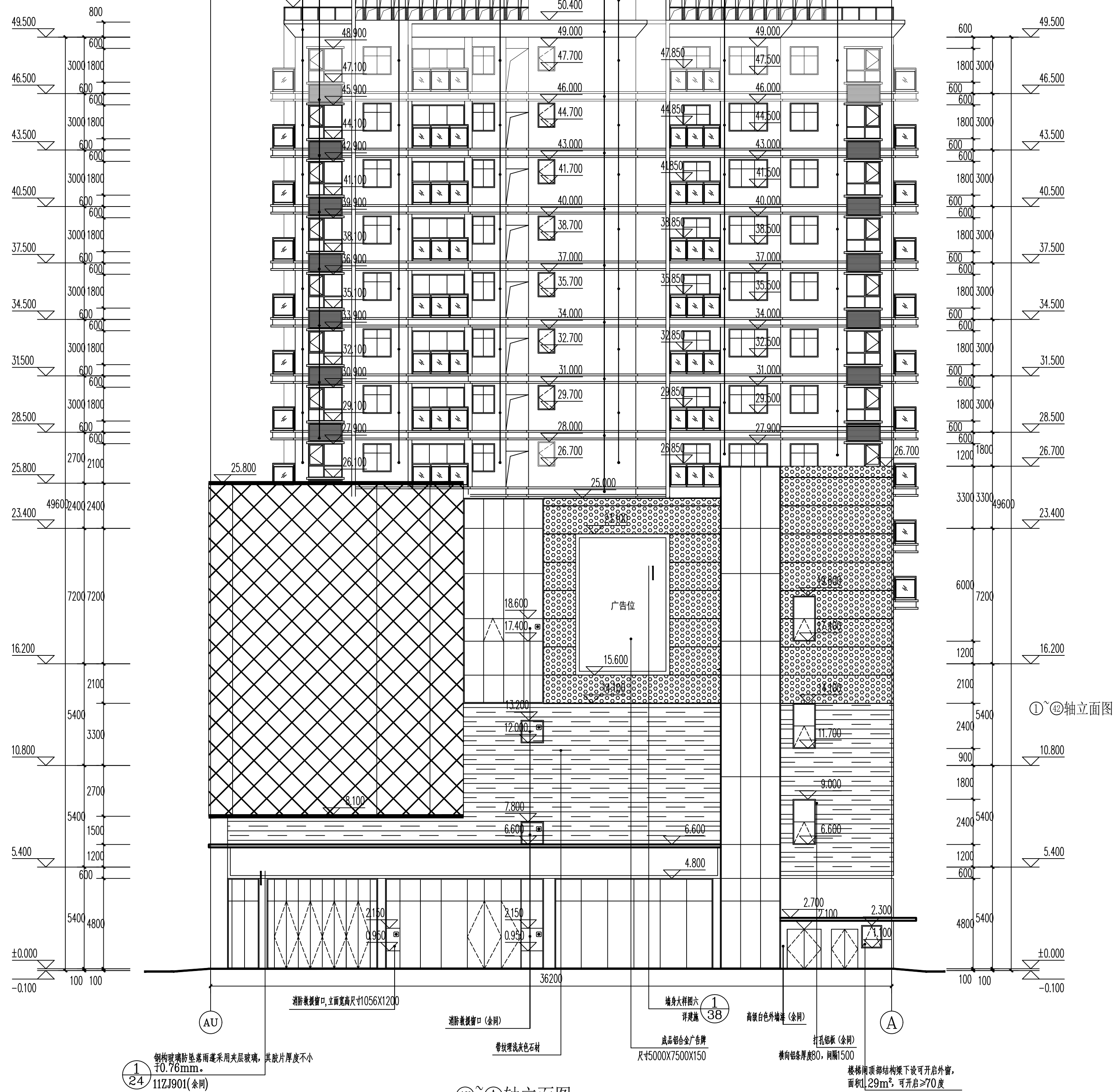
⑩~①轴立面图 1:150
