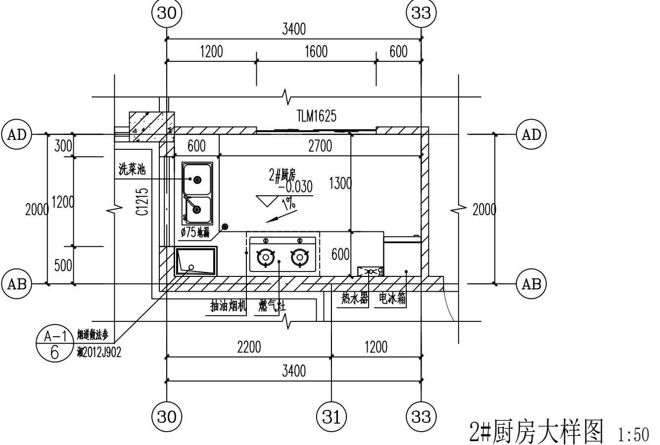
2#厨房大样图 1:50
