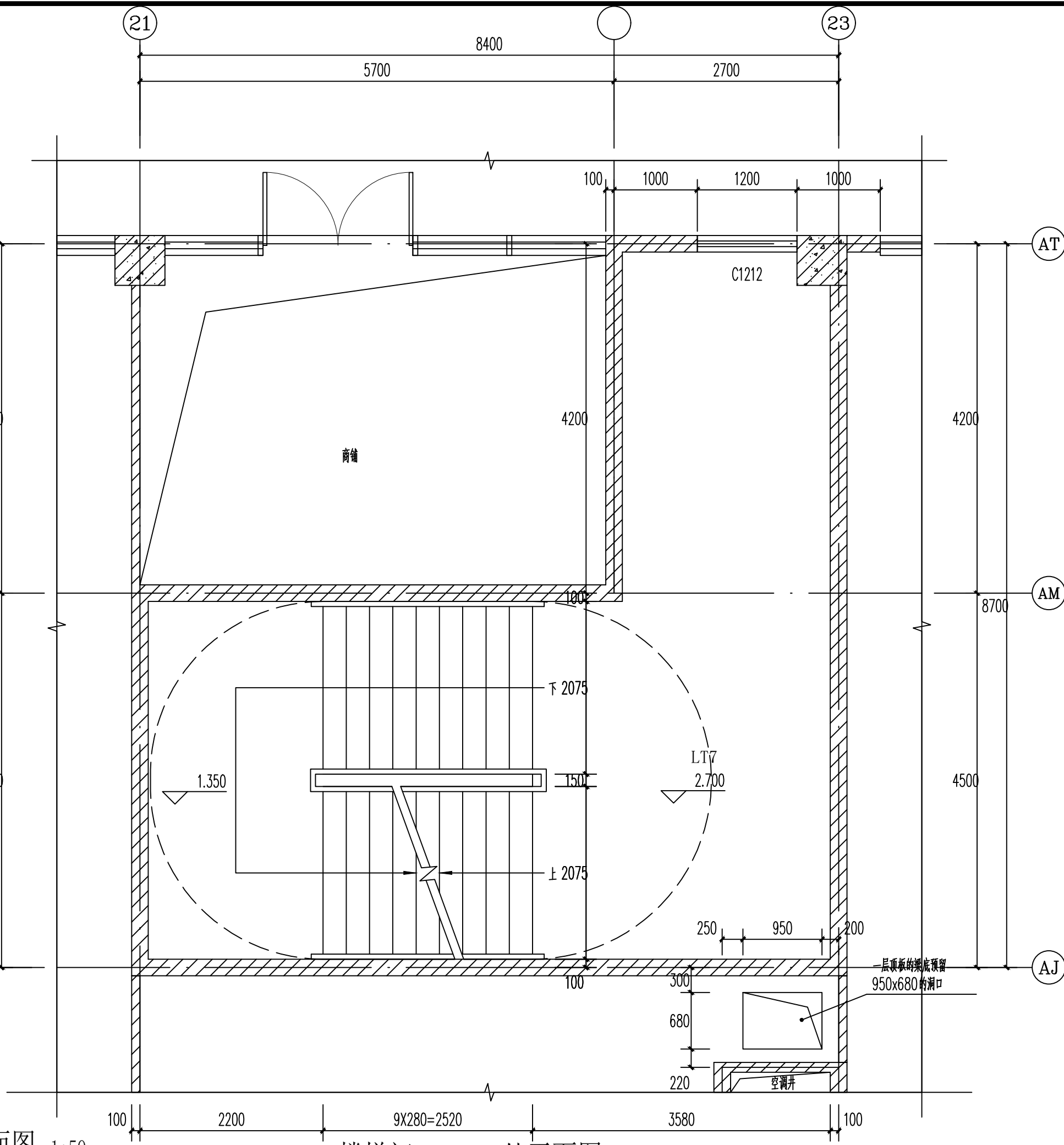
LT7楼梯间H=2.700处平面图 1:50
