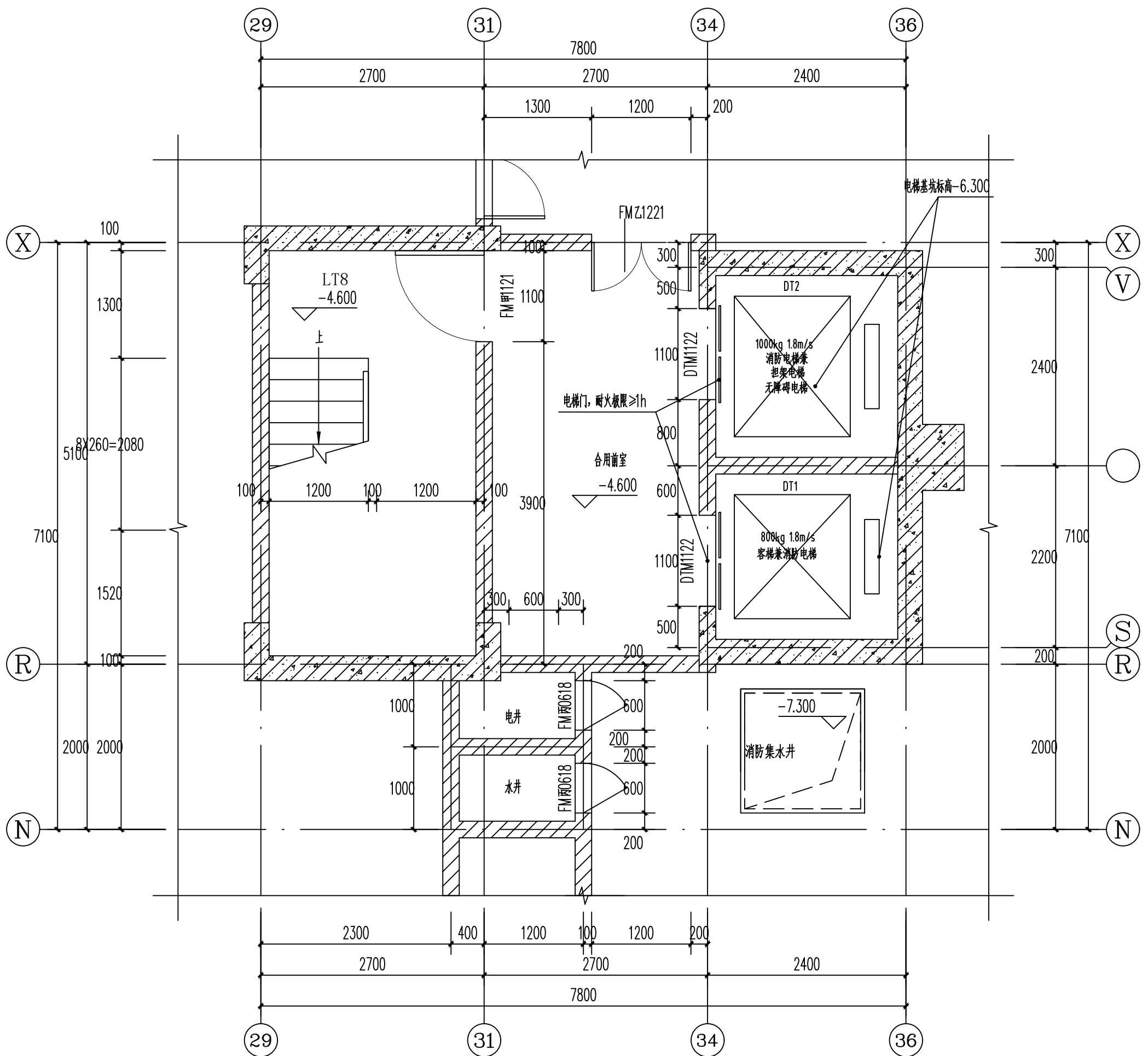
LT8楼梯间负一层平面图 1:50
