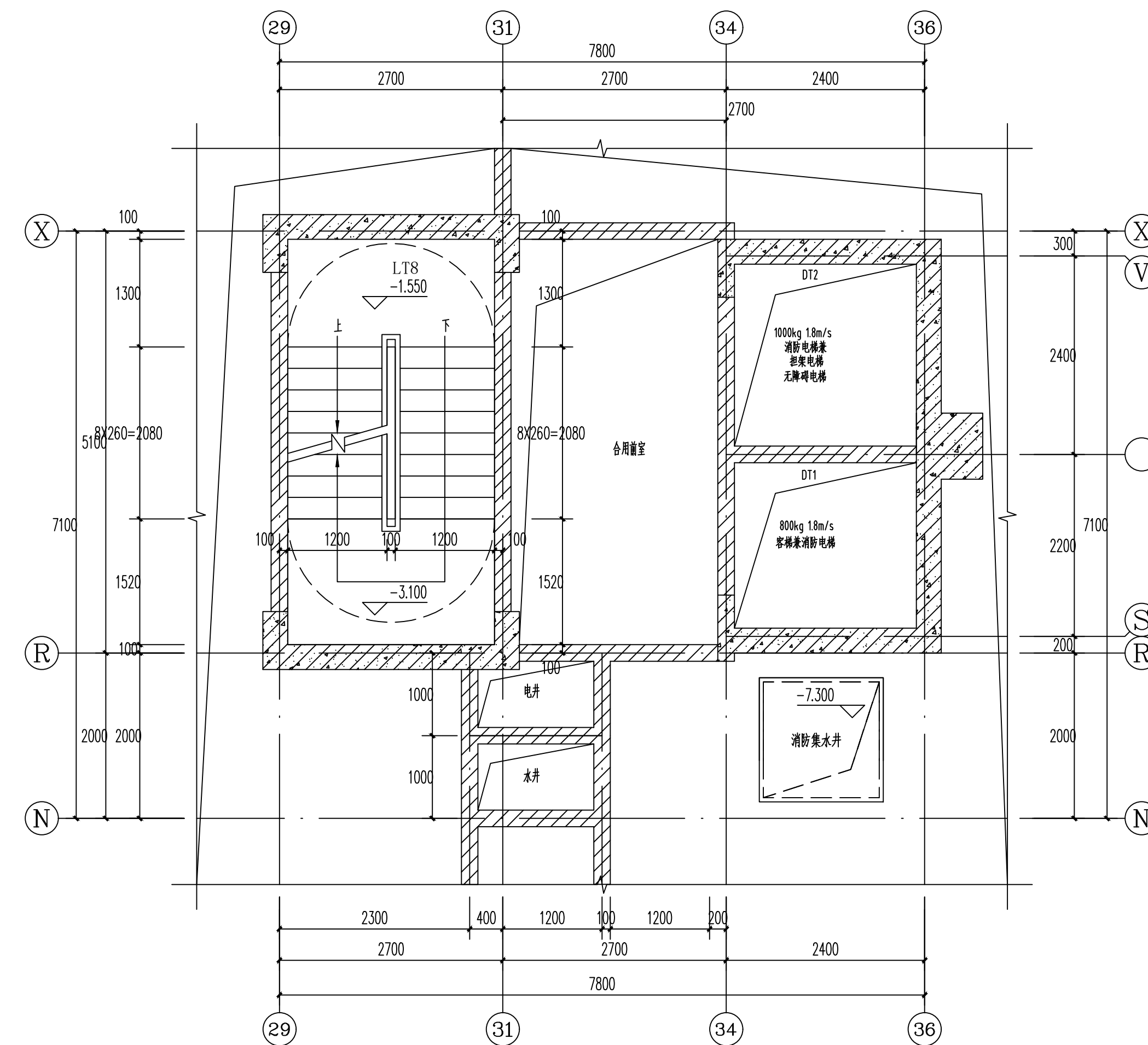
LT8楼梯间H=-1.550处平面图 1:50
