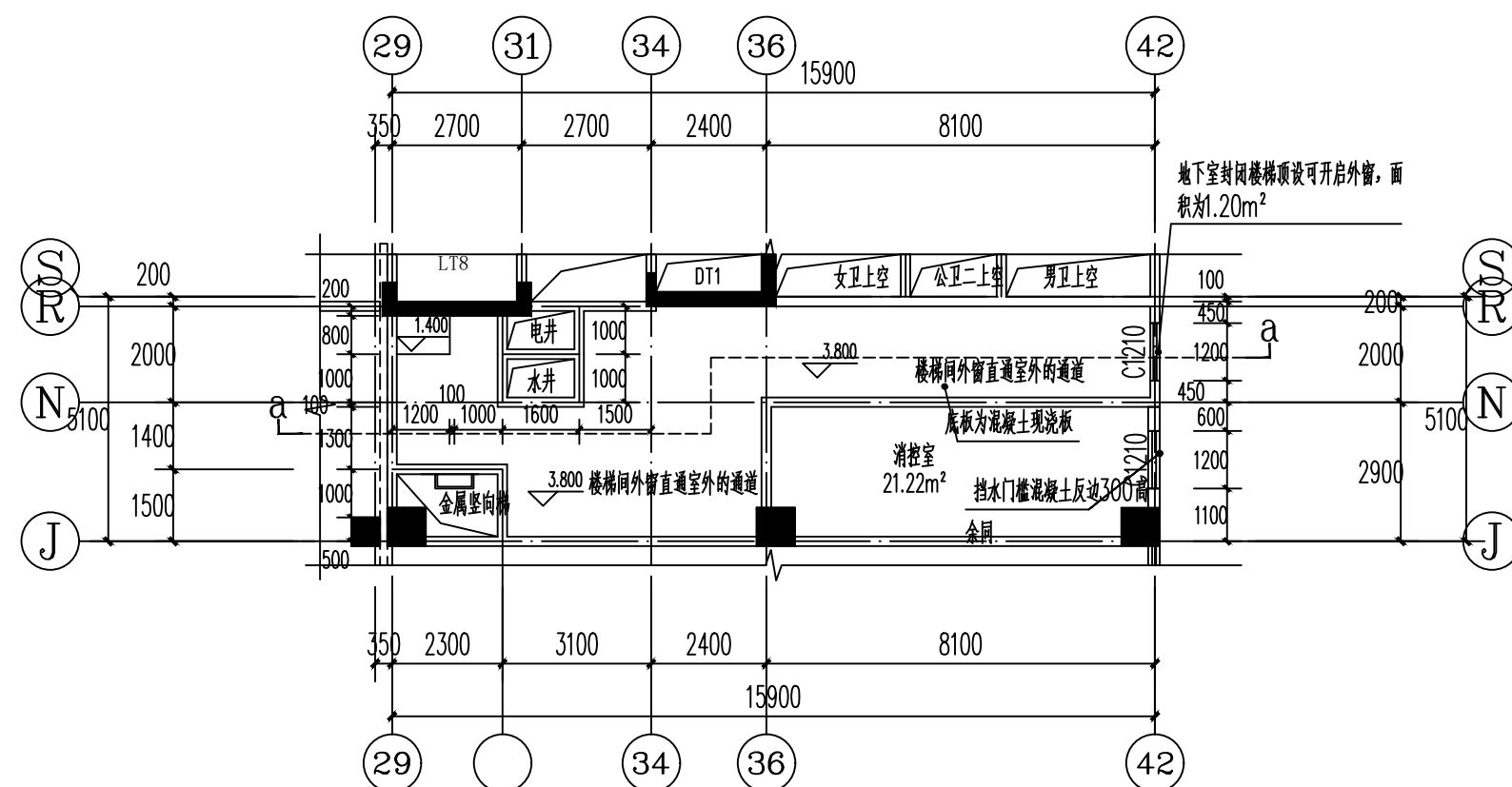
室外通道夹层平面图 1:150 注: a-a剖面图详IS-25
