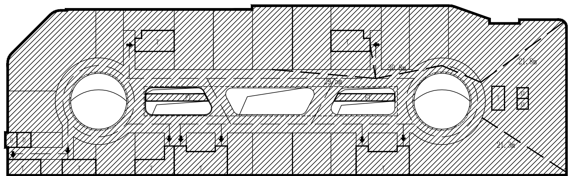
二层防火分区示意图 1:500
