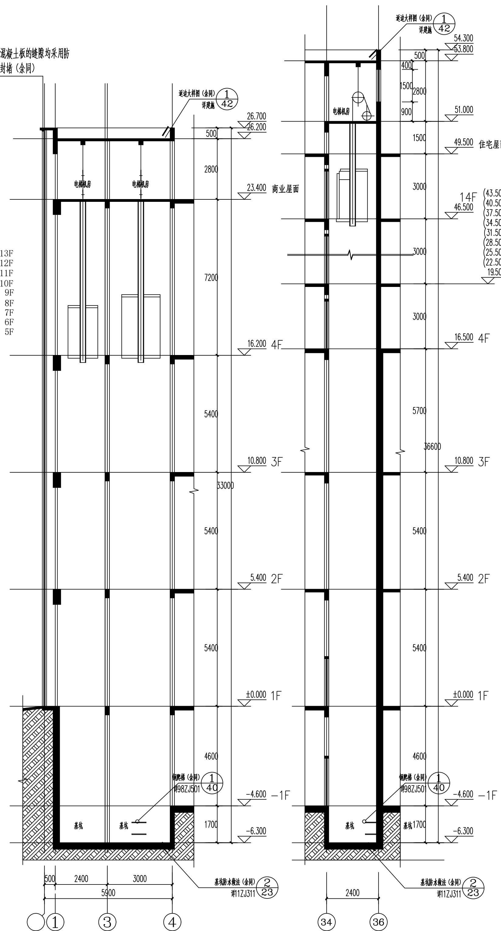
A-A断面图 1:100
