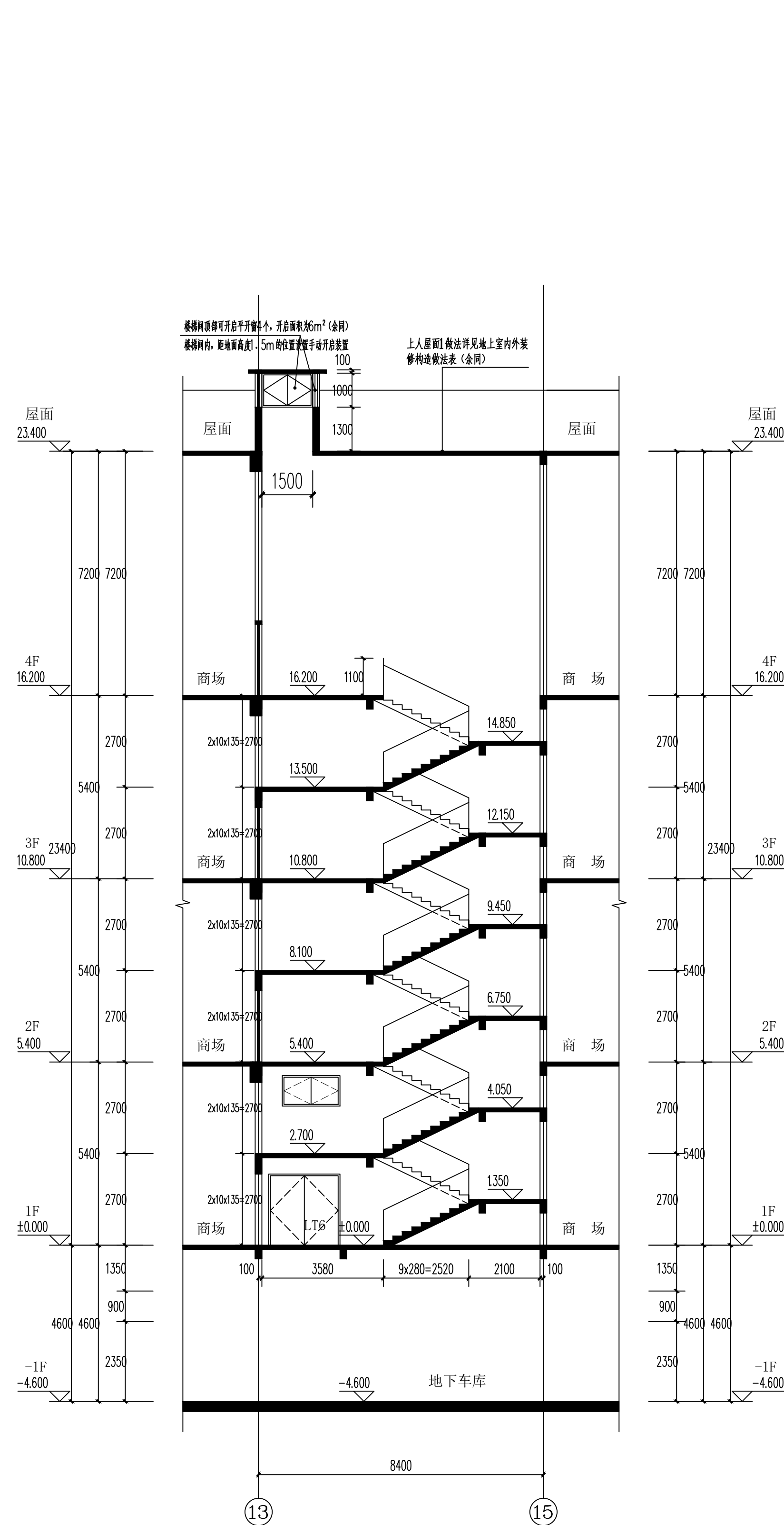
2-2剖面图 1:100
