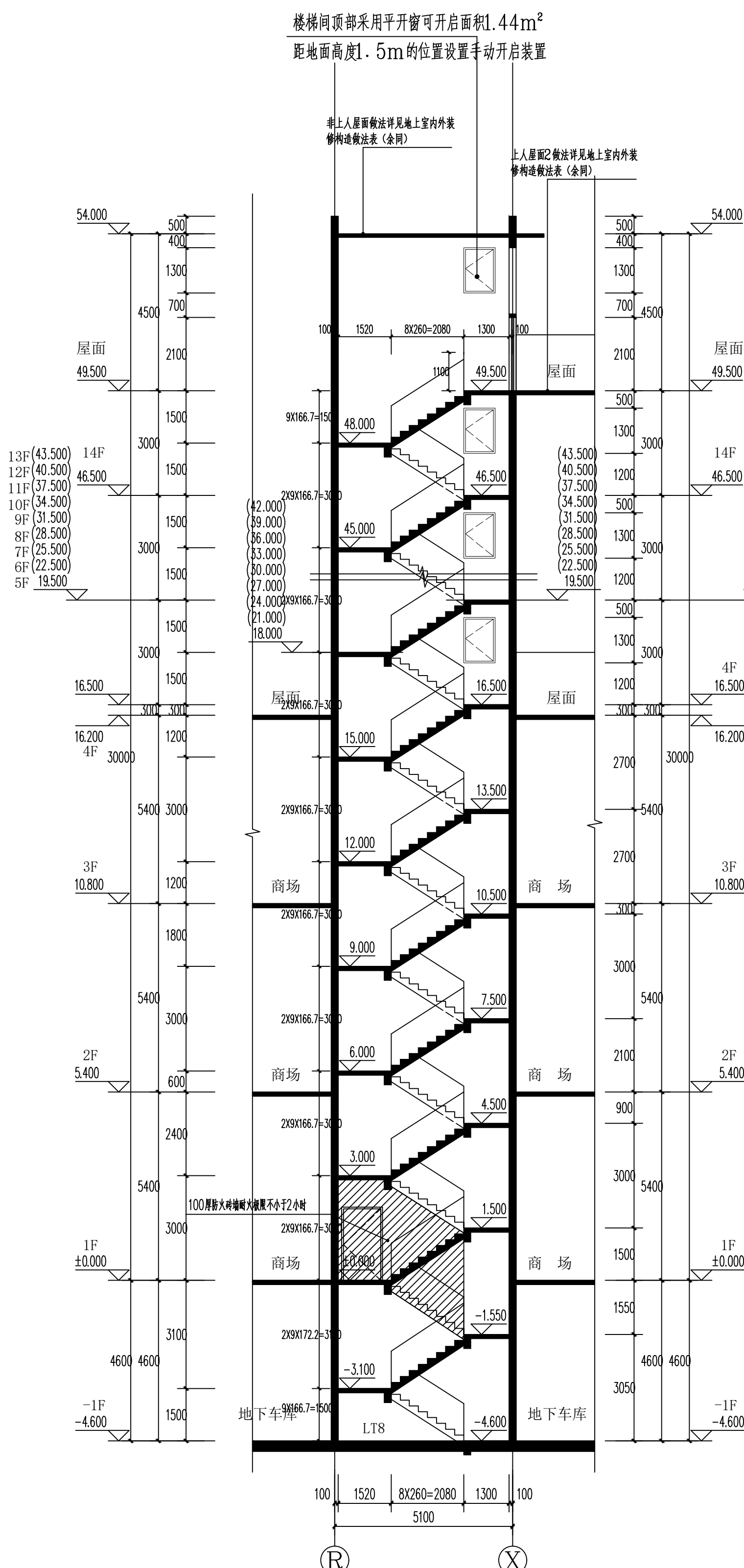
4-4剖面图 1:100
