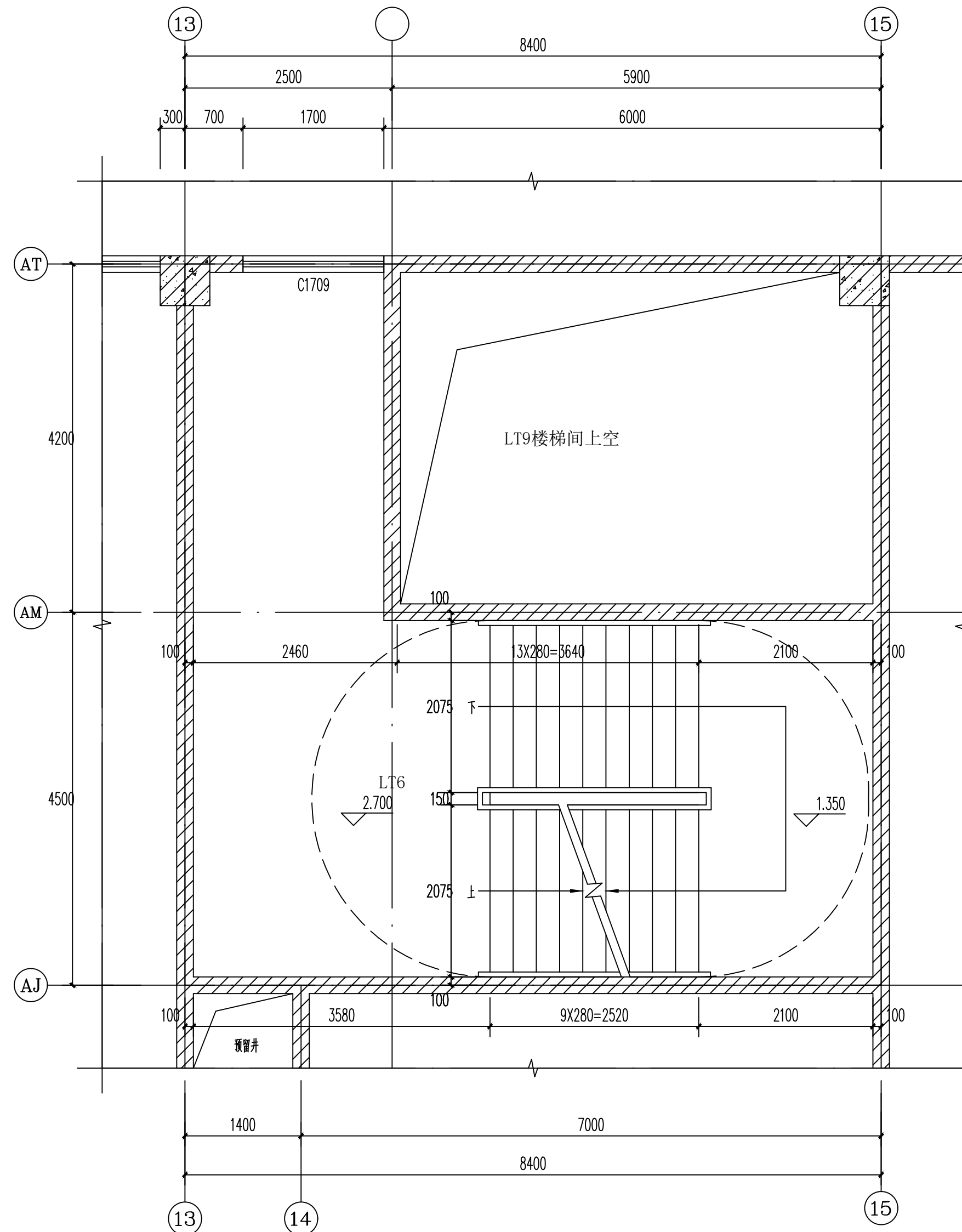
LT6楼梯间H=2.700处平面图 1:50
