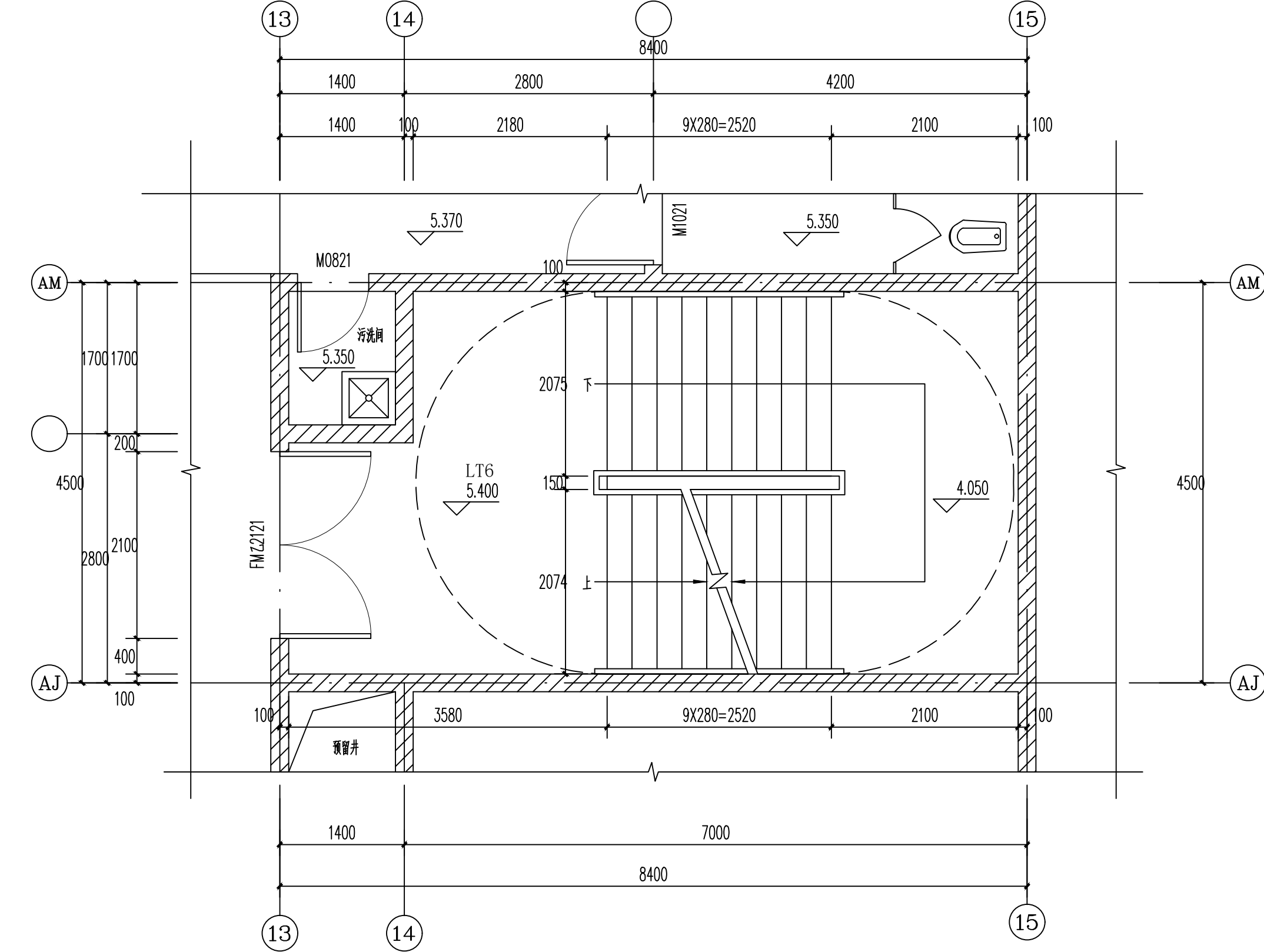
LT6楼梯间二层平面图 1:50
