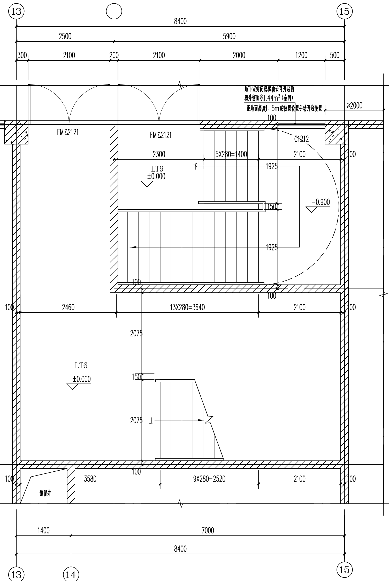
LT6、LT9楼梯间一层平面图 1:50
