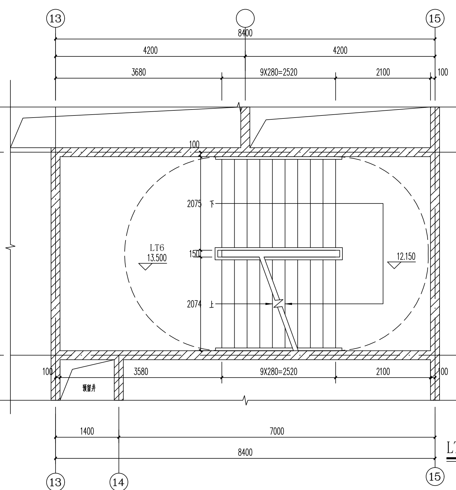
LT6楼梯间三层平面图 1:50
