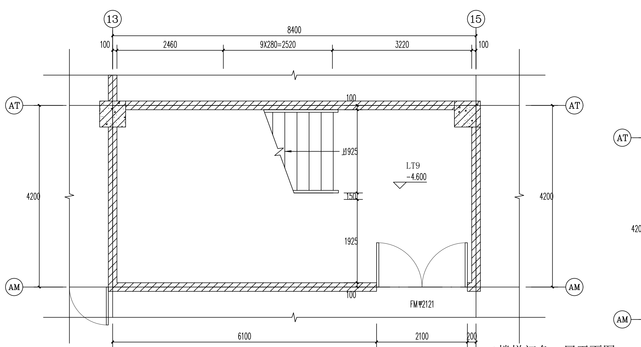
LT9楼梯间负一层平面图 1:50
