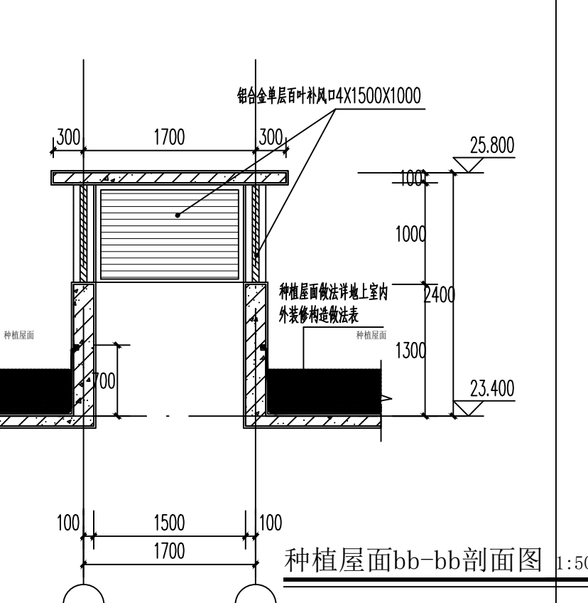
种植屋面bb-bb剖面图 1:50
