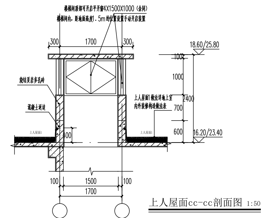
上人屋面cc-cc剖面图 1:50
