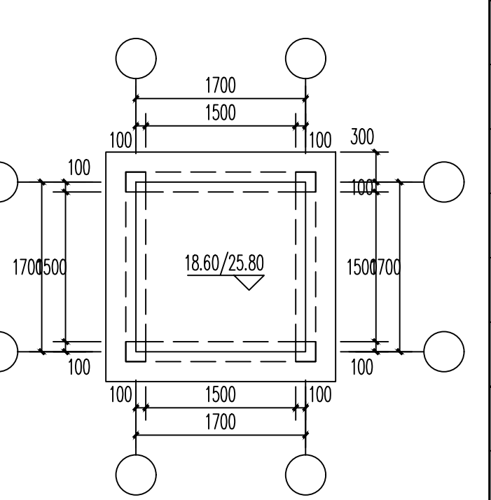
楼梯间风井出屋顶部平面图 1:50
