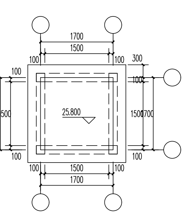
送风井出屋顶部平面图 1:100
