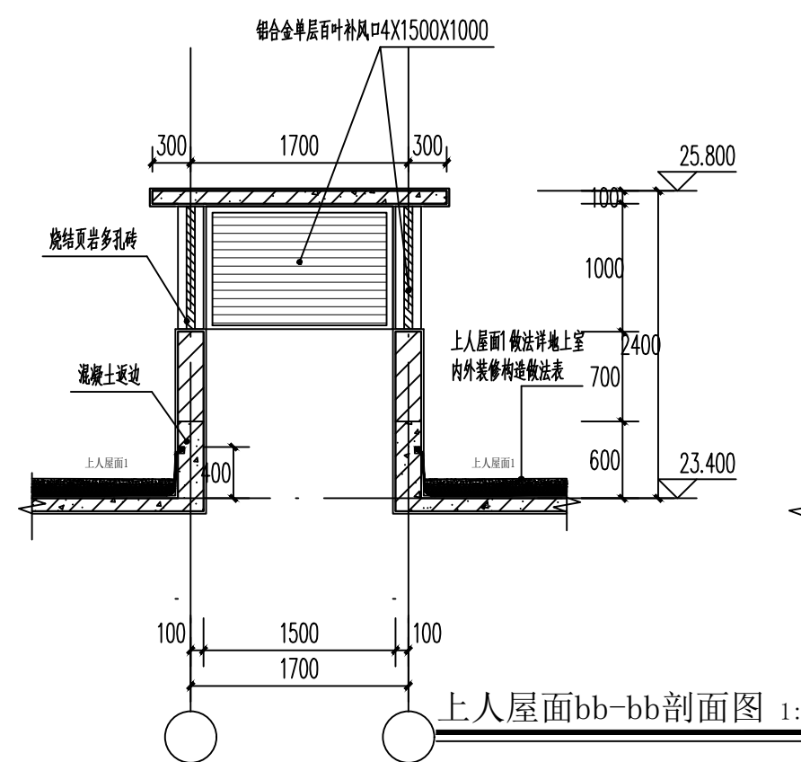
上人屋面bb-bb剖面图 1:50
