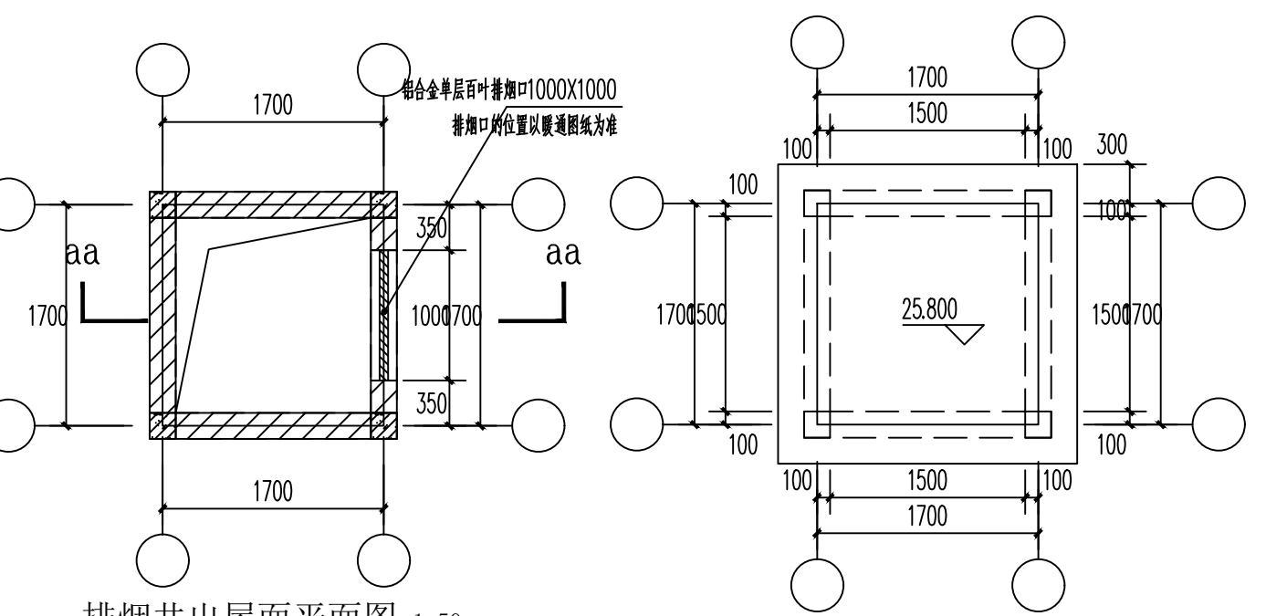
排烟井出屋顶部平面图 1:50
