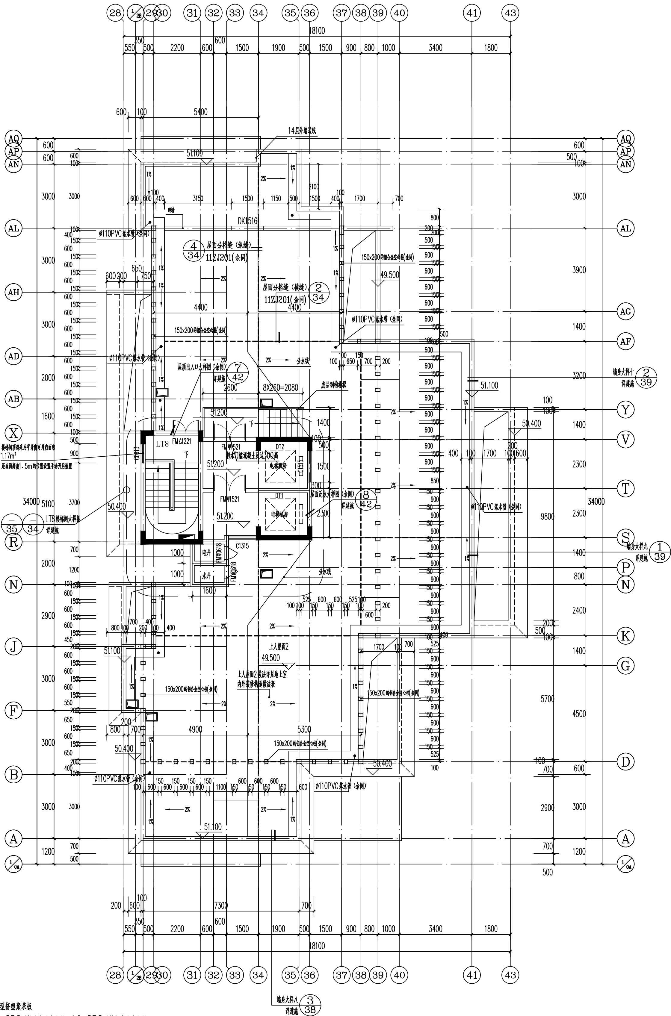
住宅屋顶平面图 1:100
