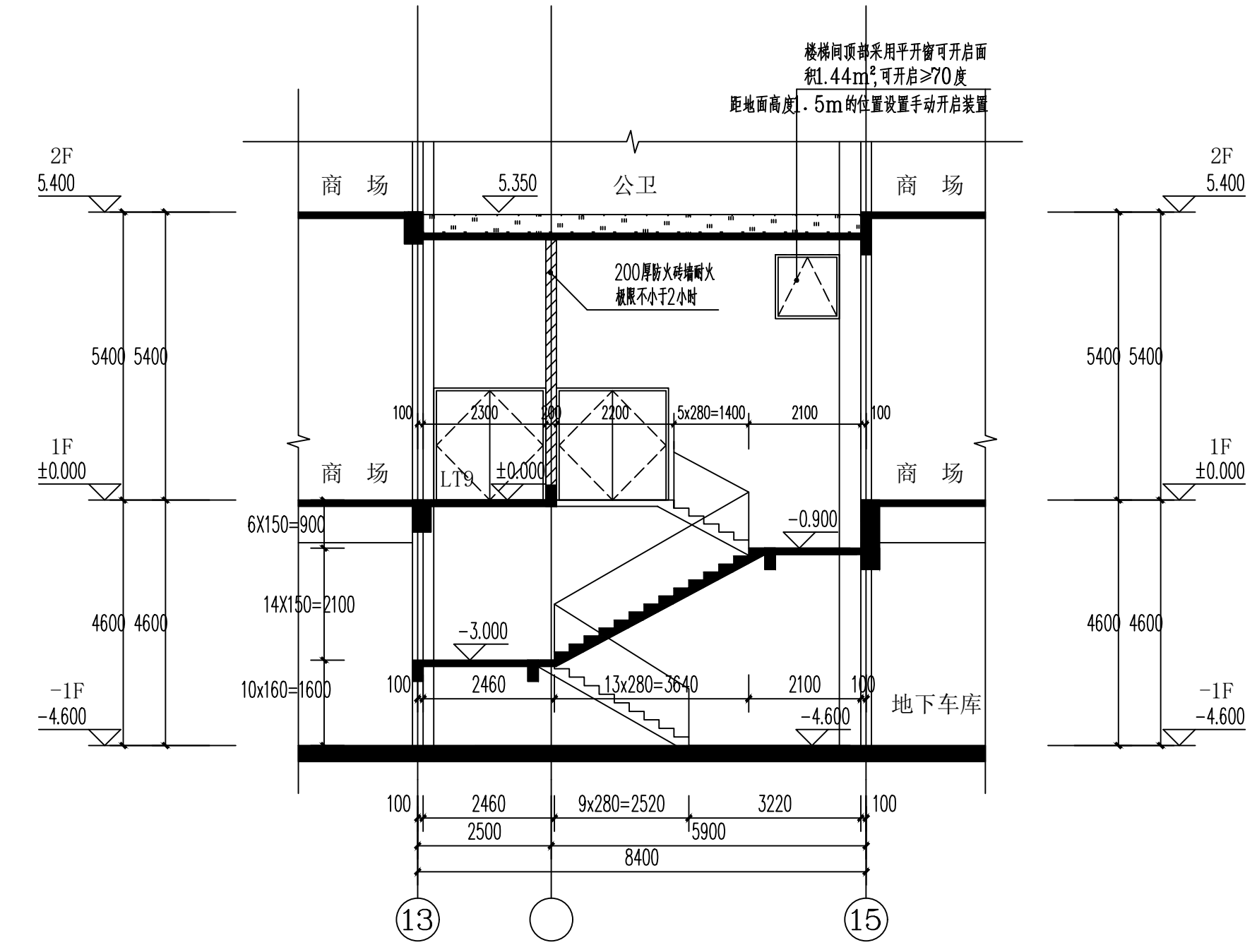
5-5剖面图 1:100
