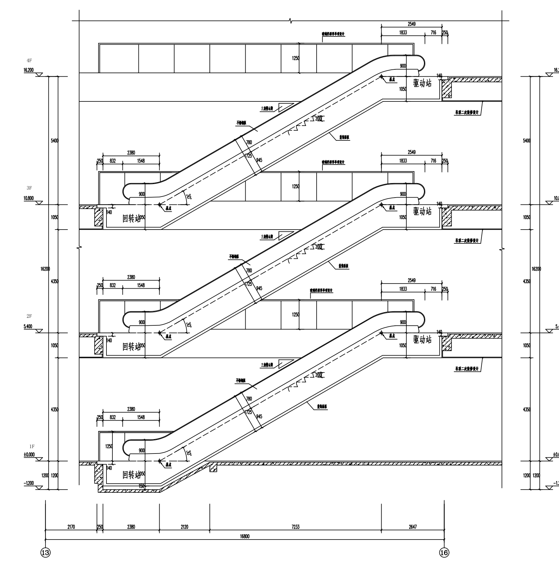
FT-01自动扶梯剖面图 1:50
