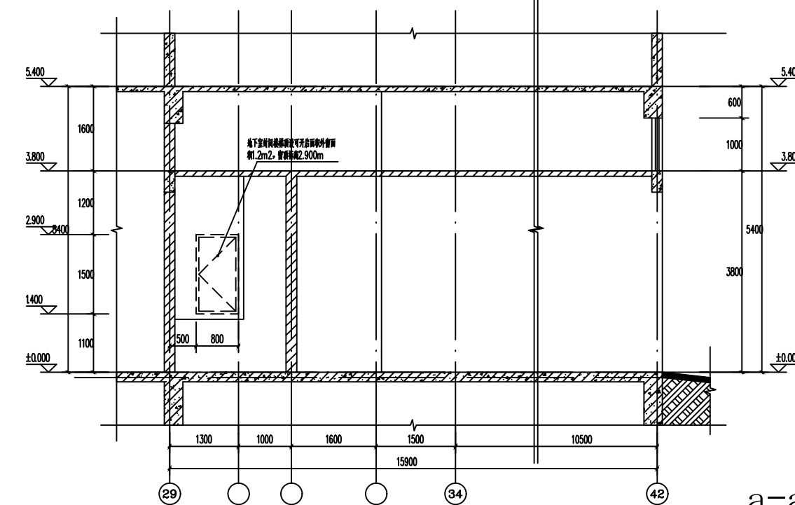
FT-03自动扶梯剖面图 1:5
