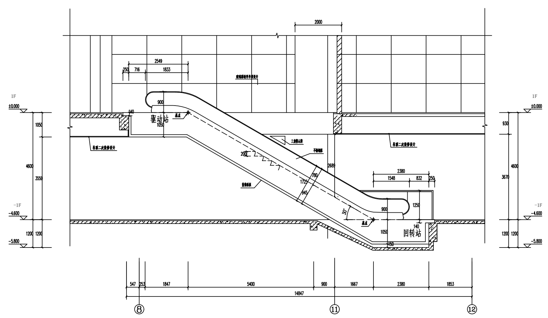
FT-03自动扶梯剖面图 1:5
