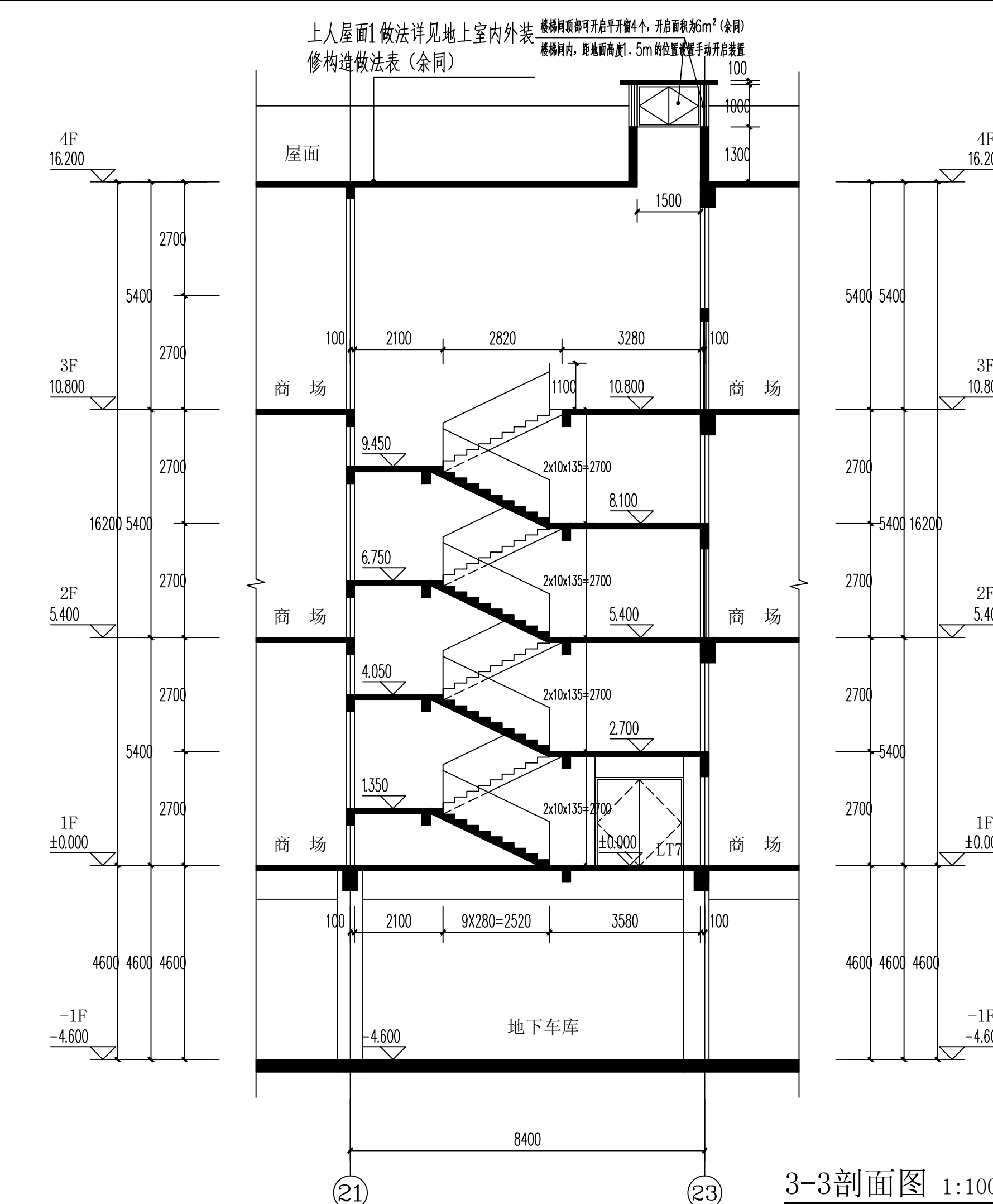
3-3剖面图 1:100
