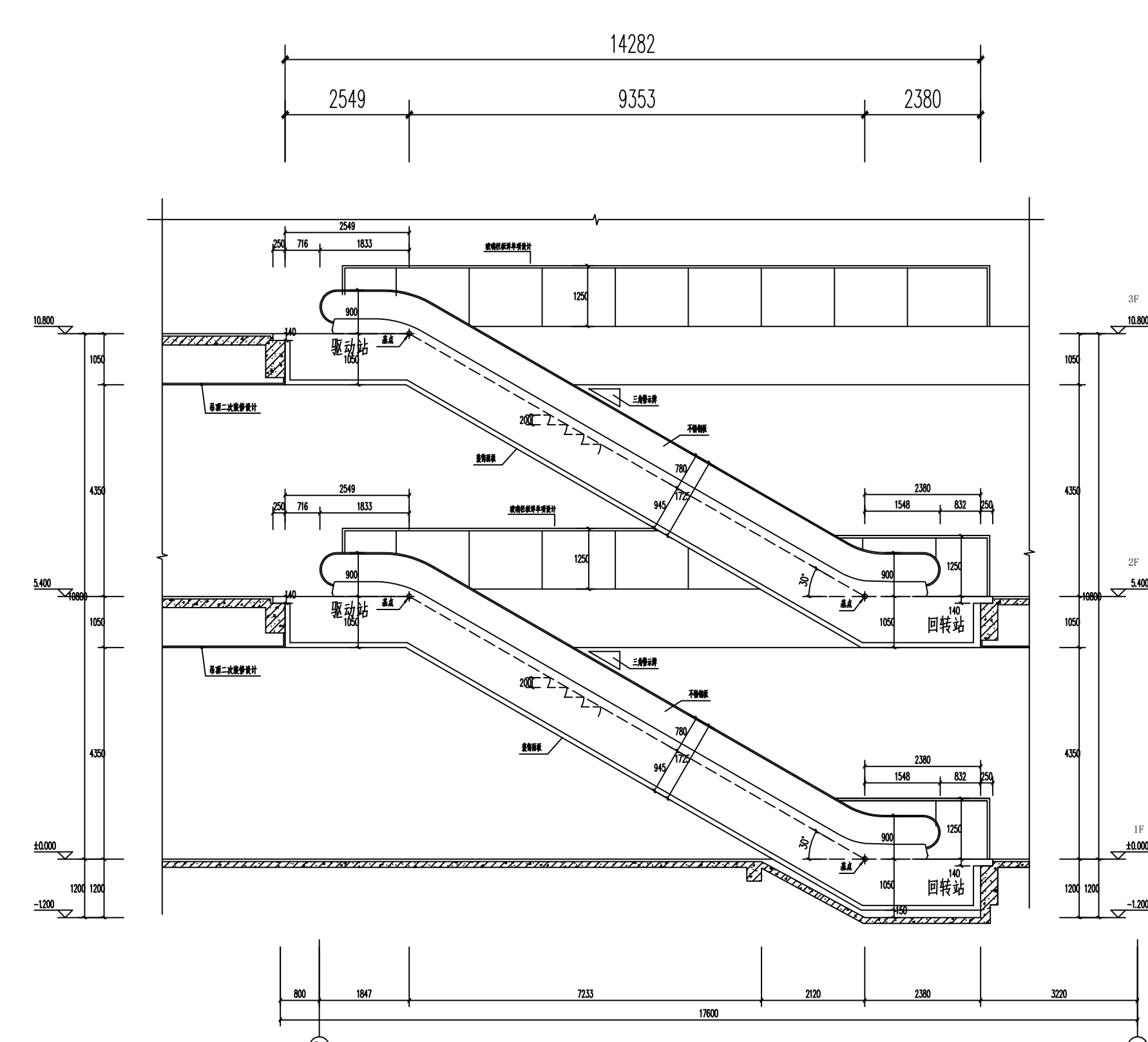
FT-02自动扶梯剖面图 1:5
