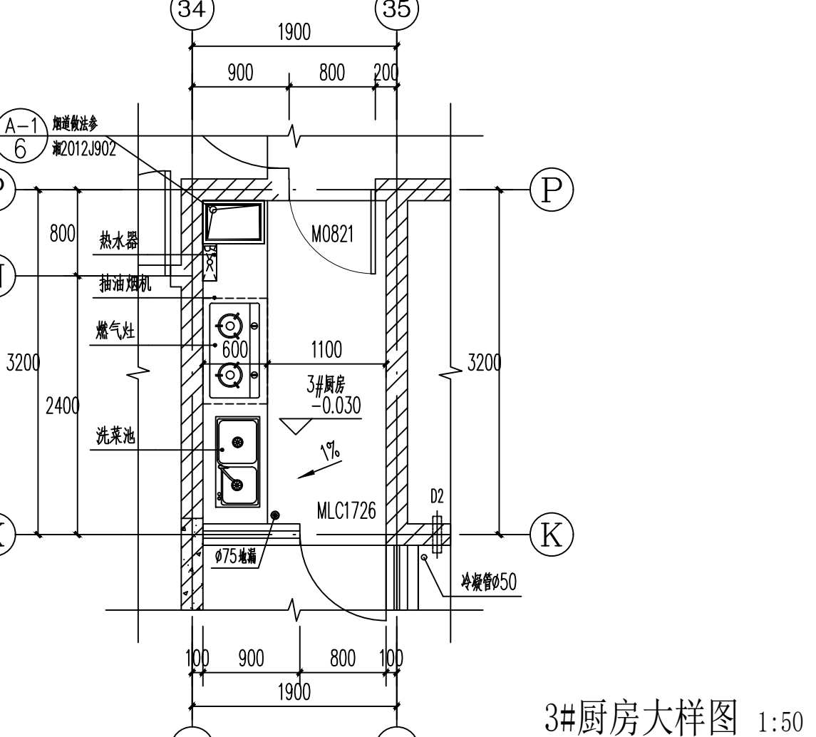
3#厨房大样图 1:50
