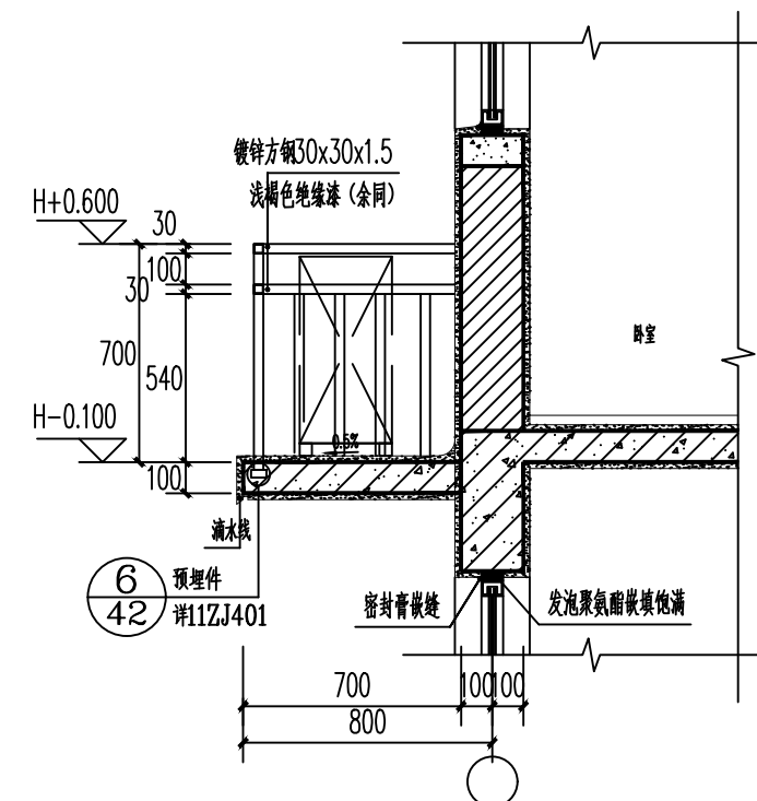
④ 空调板大样图 1:25
