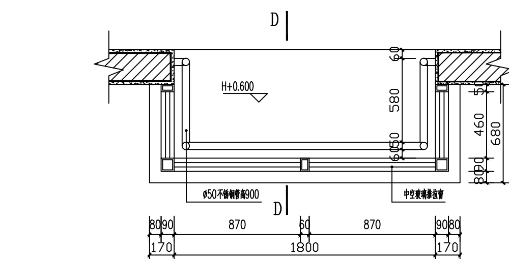
TC1平面图 1:20
