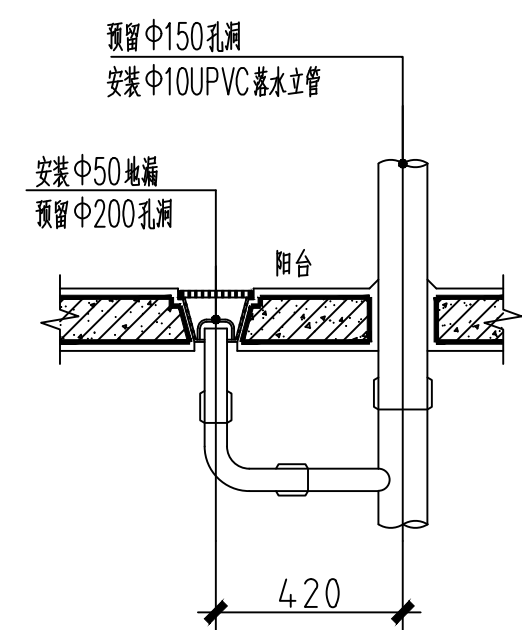
⑥单阳台排水大样图 1:25
