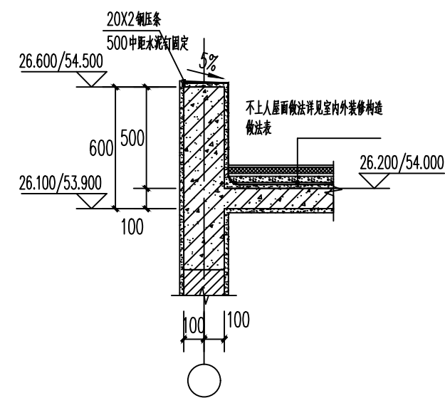
① 返边大样图 1:25
