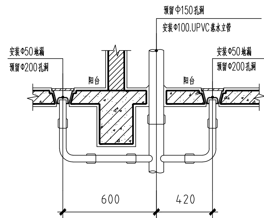
⑤ 双阳台排水大样图 1:25
