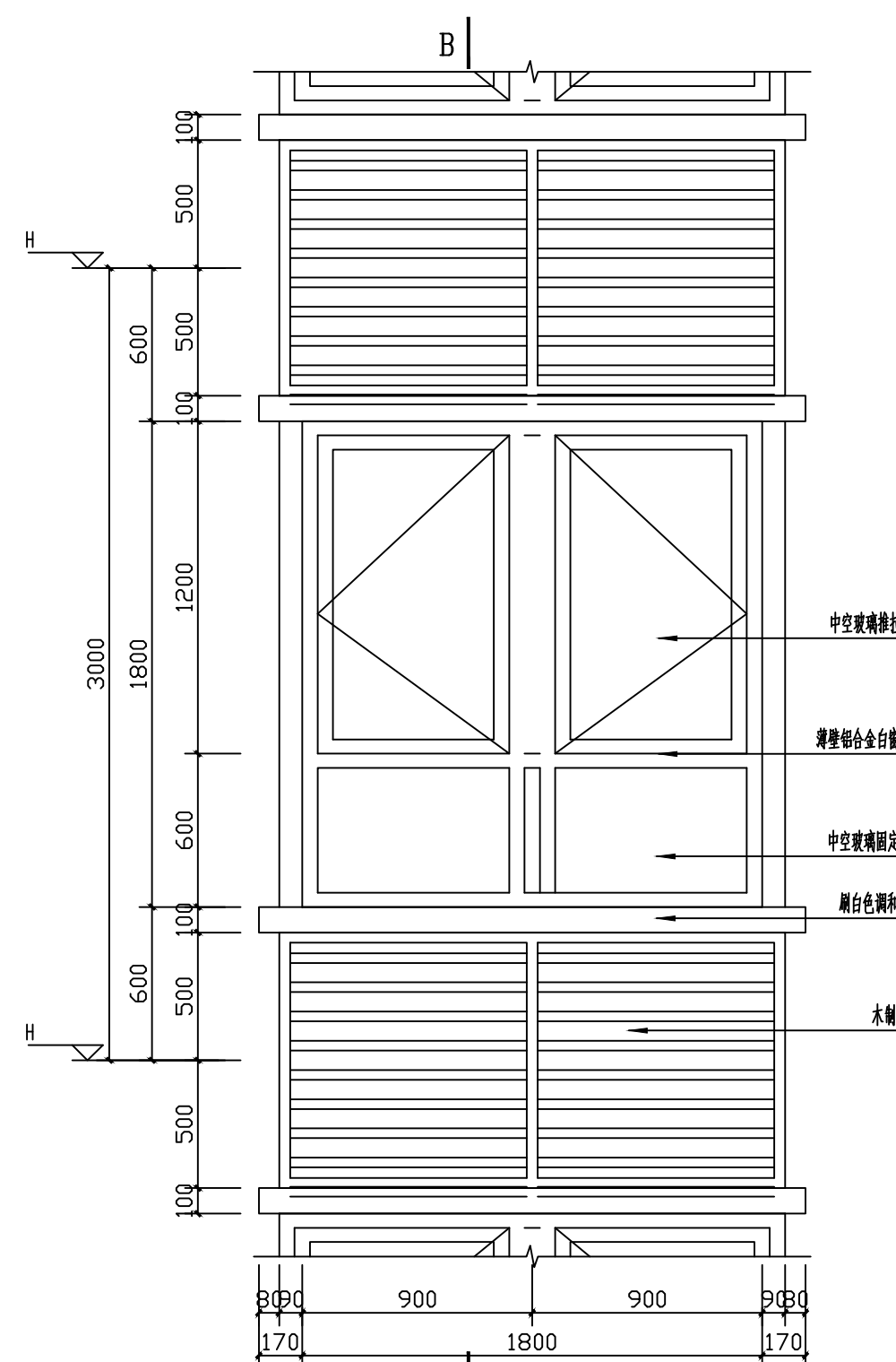
TC1立面 1:20
