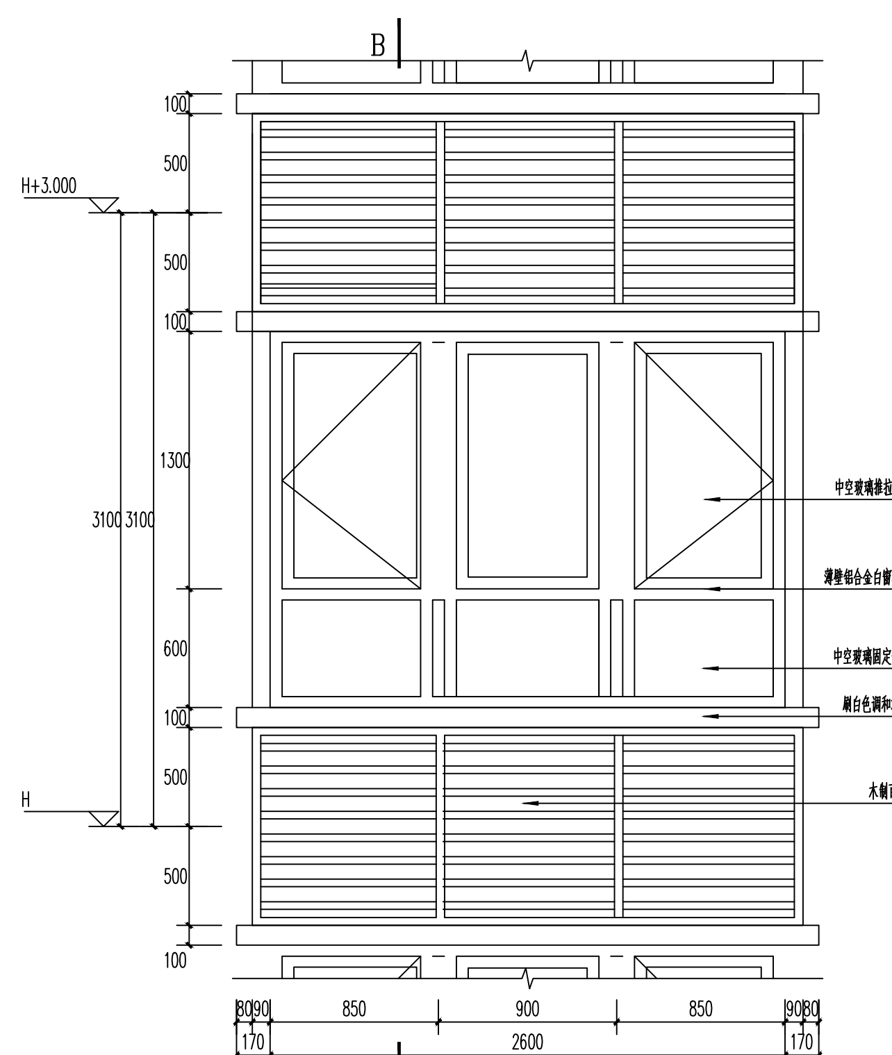
TC2立面 1:20
