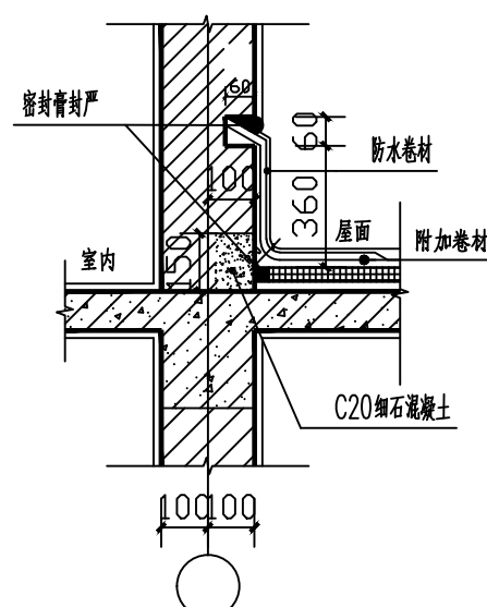
⑧ 屋面泛水大样图 1:25
