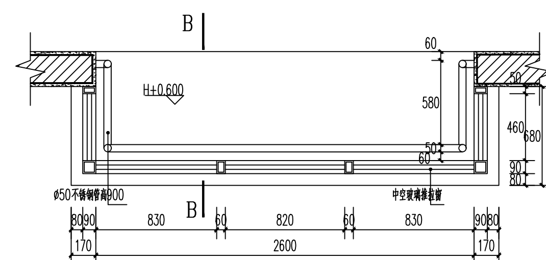
TC2平面图 1:20
