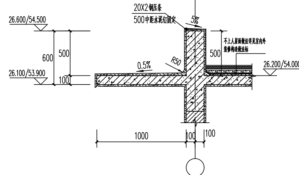
② 雨蓬大样图 1:25
