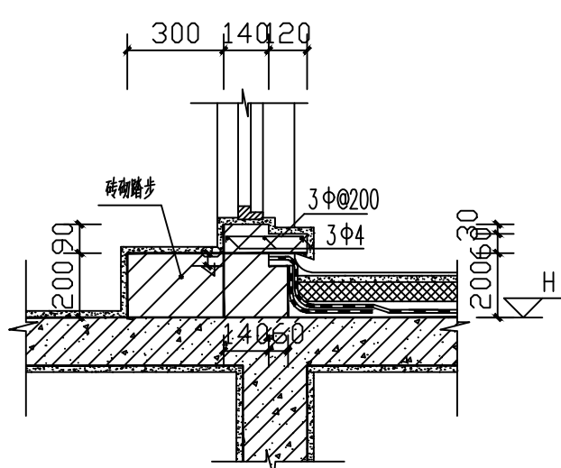
⑦ 屋顶出入口大样图 1:25
