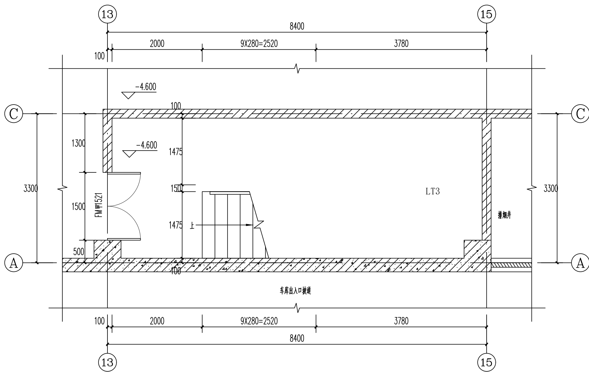
LT3楼梯间负一层平面图 1:50
