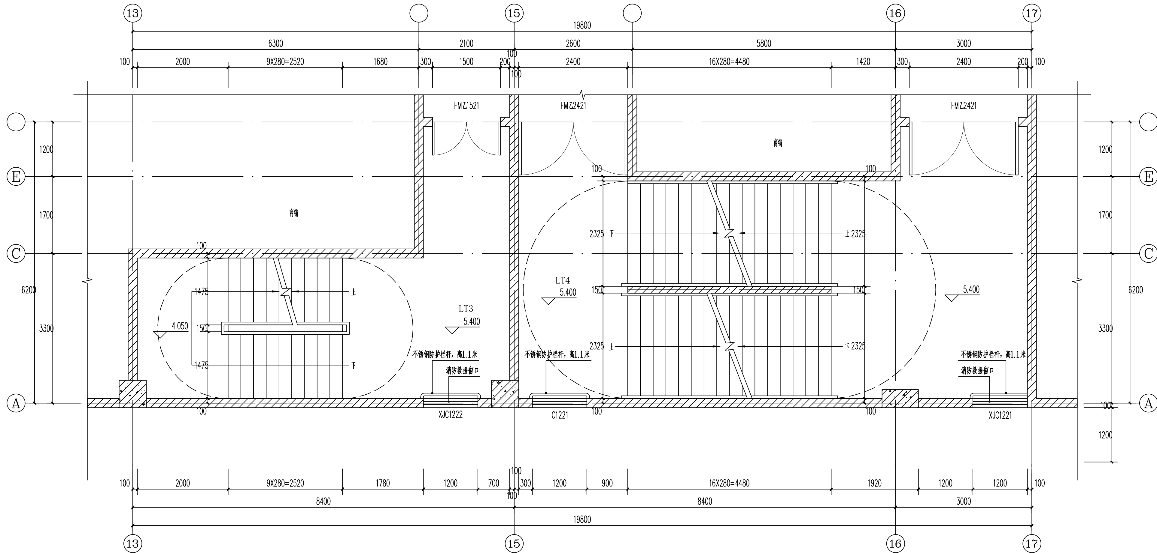
LT3、LT4楼梯间二层平面图 1:50
