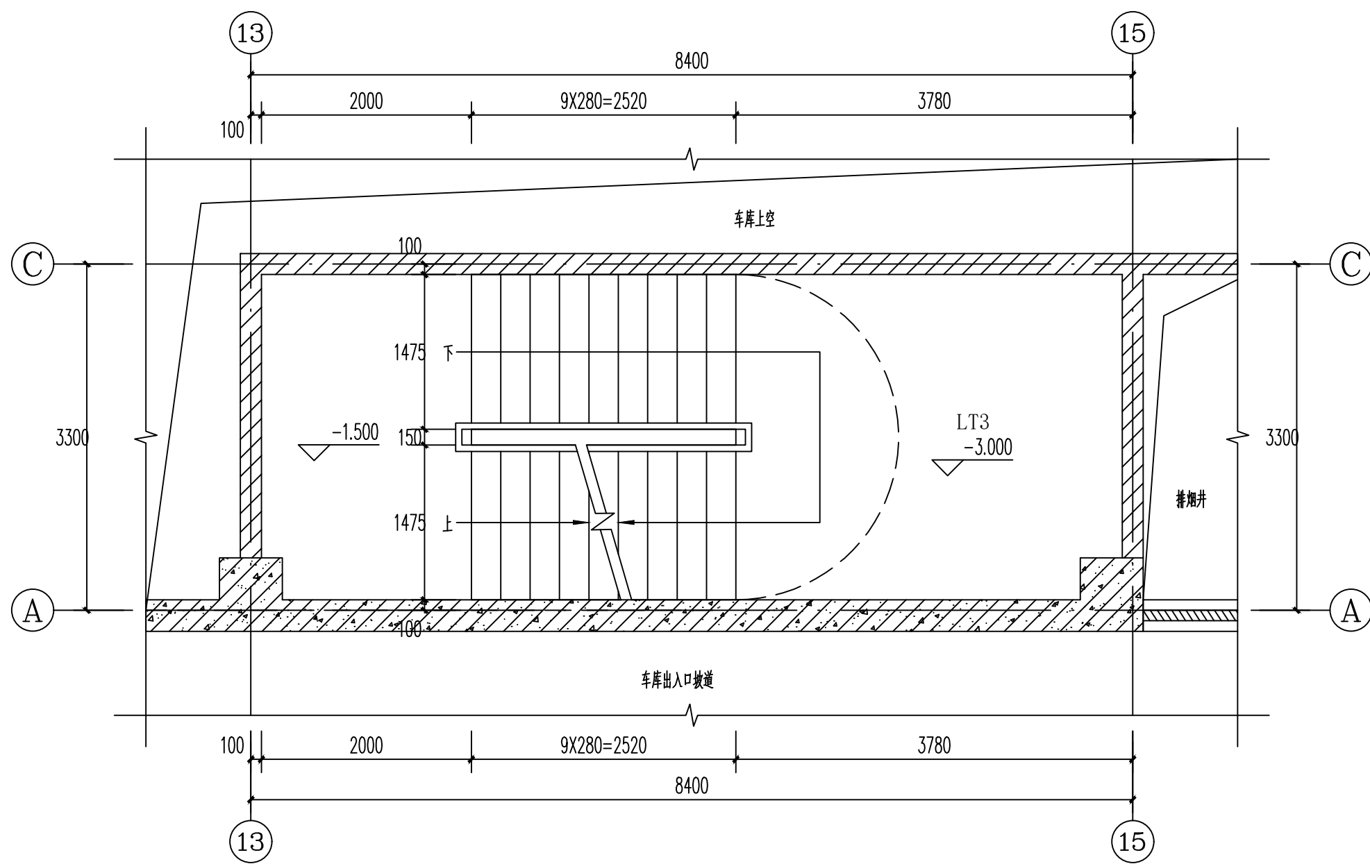
LT3楼梯间H=-3.00处平面图 1:50
