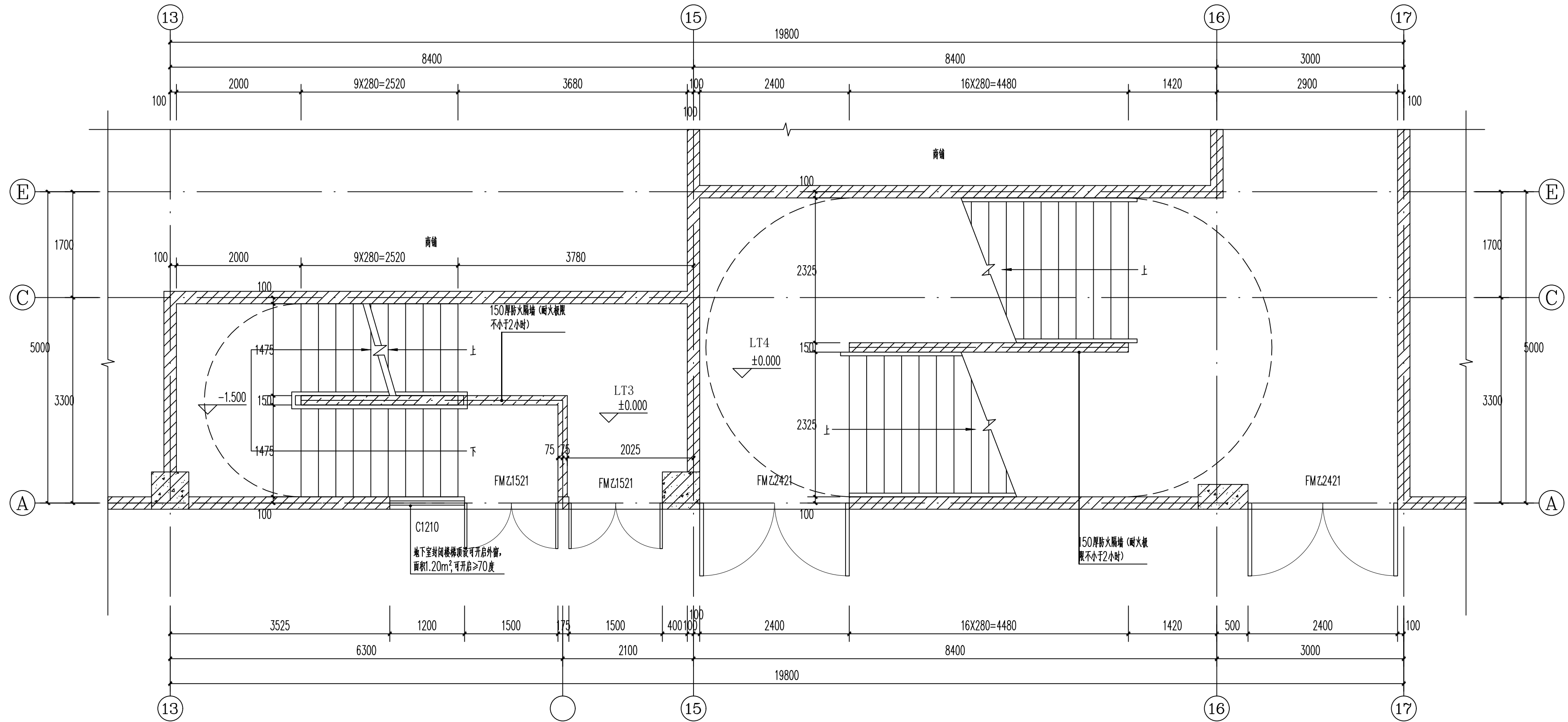
LT3、LT4楼梯间一层平面图 1:50
