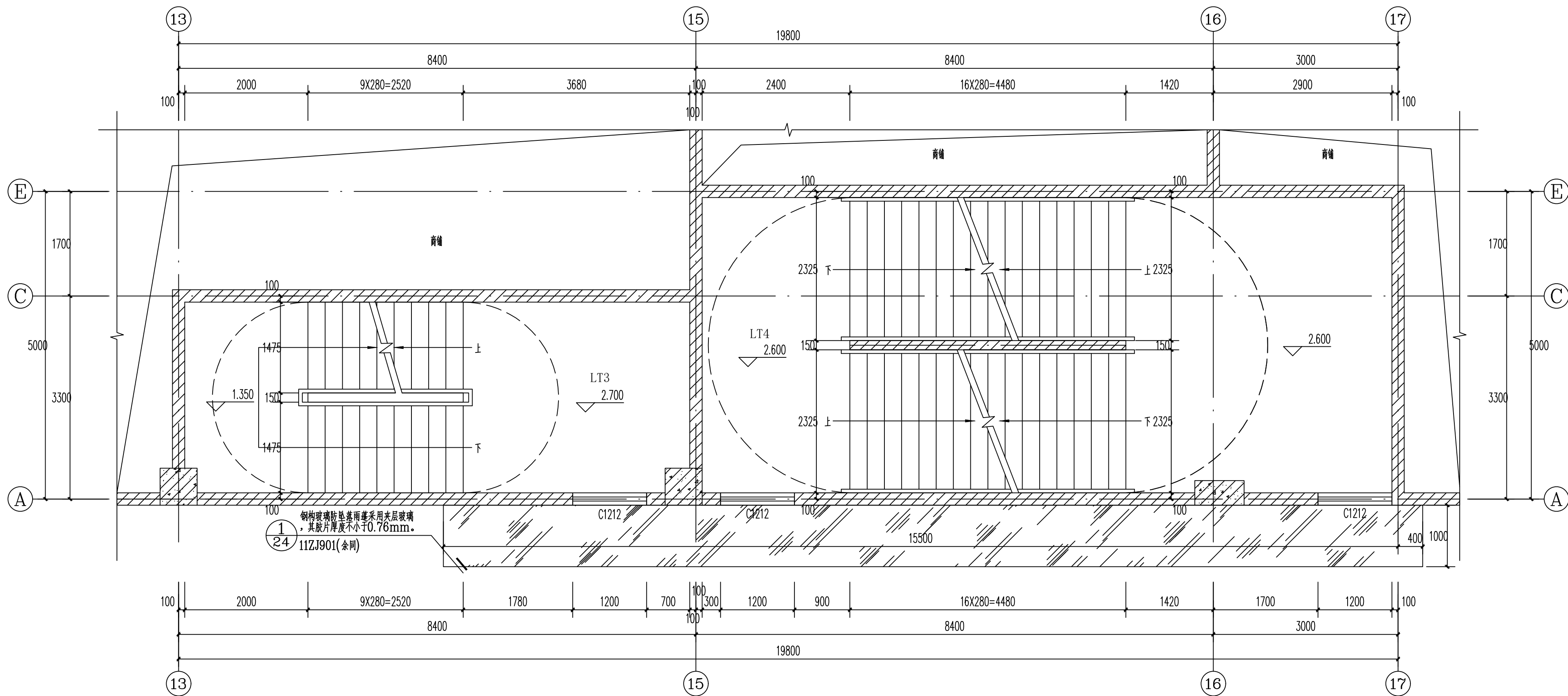
LT3、LT4楼梯间H=2.700处平面图 1:50
