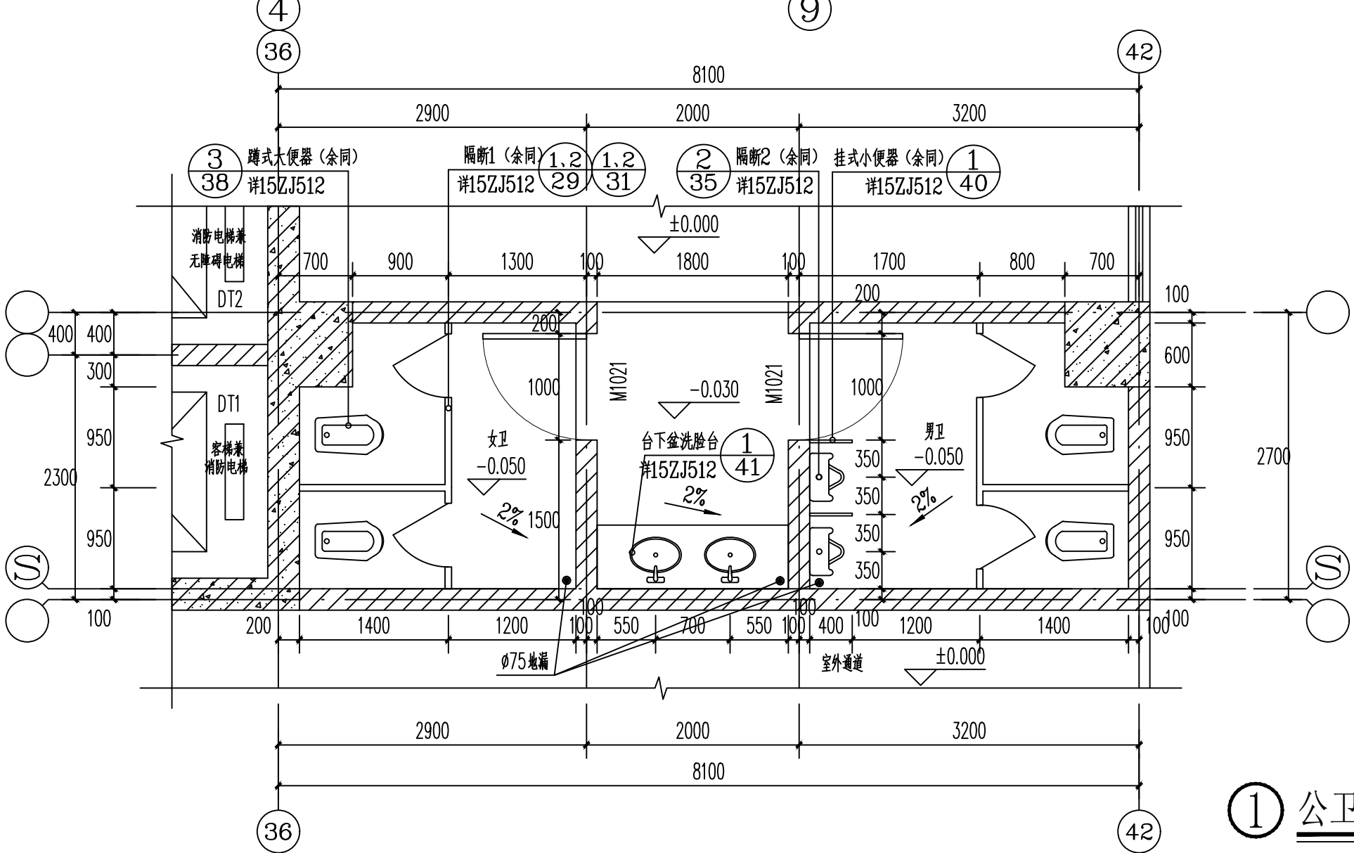
① 公卫一大样图 1:50
