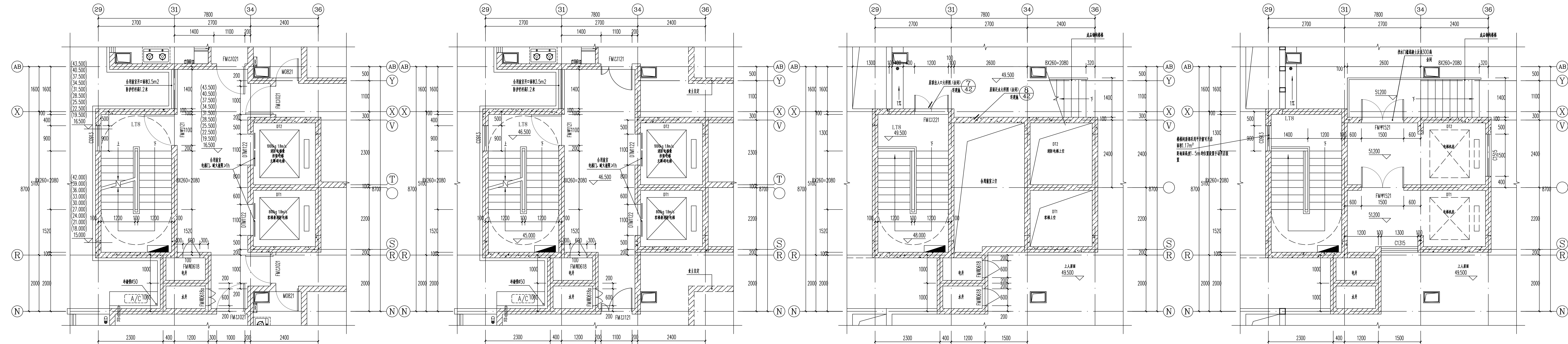
L78楼梯间四至十三层平面图 1:50
