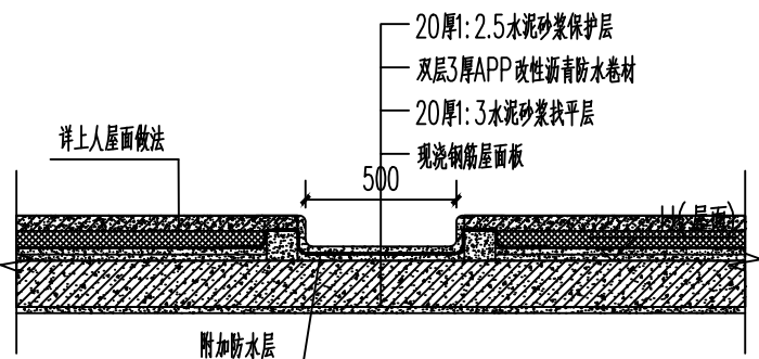
④ 屋面内天沟大样 1:50
