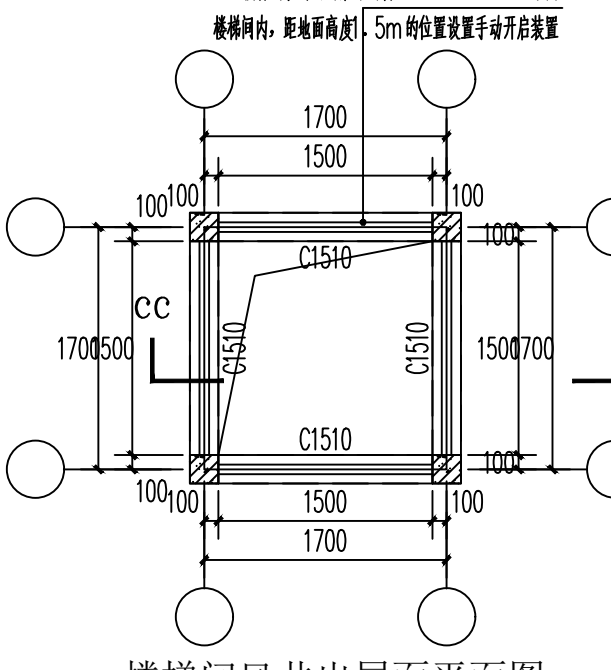
⑧ 楼梯间风井出屋面大样图 1:50
