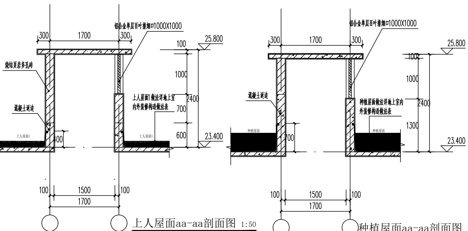
⑥ 排烟井出屋面大样图 1:50
