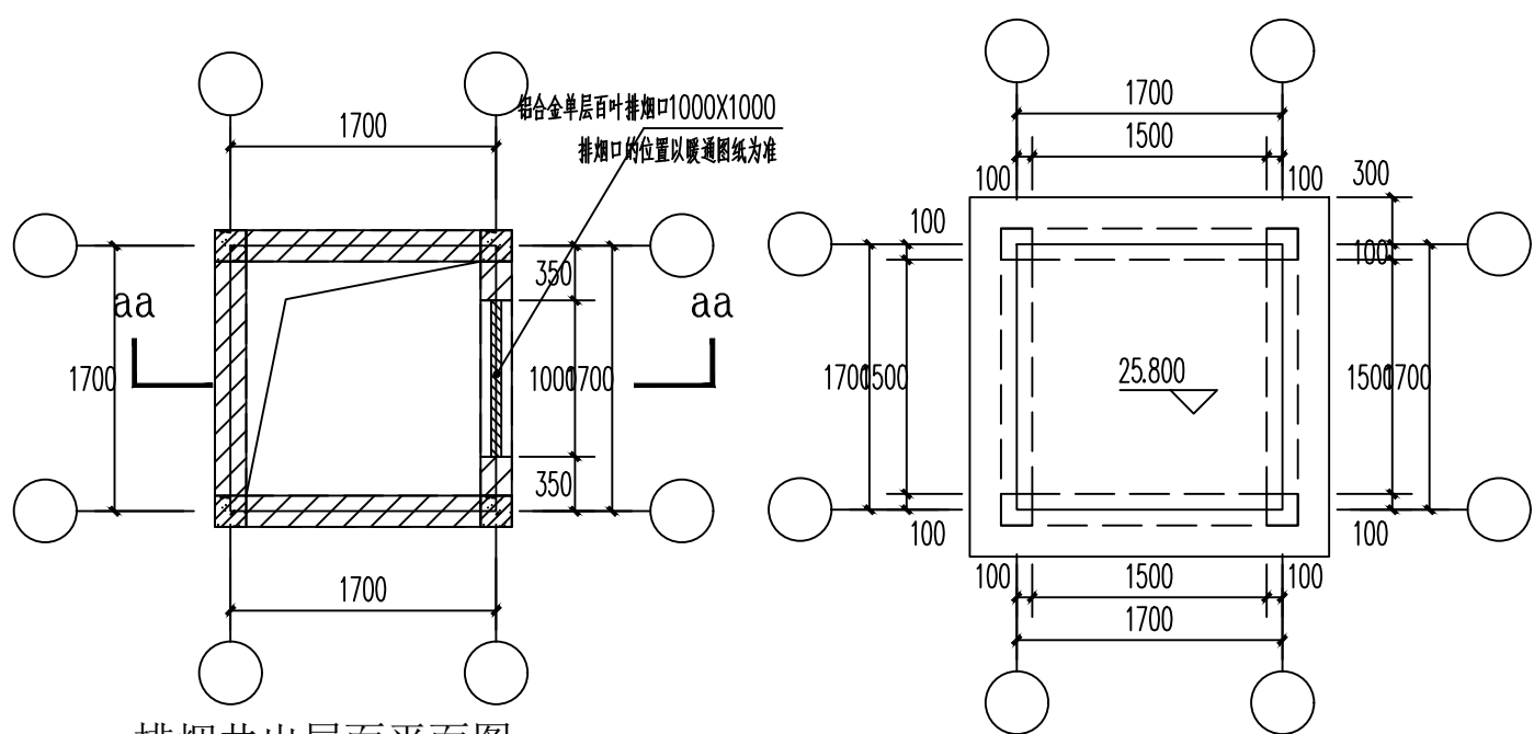
⑥ 排烟井出屋面大样图 1:50
