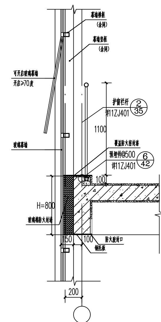
③ 幕墙防火封堵节点大样 1:50
