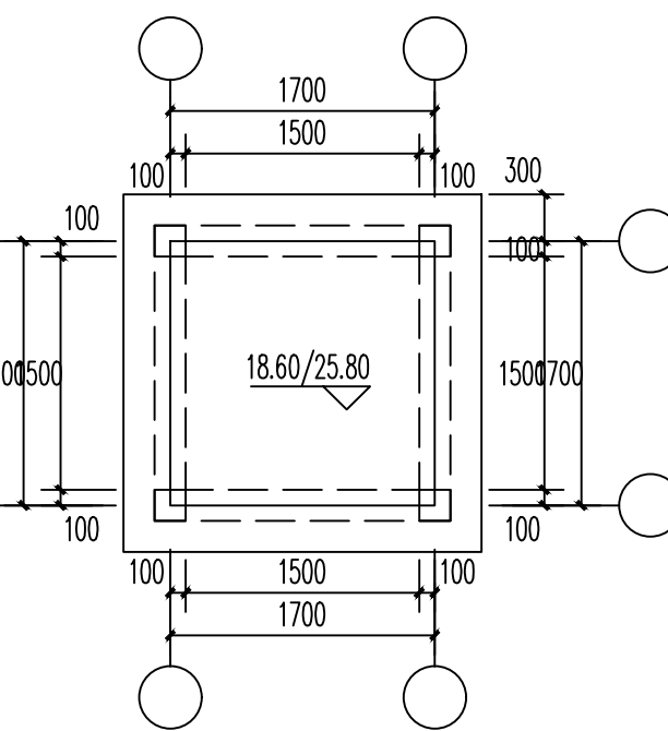
楼梯间风井出屋面部平面图 1:50
