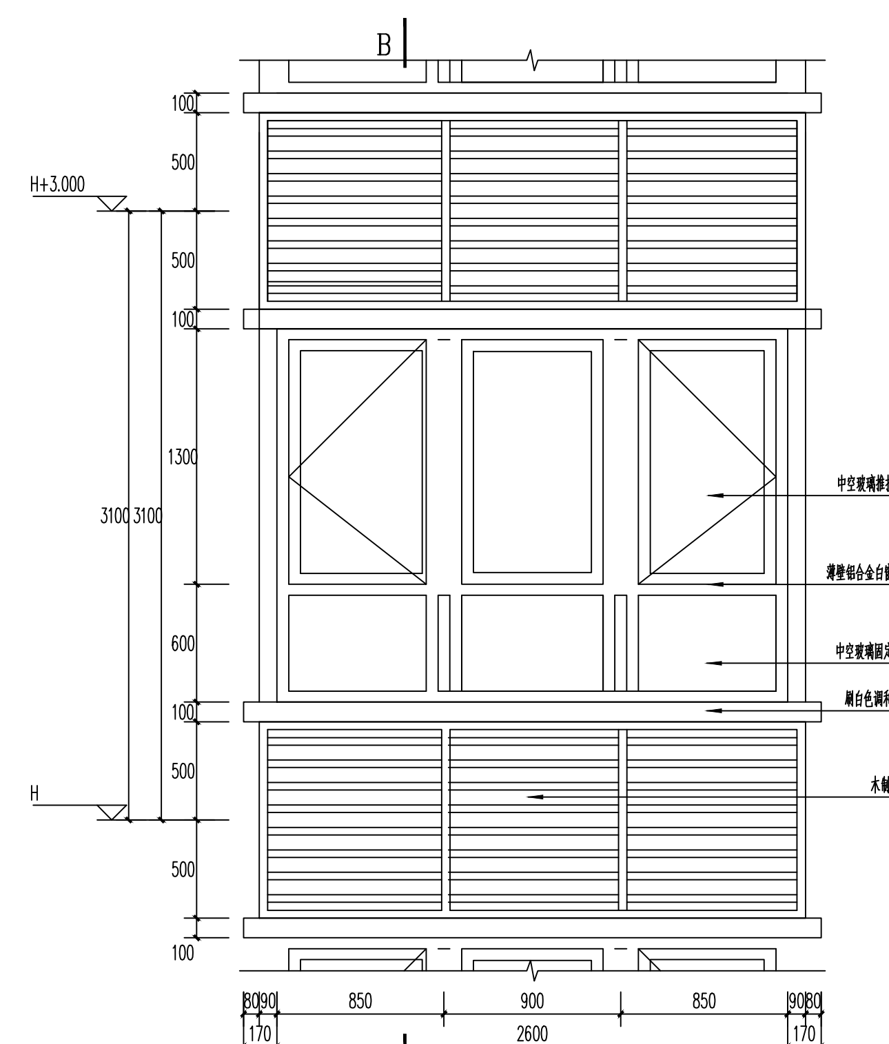
TC2立面 1:20
