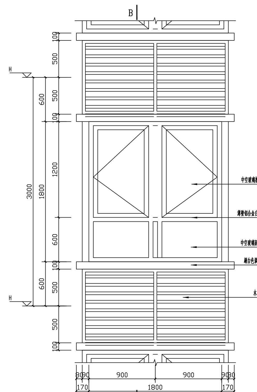
TC1立面 1:20
