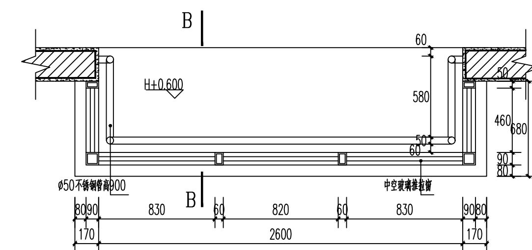
TC2平面图 1:20
