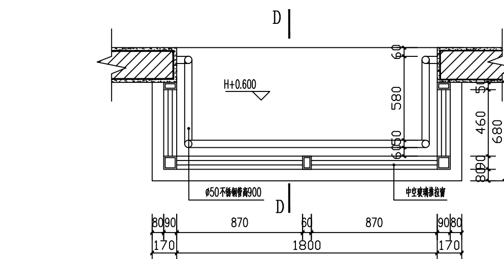
TC1平面图 1:20
