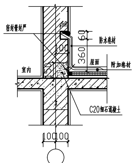
⑧ 屋面泛水大样图 1:25
