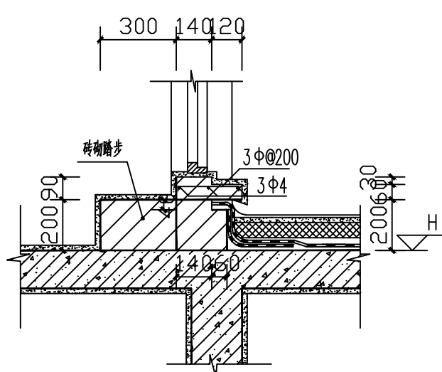
⑦ 屋顶出入口大样图 1:25
