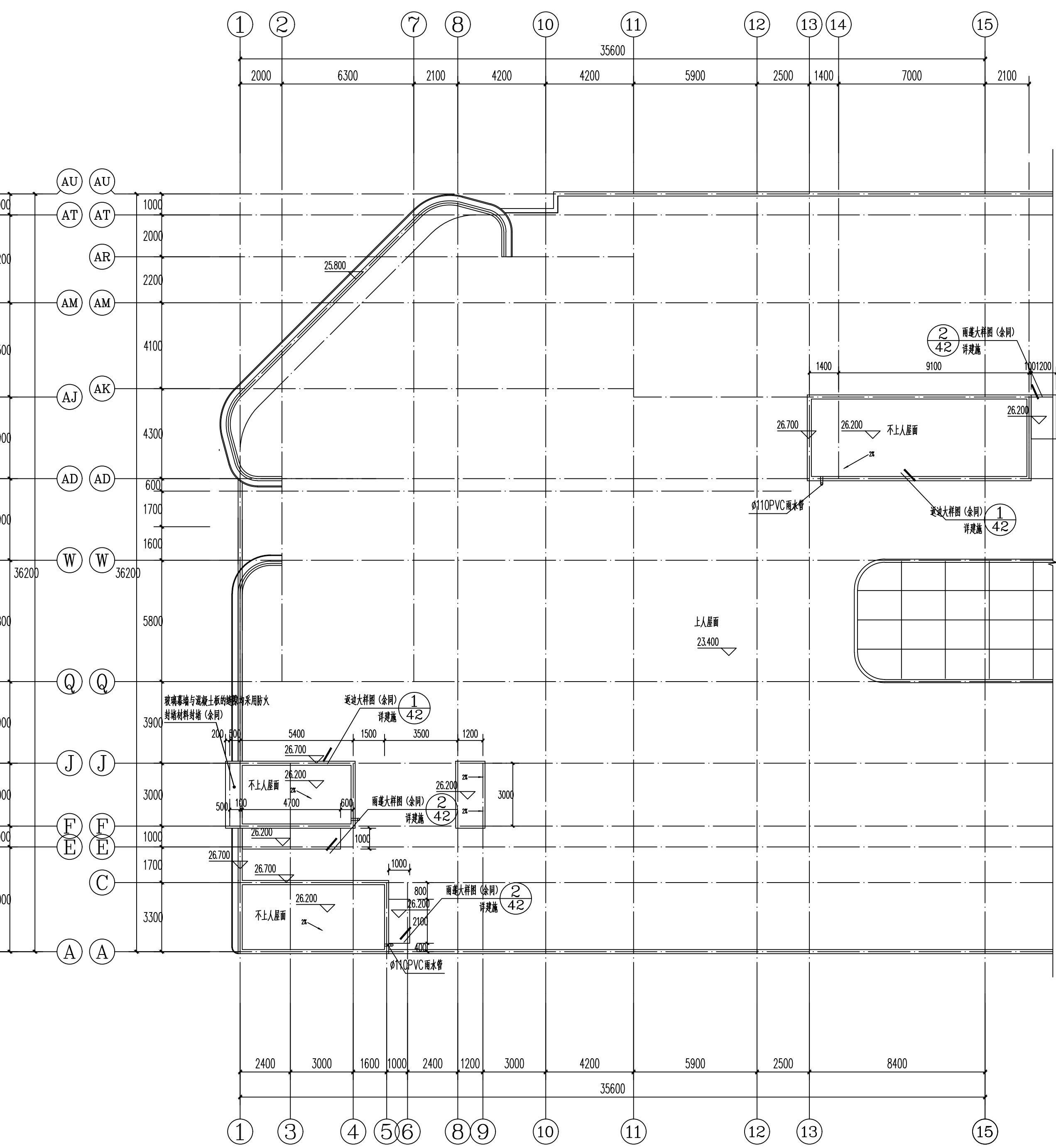
商业屋顶构件平面图 1:100
