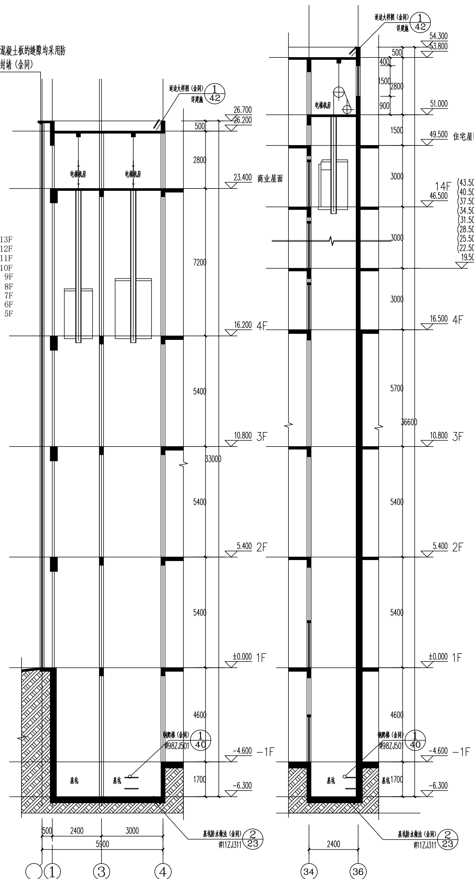
A-A断面图 1:100
