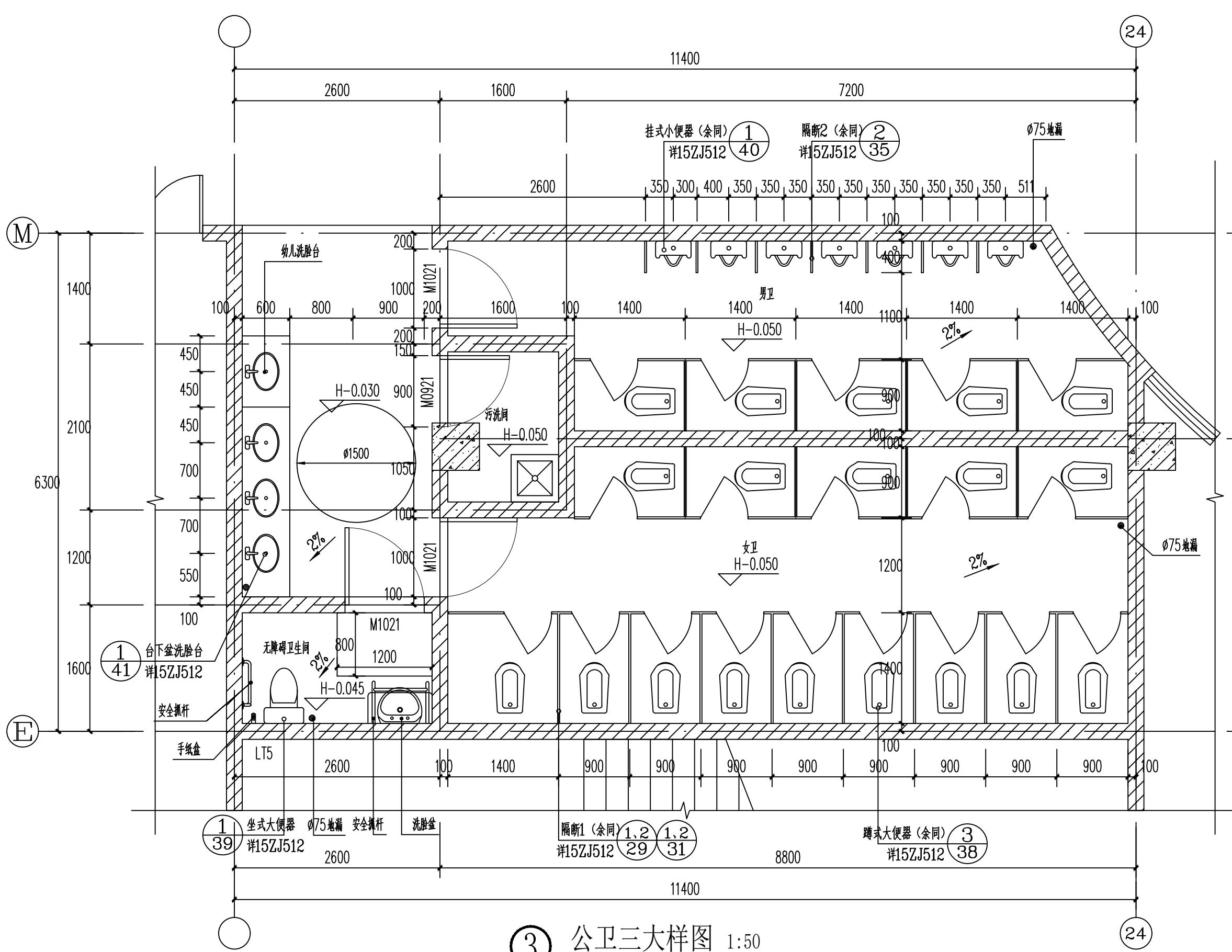
③ 公卫三大样图 1:50
