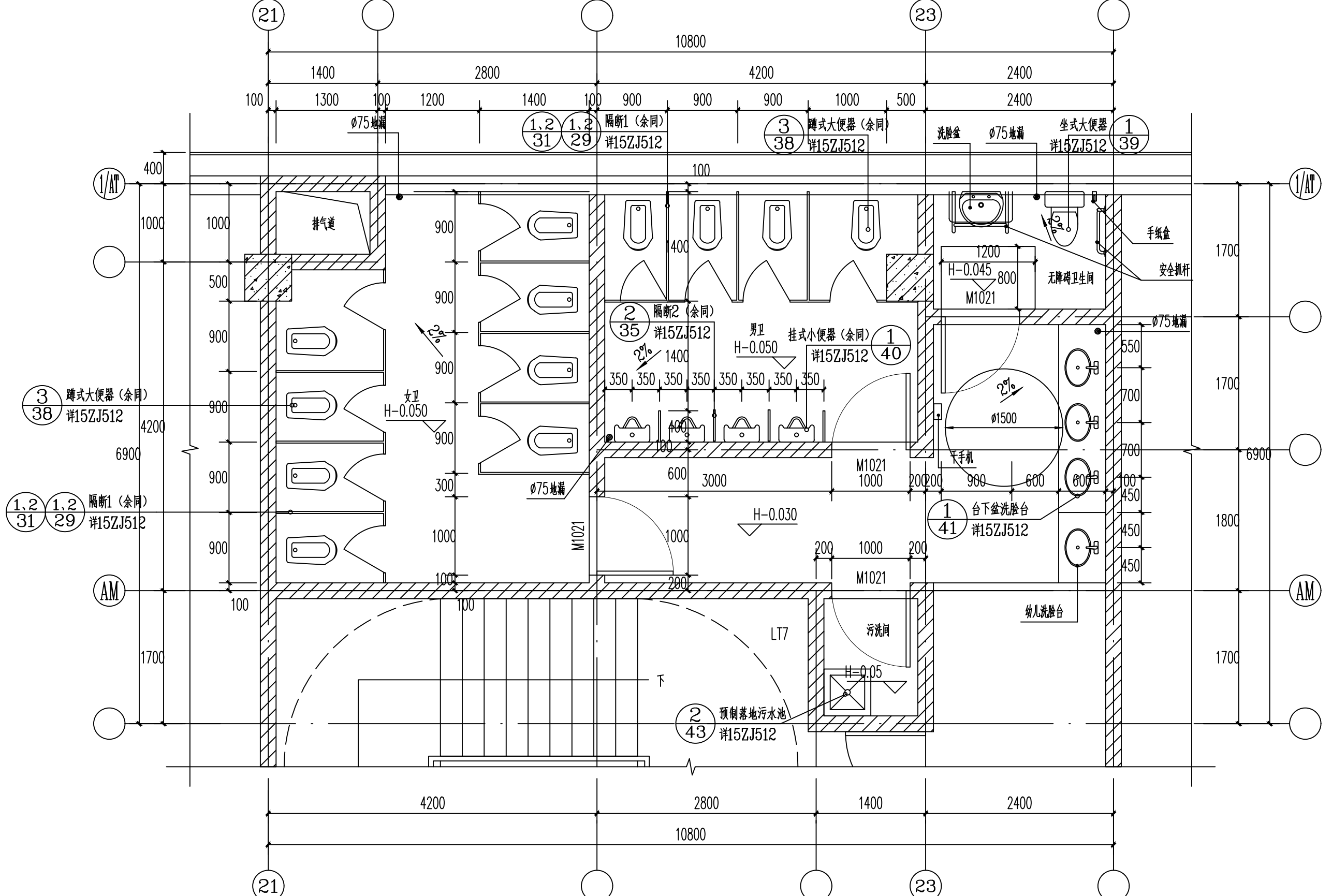
⑤ 公卫五大样图 1:50
