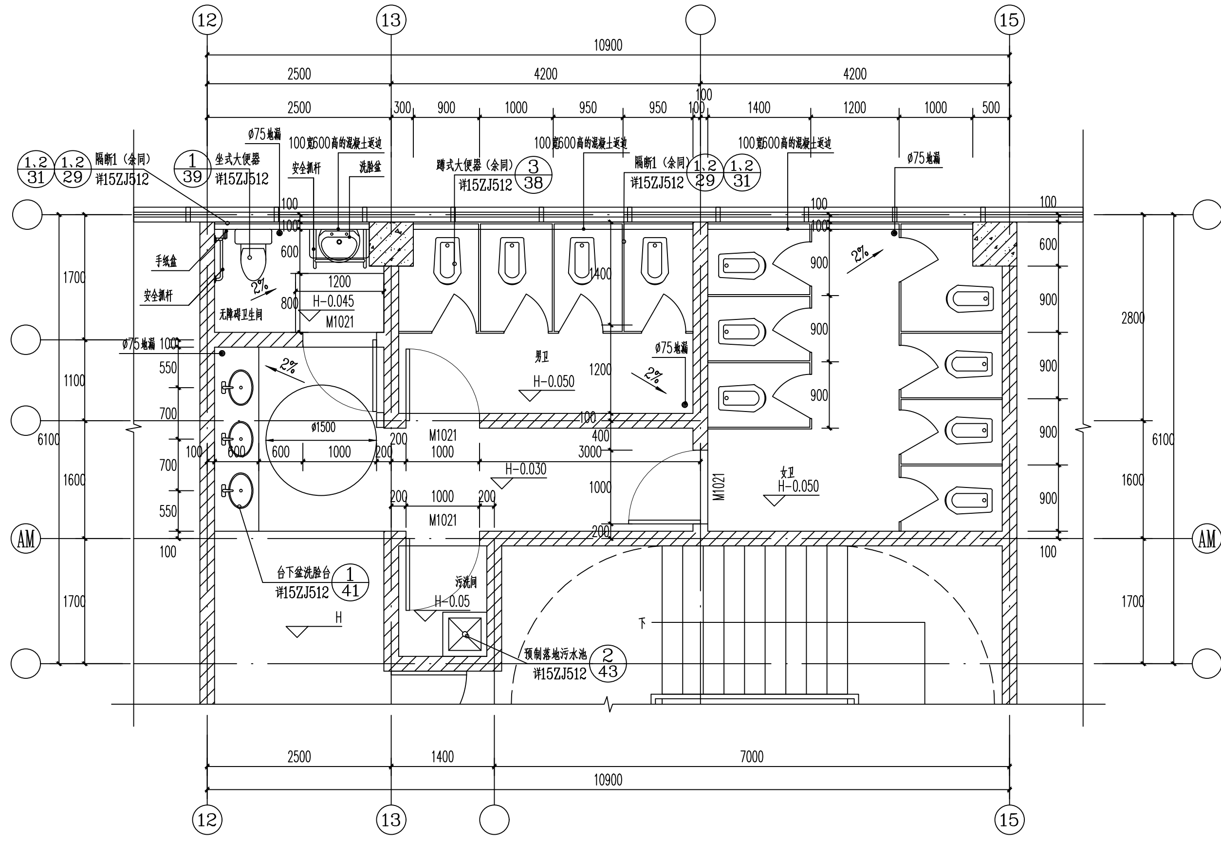
④ 公卫四大样图 1:50
