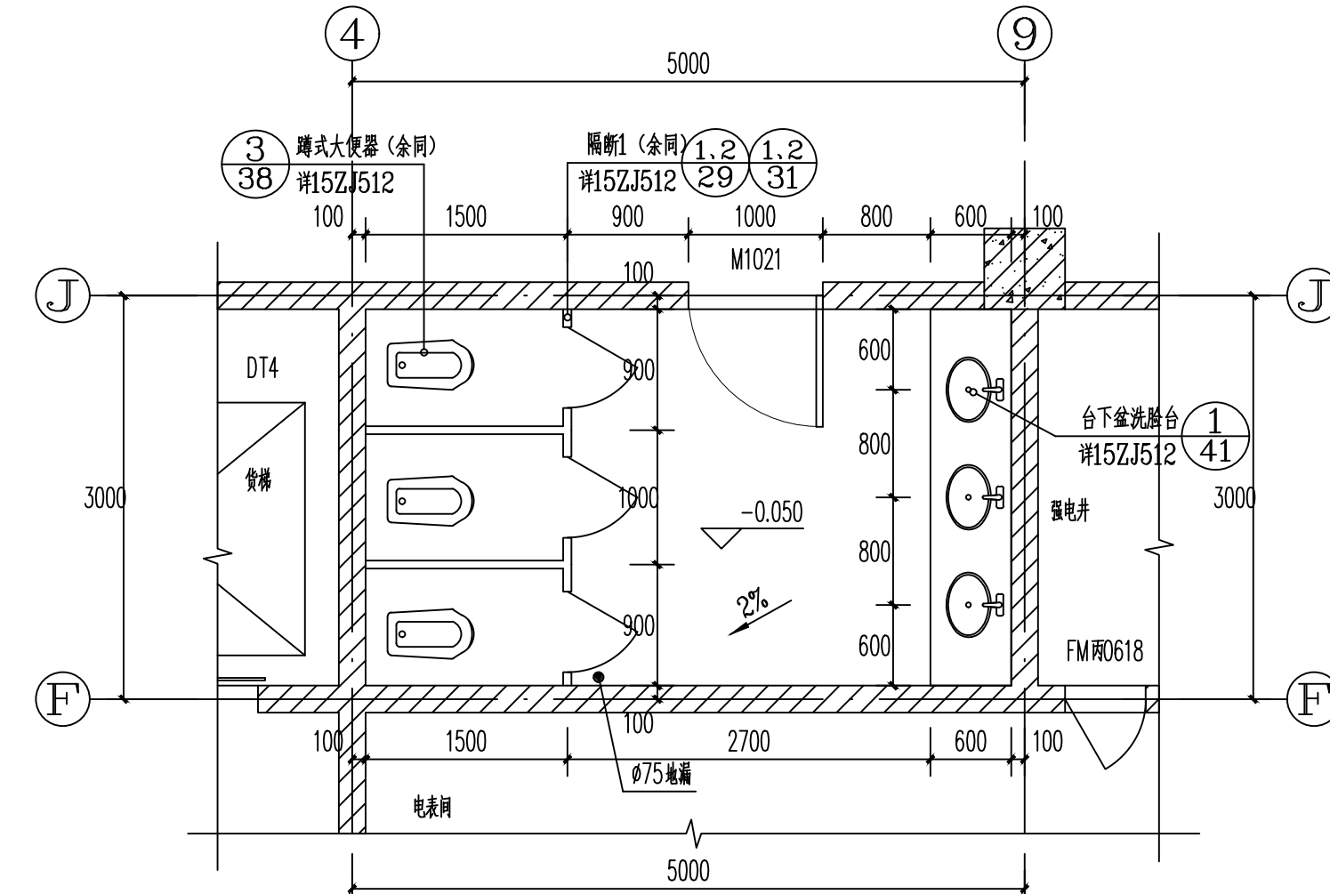
① 公卫一大样图 1:50
