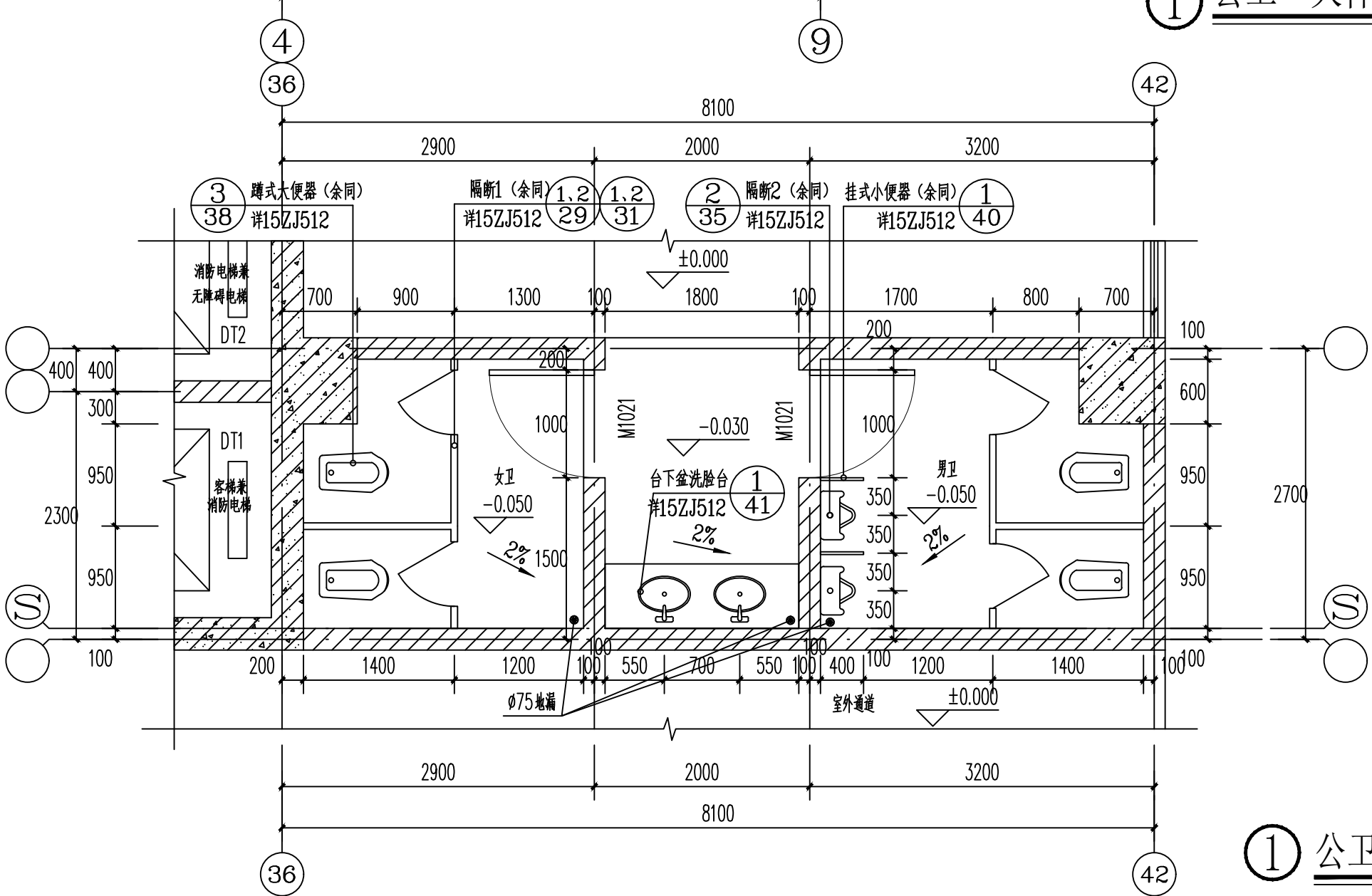
① 公卫一大样图 1:50
