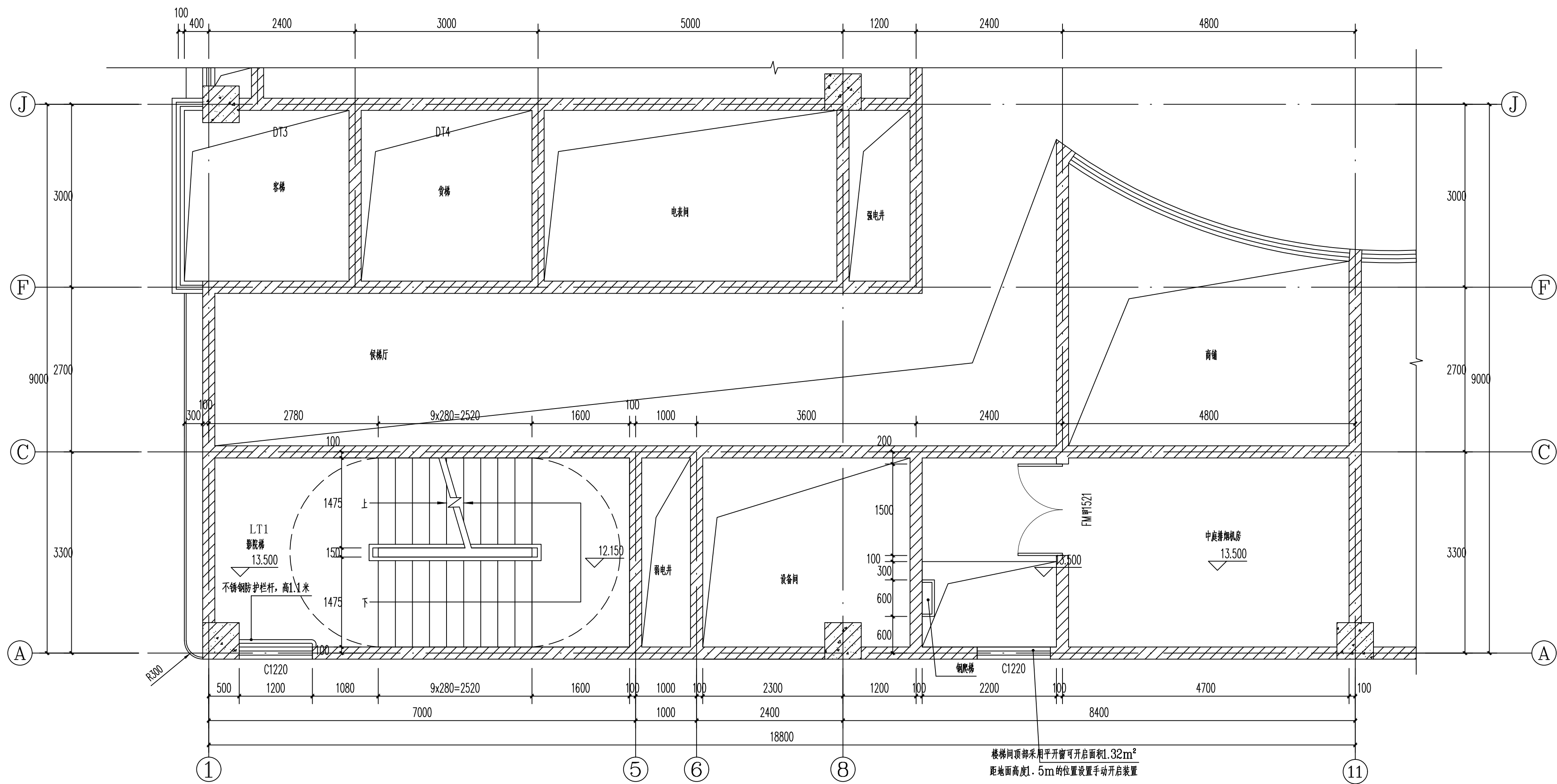
LT1、LT2楼梯间H=13.500处平面图 1:50
