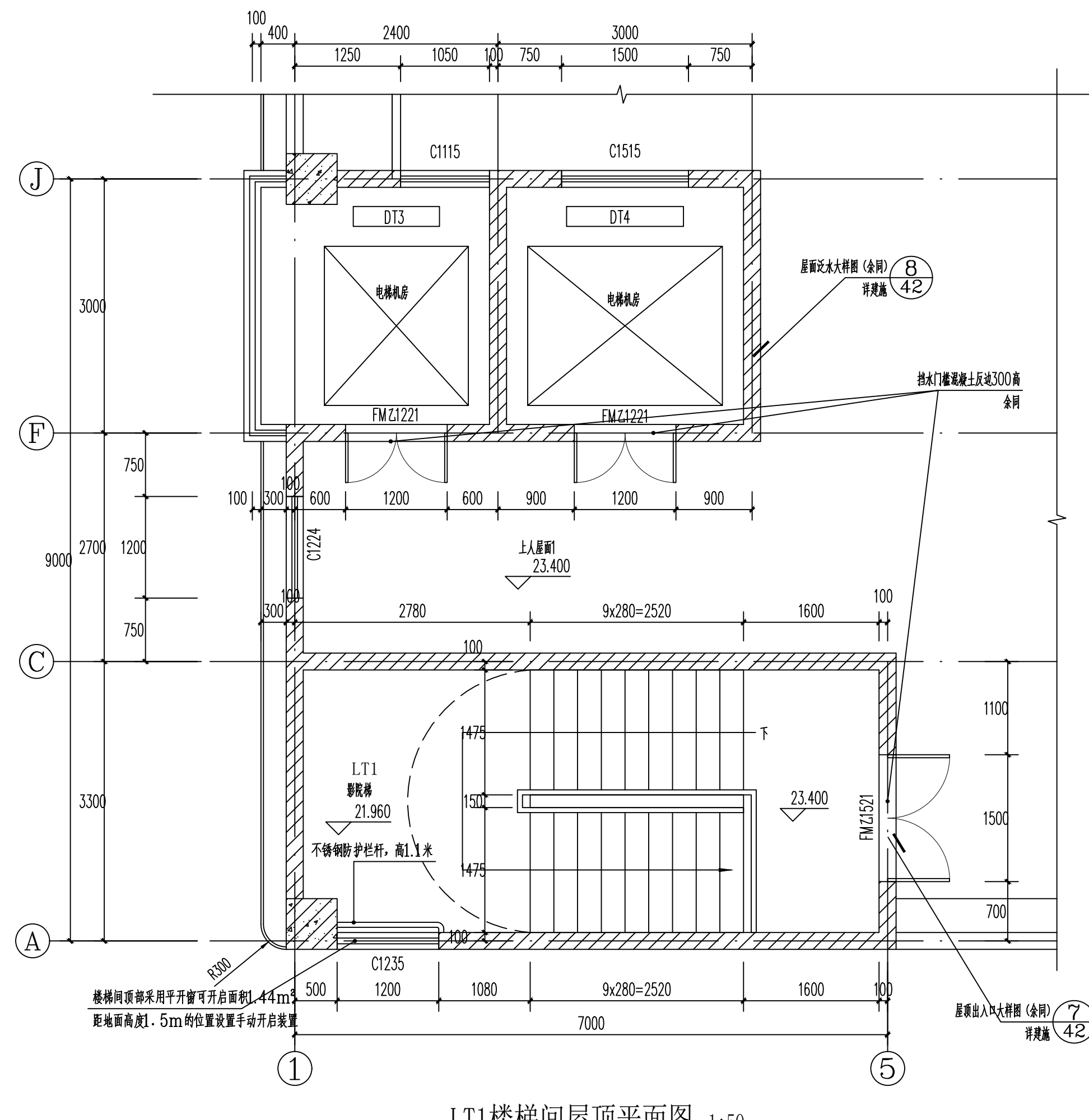
LT1楼梯间屋顶平面图 1:50
