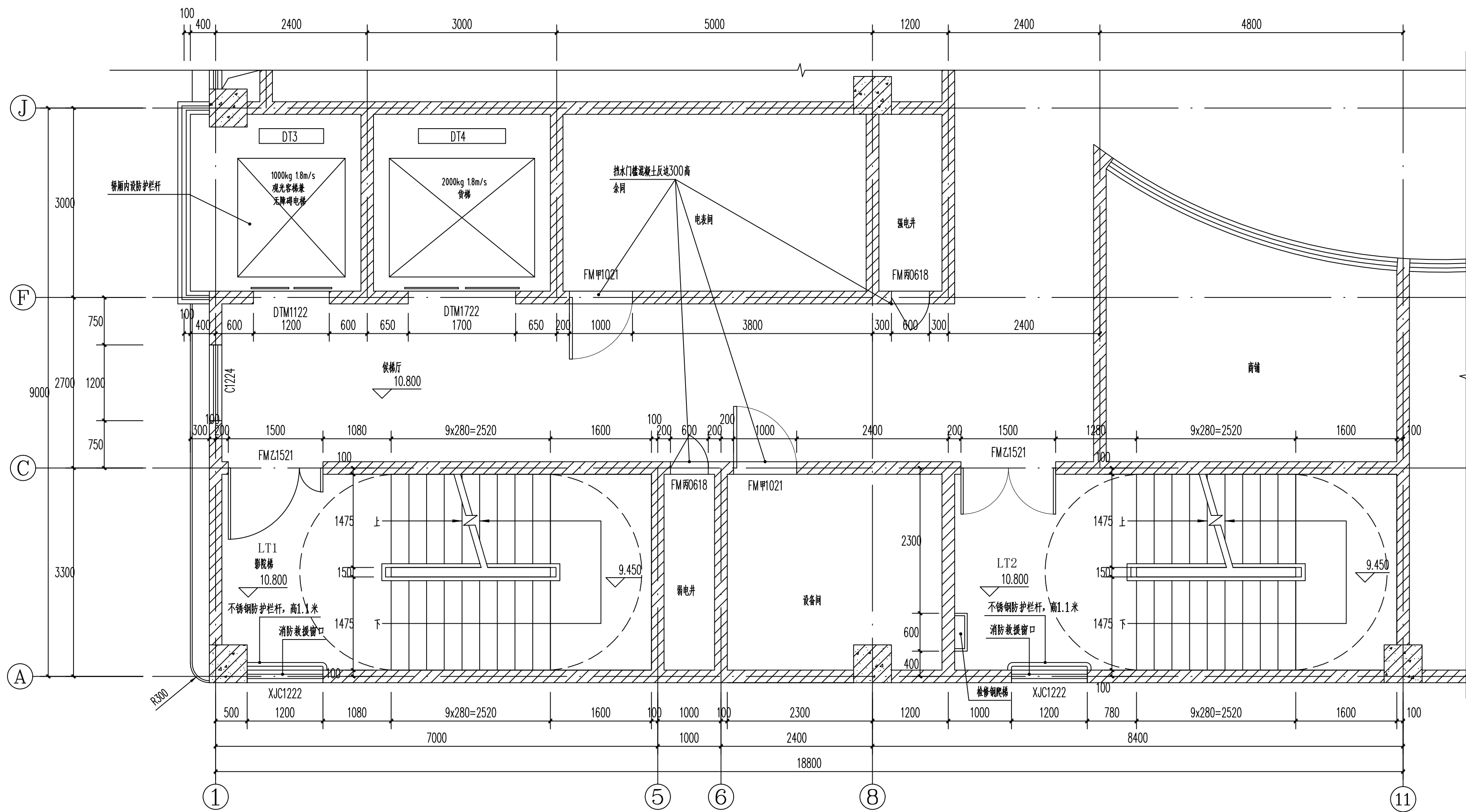
LT1、LT2楼梯间三层平面图 1:50
