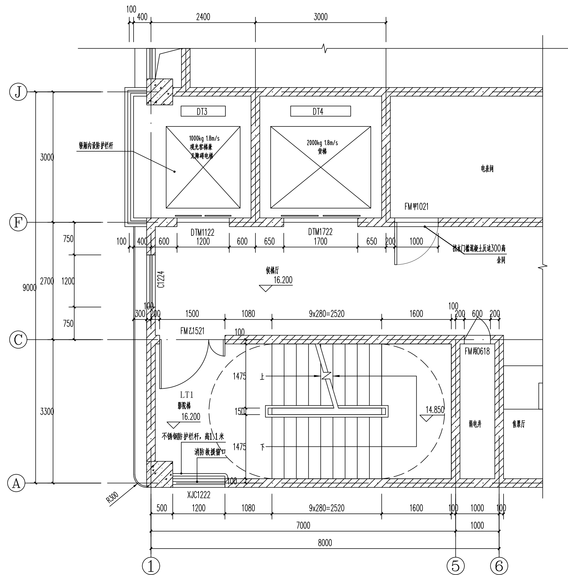
LT1、LT2楼梯间三层平面图 1:50
