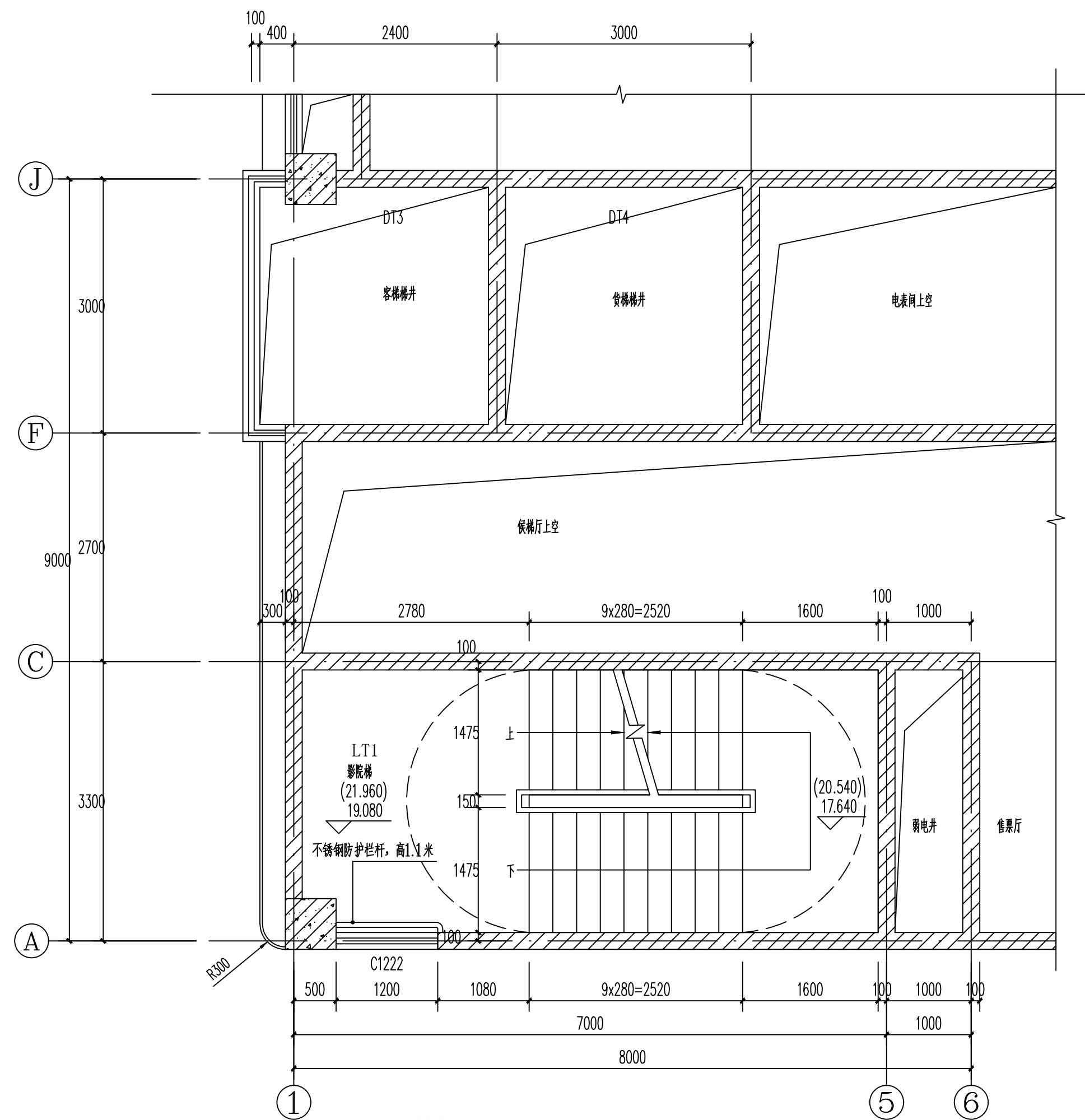
LT1楼梯间H=19.08 (21.96)处平面图 1:50
