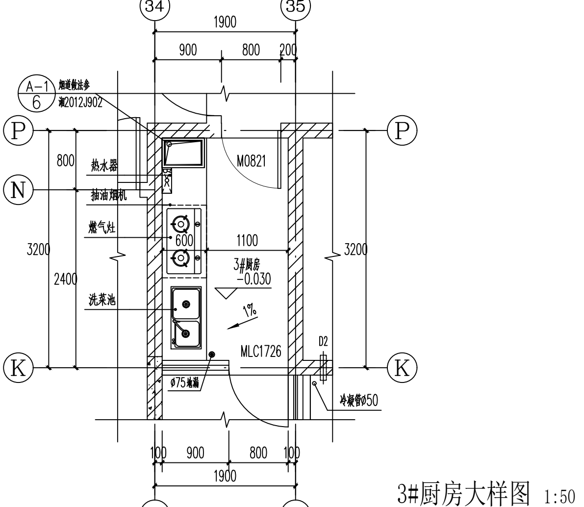
3#厨房大样图 1:50
