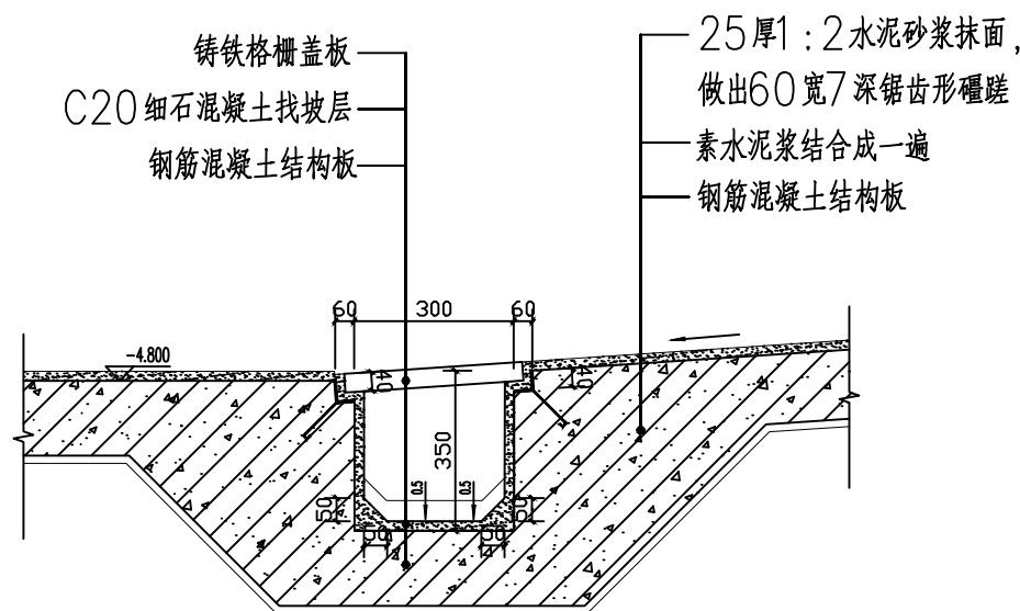
② 车道室内地面截水沟大样 1:25
