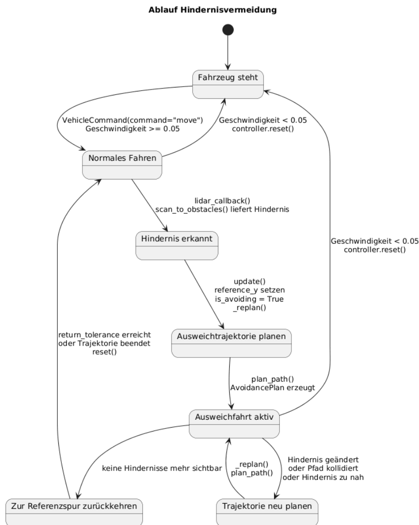
Abbildung 2: Zustandsdiagramm: Ausweichen
