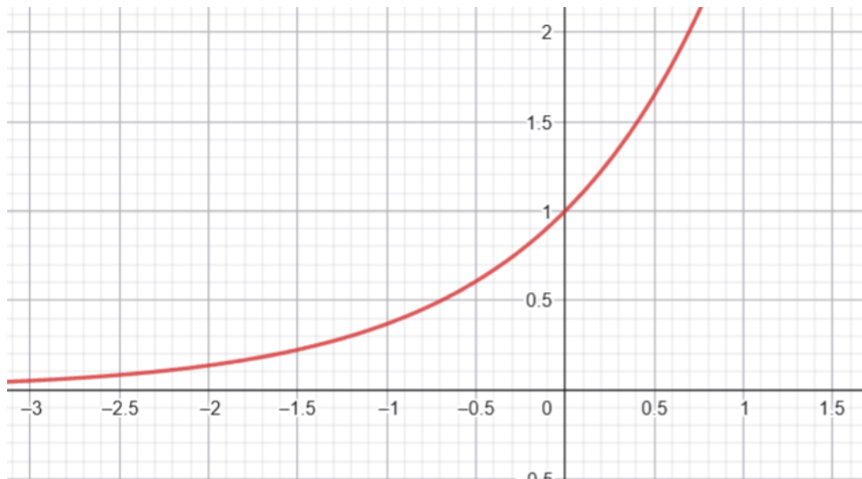
Abbildung 4: Exponential Funktion
