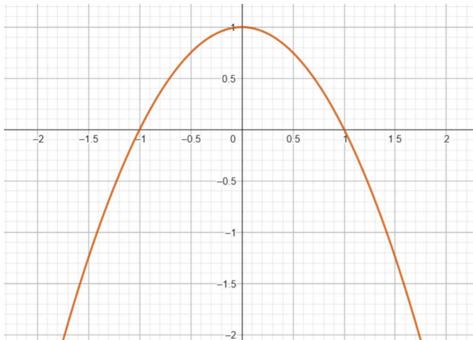
Abbildung 3: Parabel Funktion
