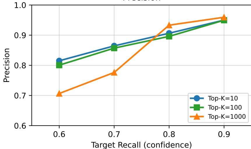
Precision
