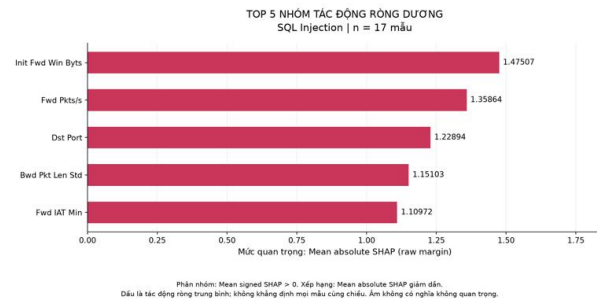
Hình 1. Top 5 SHAP global của bốn lớp đại diện. SQL Injection chỉ có 17 flow nên chỉ có ý nghĩa minh họa.
