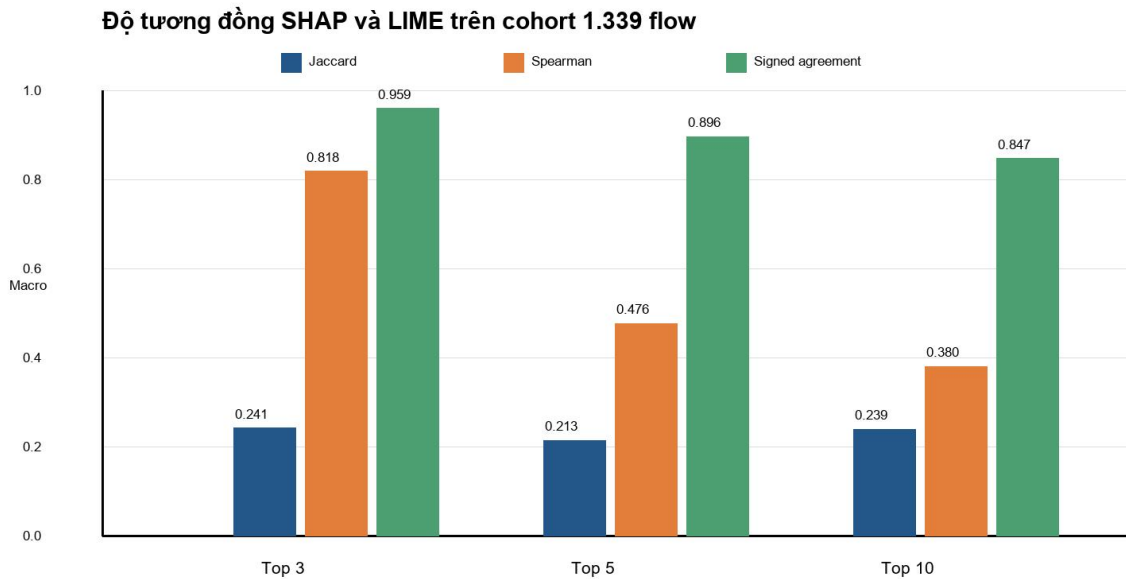
Hình 2. Agreement SHAP - LIME theo Top k trên cùng cohort 1.339 flow.
