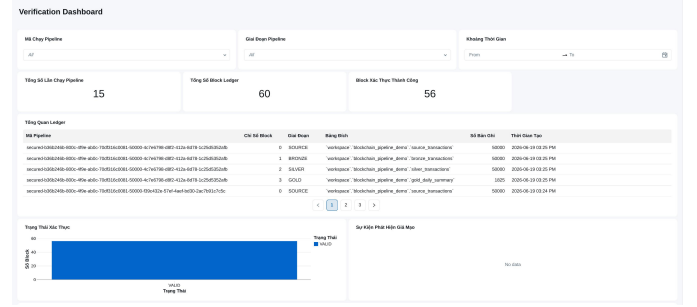
Fig. 4. Verification Dashboard (xuất từ Databricks SQL) ở trạng thái sạch: 15 lần chạy pipeline, 60 block ledger, 56 block xác thực thành công; biểu đồ trạng thái chỉ ghi nhận outcome VALID và mục “Sự Kiện Phát Hiện Giả Mạo” không có dữ liệu trong bộ lọc hiện tại, đối chiếu với hàng NONE/VALID của Bảng IV.
