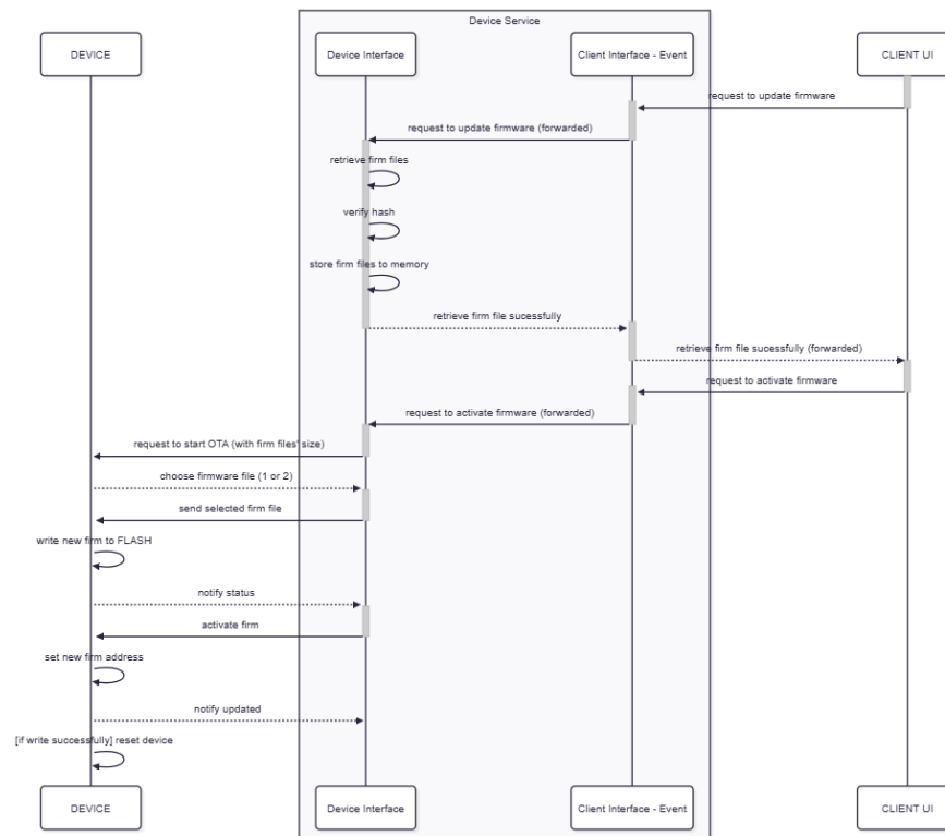
Hình 3.15. Trình tự giao tiếp phần mềm trong trường hợp thực hiện OTA
