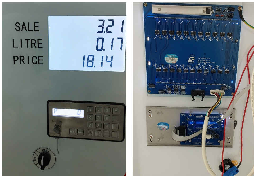
Hình 1.2. Màn hình và mạch phần cứng màn hình cây xăng hãng ZCheng
