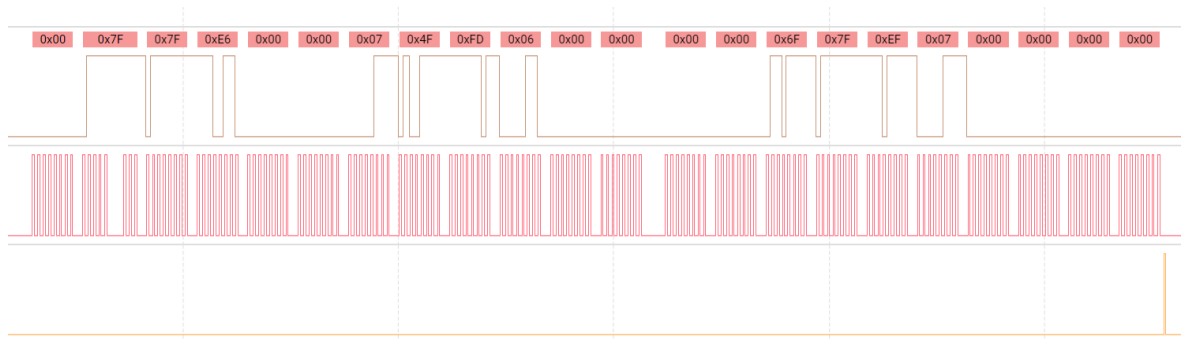
Hình 1.3. Một mẫu tín hiệu màn hình thu được sử dụng Logic Analyzer
