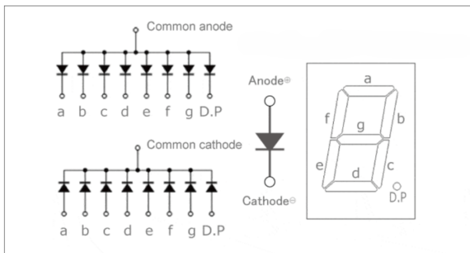
Hình 2.3. Cấu trúc của LED 7 thanh
