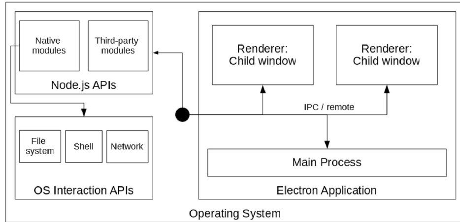
Hình 3.17. Giao tiếp giữa các process của ứng dụng thông qua IPC
