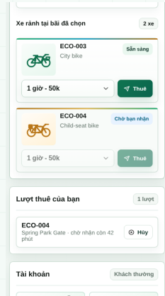
Chọn xe
