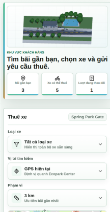
Tổng quan
