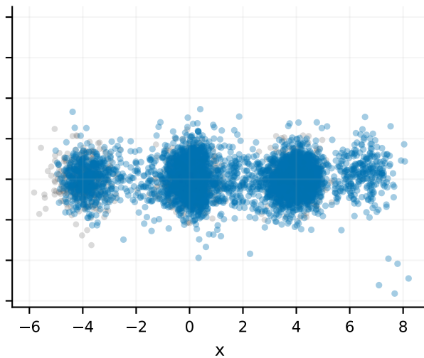
seed 43; EMD=1.826
