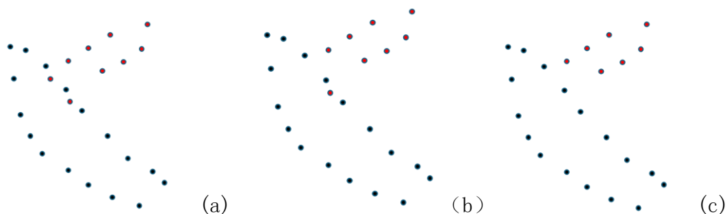
图 2.8 分支型相交断层
