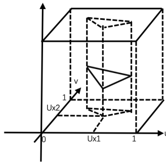
(b)三角面UV映射
