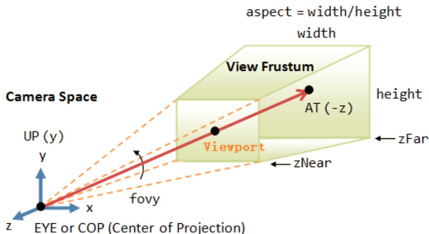
图3.3 透视相机示意图
