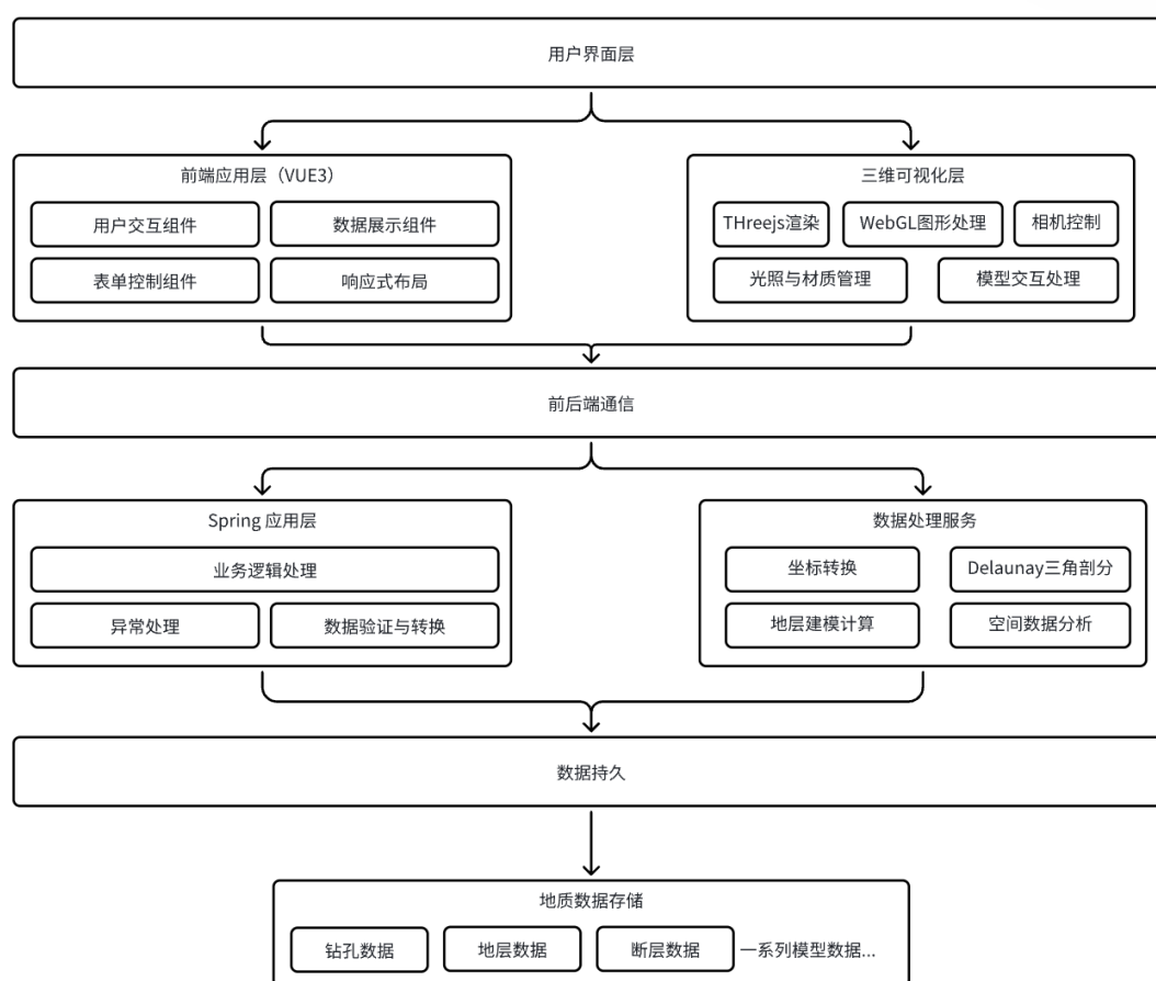
图4.1 系统结构图
