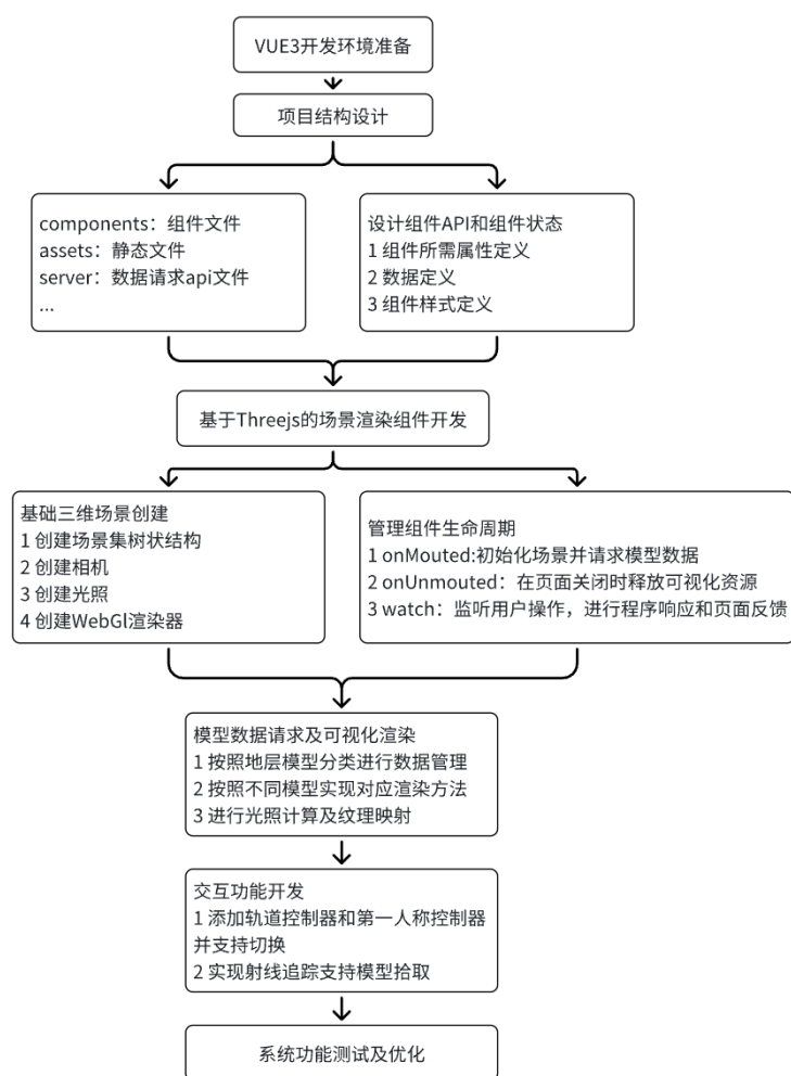
图4.13 VUE3框架开发流程图
