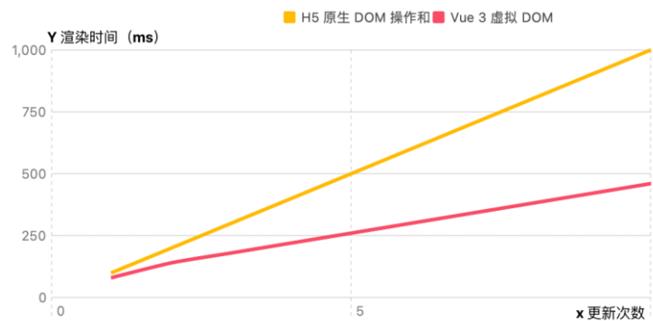
图4.14 DOM操作频次对比
