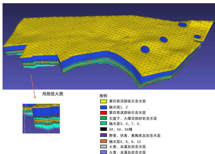
图5.1 三维地层模型图例示意
