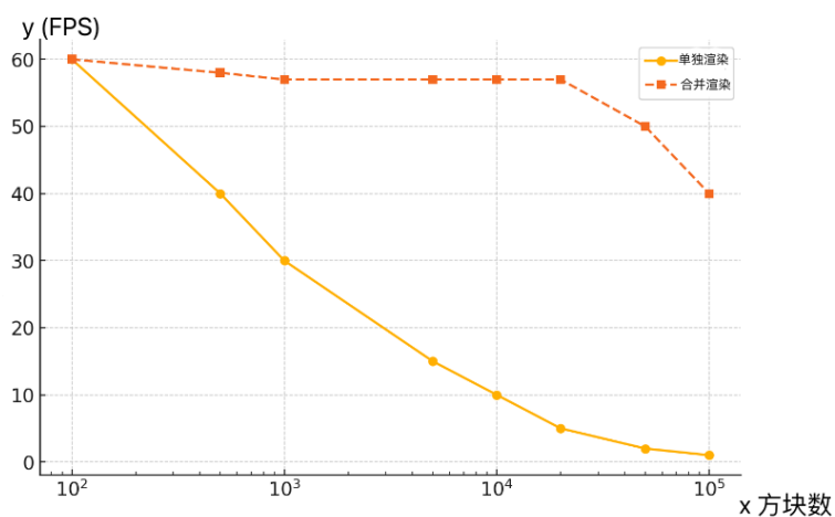
图4.11 随模型增多不同渲染方式对FPS的影响
