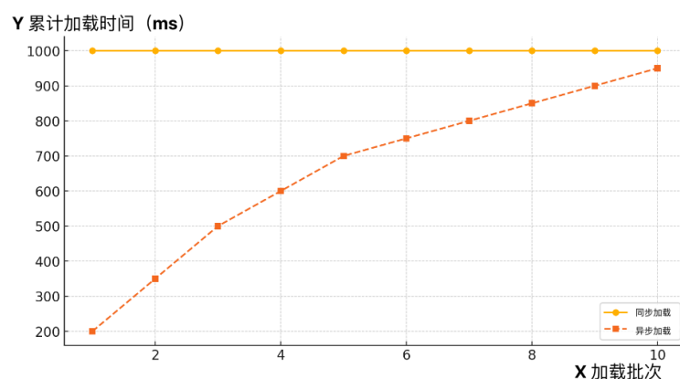
图4.16 分批次累计加载时间对比
