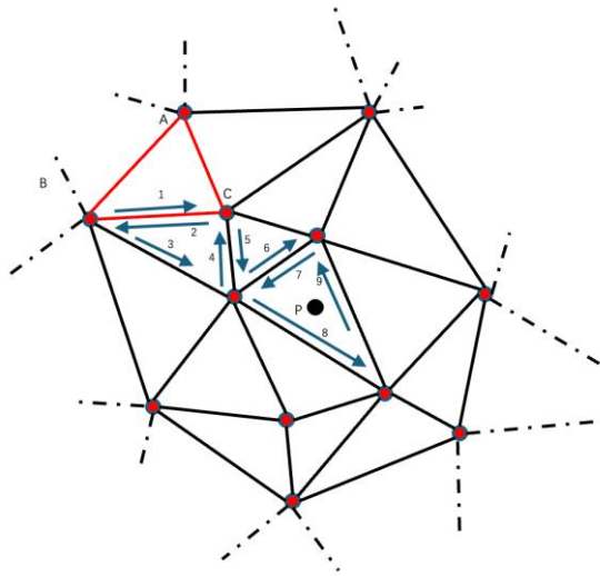
图 2.2 定位包围三角形网格局部示例
