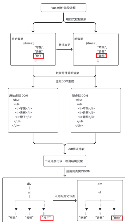
图4.15 虚拟DOM操作示意图
