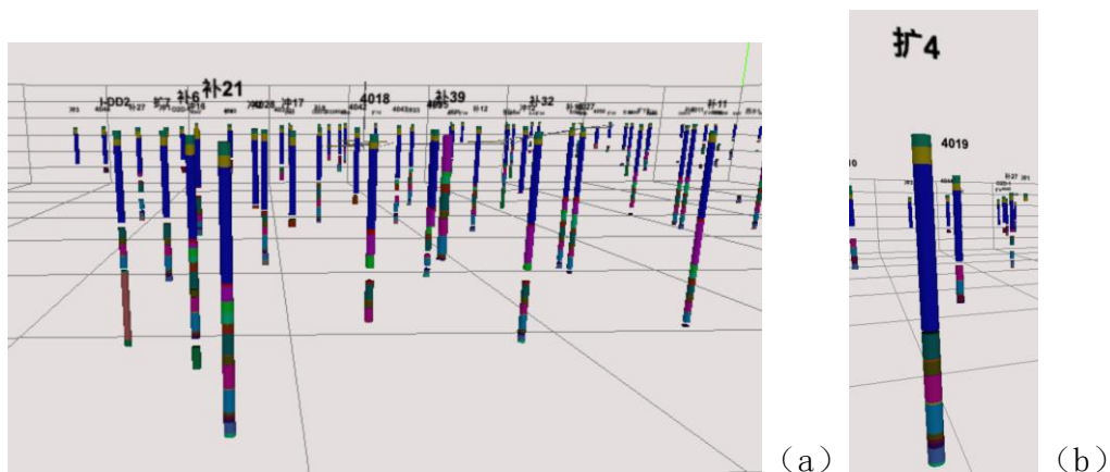
图4.6 钻孔模型可视化和局部展示
