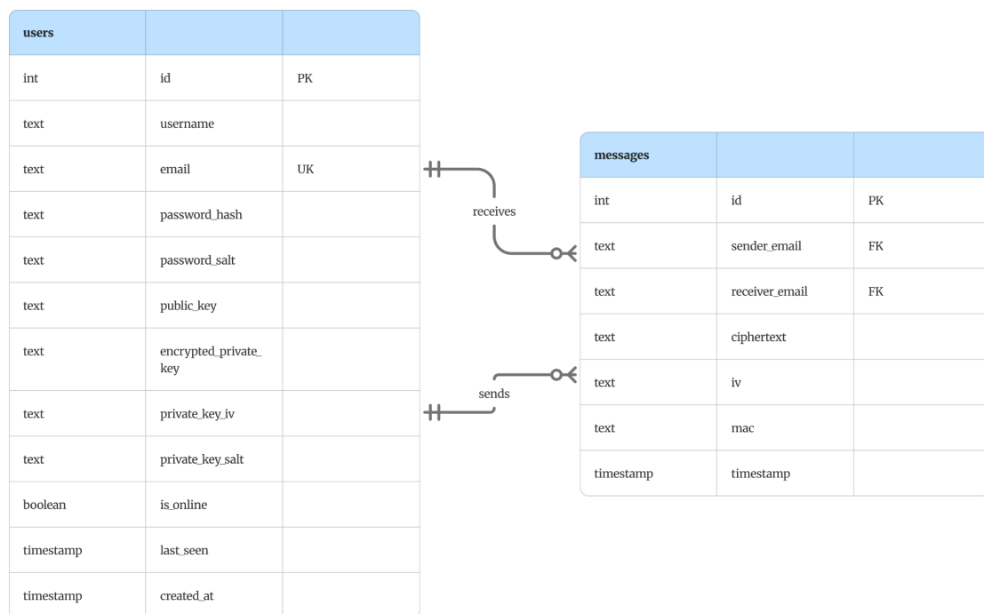
Gambar 3.2 ERD database
