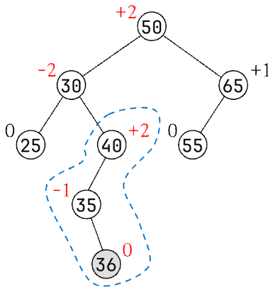
(a) 단순 삽입 결과
