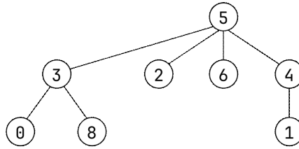
그림 10.11: union(3, 5)의 수행
