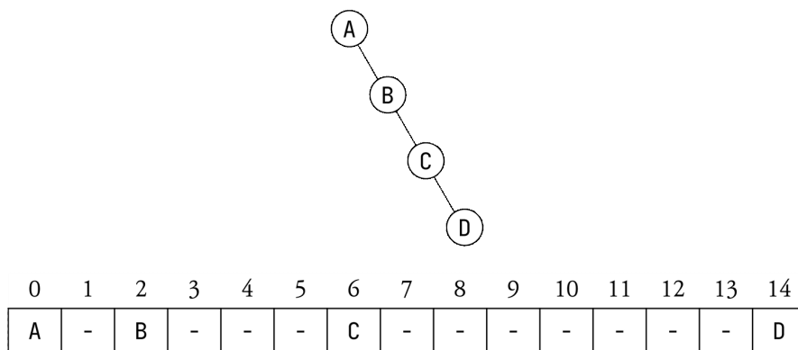
그림 9.9: 경사 이진 트리의 배열 표현
