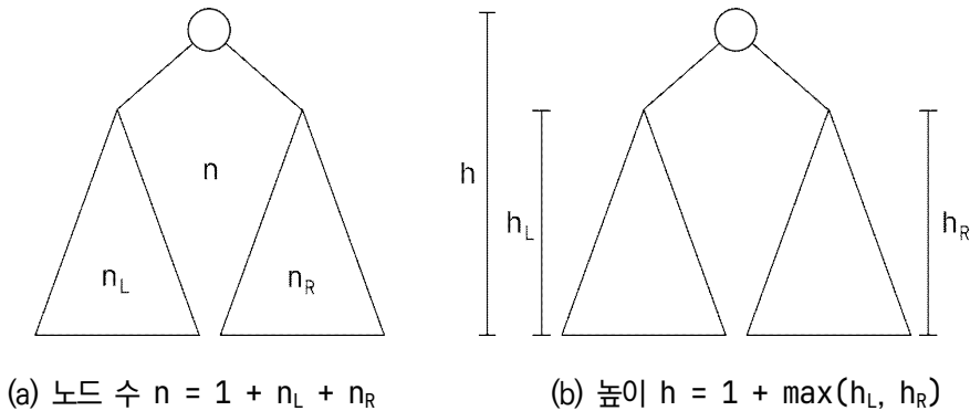
그림 9.12: 이진 트리의 크기와 높이
