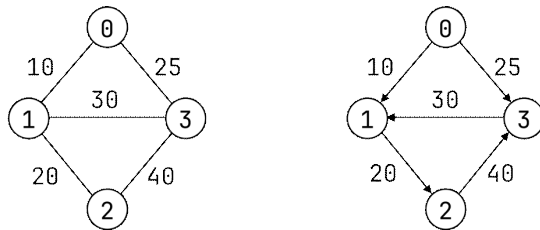
그림 12.1: 가중치 그래프의 예
