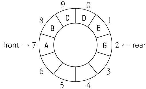
그림 6.6: 원형 큐의 예
