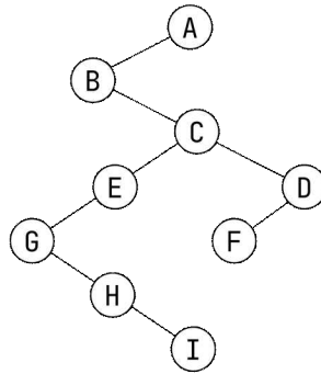
그림 9.16: 그림 9.15의 트리에 대한 이진 트리 표현
