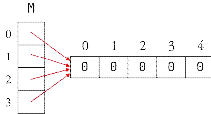
그림 3.8: 동일한 리스트를 참조하는 리스트
