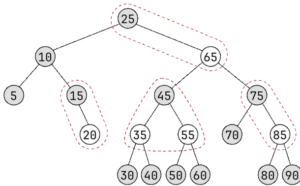
그림 13.19: 그림 13.17의 2-3-4 트리가 변환된 레드-블랙 트리
