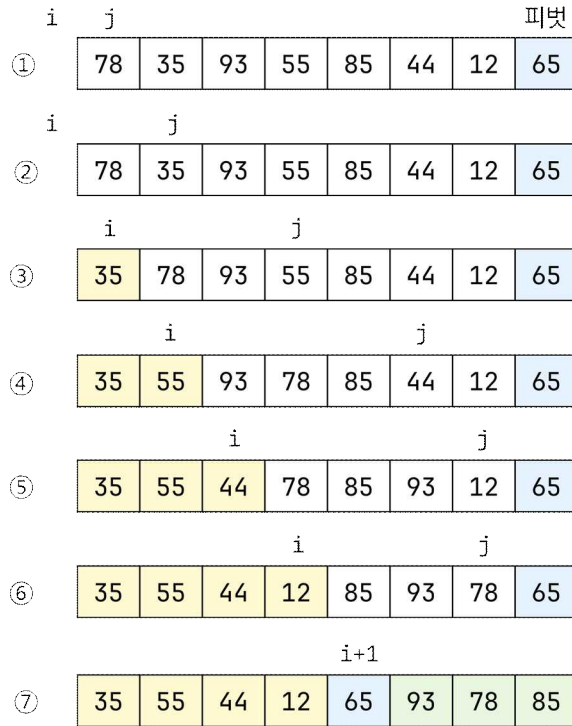
그림 8.6: 퀵 정렬에서 분할을 수행하는 예
