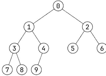
그림 9.7: 10개의 노드를 가진 완전 이진 트리
