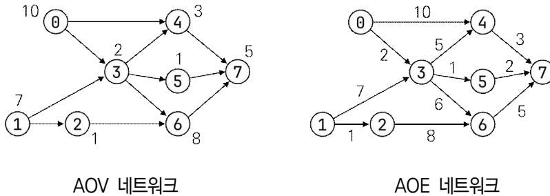
그림 12.13: 작업 네트워크의 예
