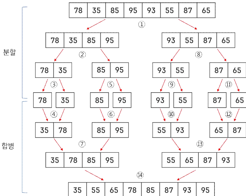
그림 8.3: 합병 정렬의 수행 과정
