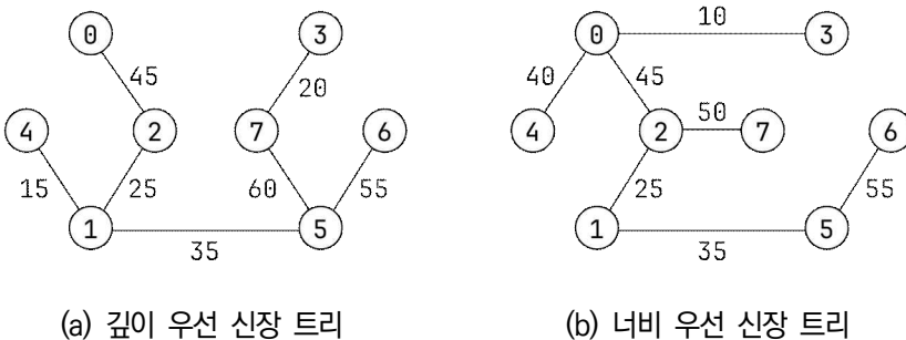
그림 12.5: 그림 12.4의 가중치 그래프에 대한 신장 트리
