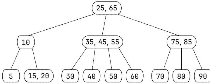
그림 13.17: 차수가 4인 B-트리의 예
