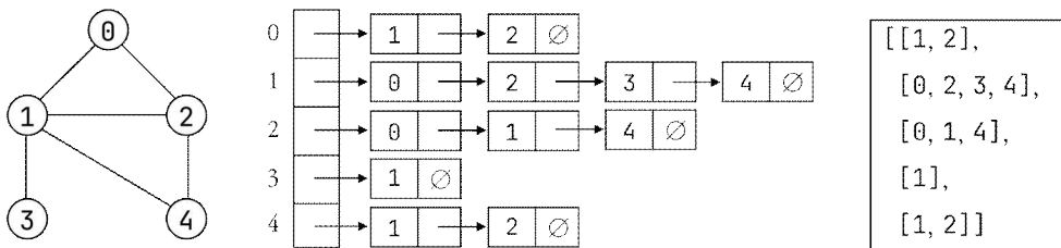
그림 11.11: 무향 그래프의 인접 리스트 (연결리스트와 파이썬 리스트)
