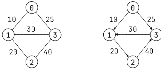
그림 12.1: 가중치 그래프의 예
