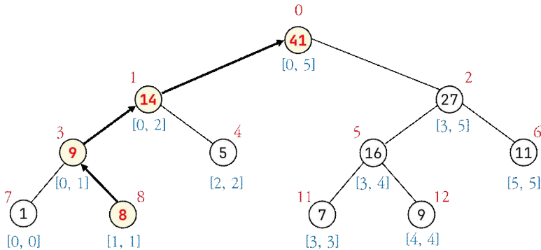
그림 10.17: 프로그램 10.15의 수행에서 update() 의 복귀 과정
