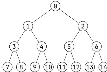
(b) 포화 이진 트리
