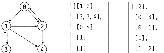
그림 11.12: 방향 그래프의 인접 리스트와 역 인접 리스트
