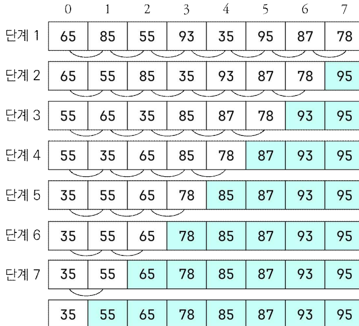
그림 3.11: 버블 정렬 알고리즘의 수행 과정
