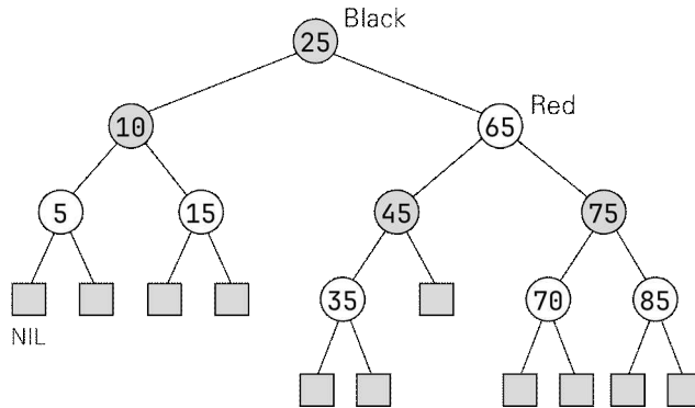
그림 13.9: 레드-블랙 트리의 예
