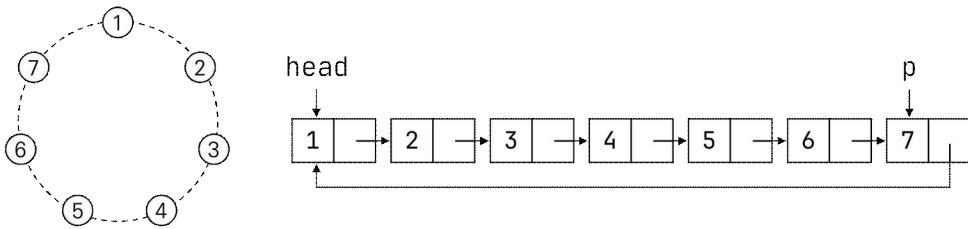
그림 7.8: 요셉 문제를 위한 원형 연결리스트의 예
