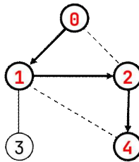
(e) 정점 1까지 퇴각한다
