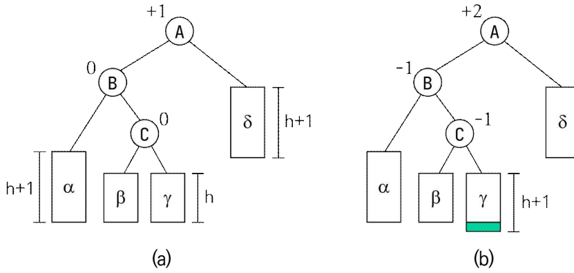
그림 13.4: LR 유형의 예
