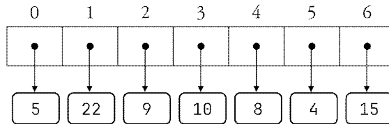
그림 3.4: 파이썬 리스트의 참조 배열 구조
