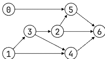
그림 11.18: 방향 비순환 그래프의 예
