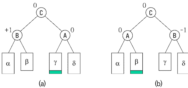
그림 13.6: LR 회전과 RL 회전 변환의 예
