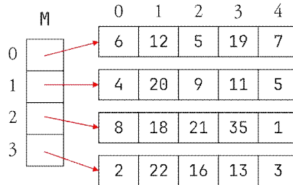
그림 3.7: 행렬 데이터를 위한 리스트의 리스트 구조
