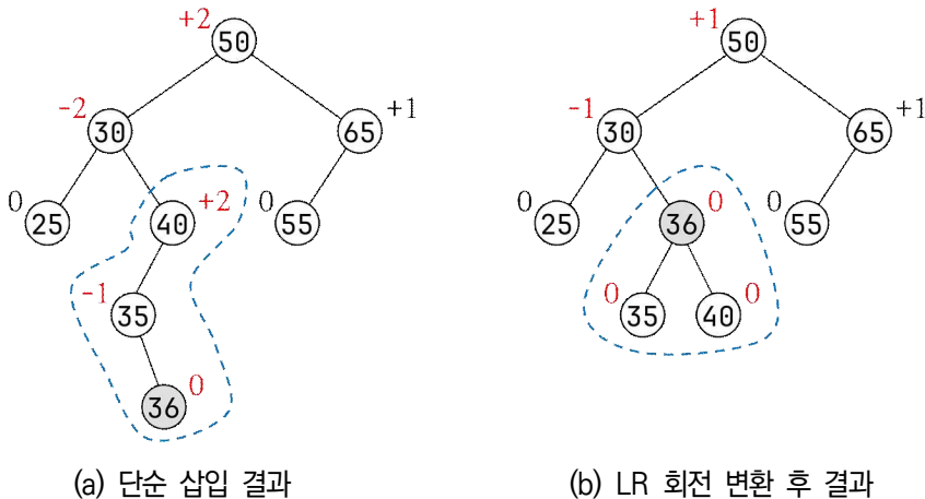
그림 13.7: 그림 13.1의 AVL 트리에서 노드 36의 삽입 과정
