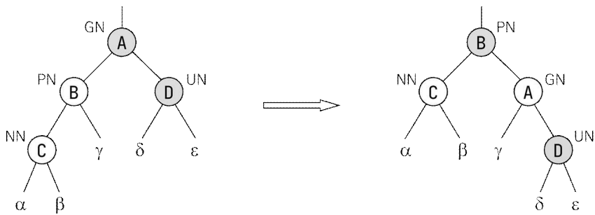
그림 13.13: LLb 유형에 대한 회전 변환 및 색상 변경
