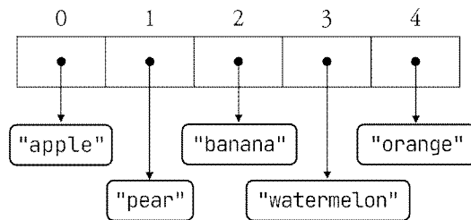
그림 3.3: 참조 배열의 예
