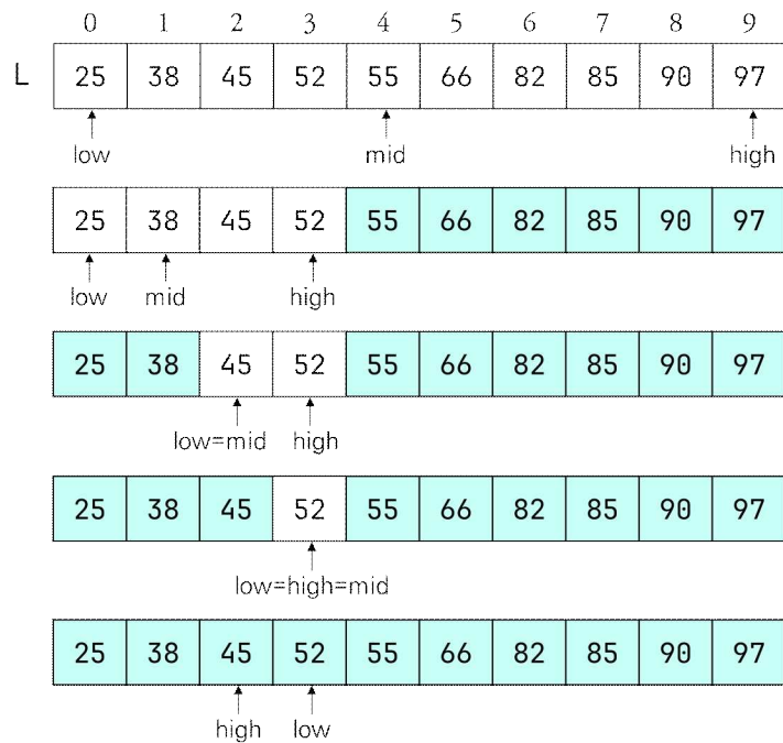
그림 4.7: 리스트 L에서 탐색값 50을 찾는 이진 탐색의 수행 예 (탐색 실패)
