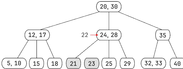
(a) 각각 21과 23을 가진 분리된 노드와 부모 노드에 22를 삽입하려는 과정
