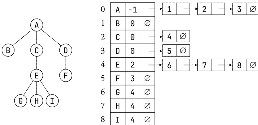
그림 9.17: 자식 리스트-부모 포인터 표현
