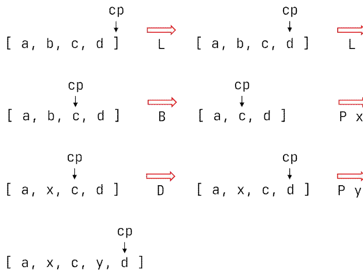
그림 7.15: 연결리스트에서 편집 명령을 수행하는 과정
