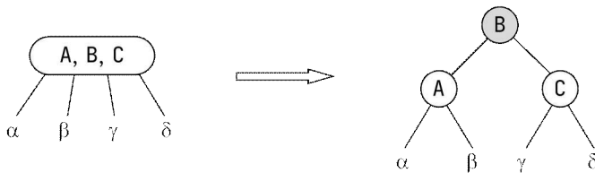
(b) 3-노드의 변환
