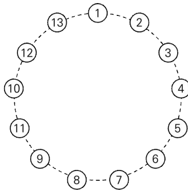
그림 6.10: 요셉 문제 n=13 , k=3
