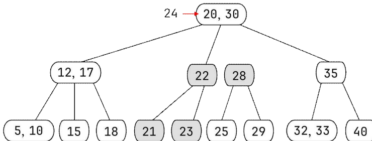
(b) 각각 22와 28을 가진 분리된 노드와 부모 노드에 24를 삽입하려는 과정
