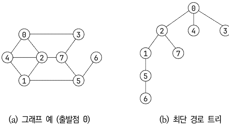
그림 11.17: 최단 경로 트리의 예
