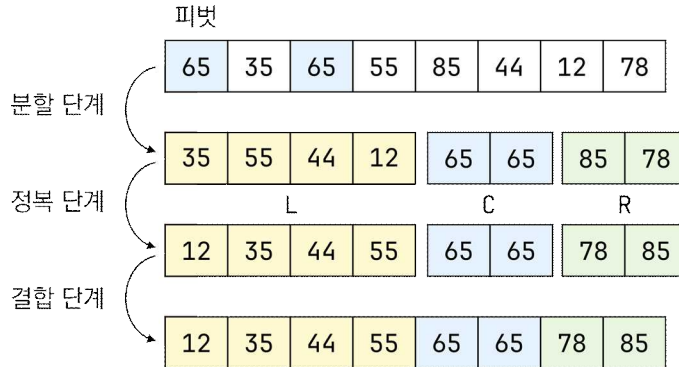
그림 8.4: 퀵 정렬의 기본 전략
