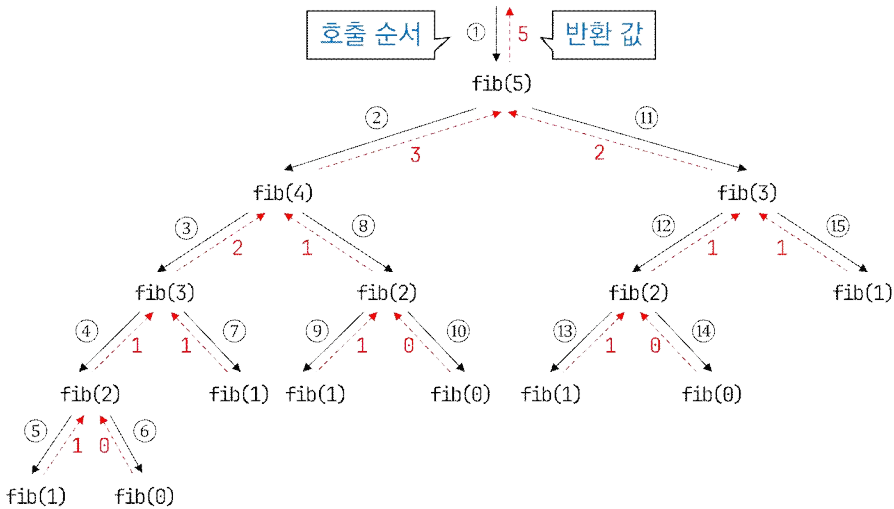
그림 4.2: 재귀 함수 fib()의 수행 과정
