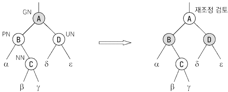
그림 13.12: LRr 유형에 대한 색상 변경
