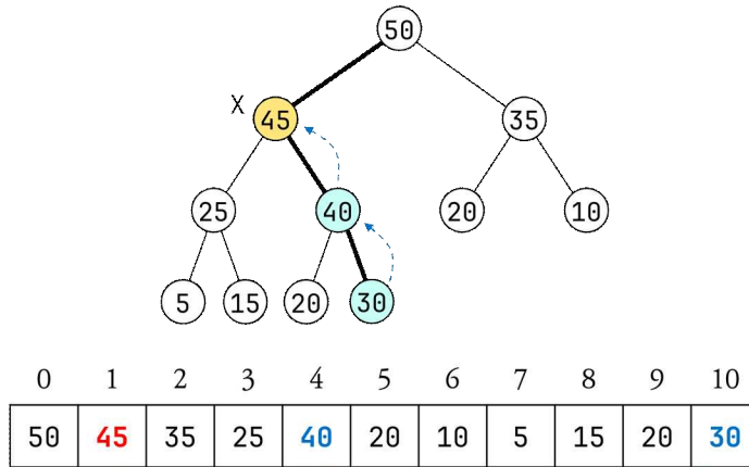
그림 10.6: 그림 10.5의 힙에 원소 '45'의 삽입
