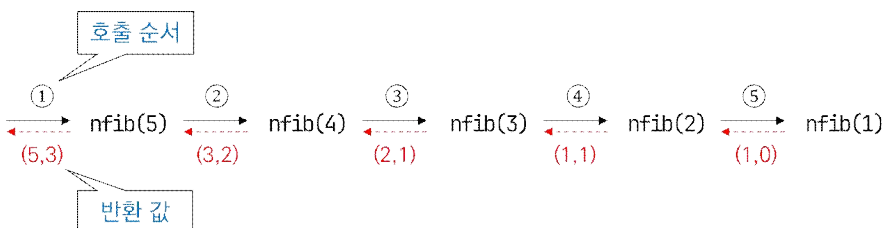
그림 4.3: 재귀 함수 nfib() 의 수행 과정
