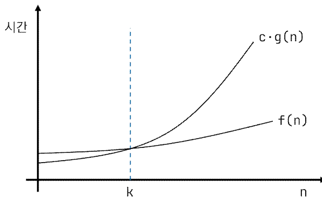
그림 1.1: O -표기법의 정의
