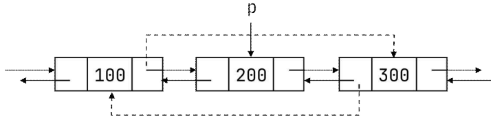
그림 7.13: 원형 이중 연결리스트에서 노드의 삭제
