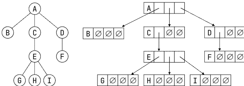
그림 9.14: 트리의 다중 링크 표현
