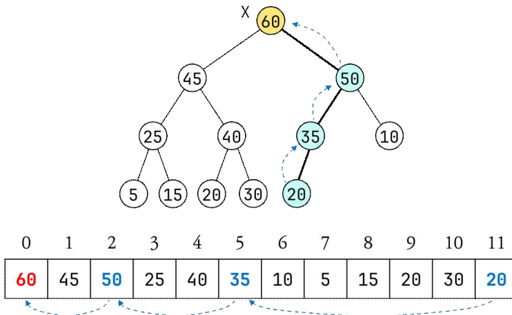
그림 10.7: 그림 10.6의 힙에 원소 '60'의 삽입
