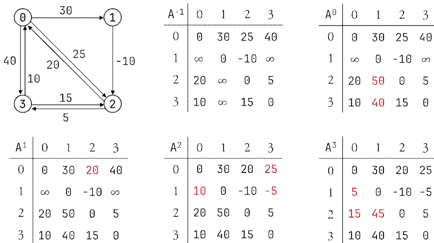
그림 12.12: 플로이드-와샬 알고리즘의 수행 과정
