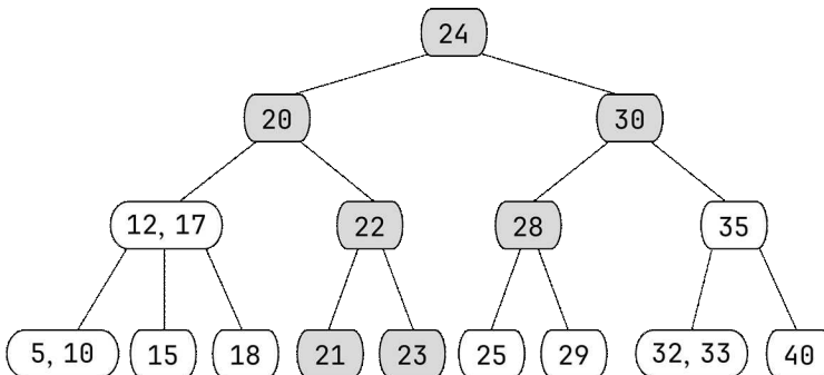
(c) 각각 20과 30을 가진 분리된 노드와 새로운 루트 노드가 생성되는 과정
