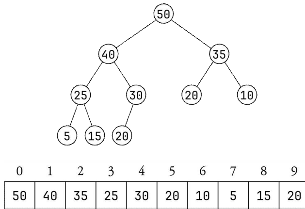
그림 10.5: 최대 힙과 배열 표현 예
