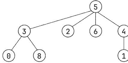
그림 10.11: union(3, 5)의 수행
