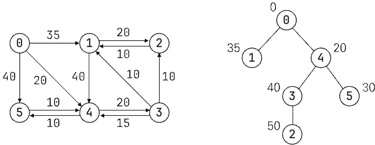
그림 12.9: 가중치 방향 그래프와 최단 경로 트리
