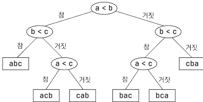
그림 9.19: 세 숫자의 정렬을 위한 결정 트리
