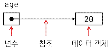
그림 2.1: 배정 연산 ' age = 20 '으로 생성되는 변수와 데이터 객체
