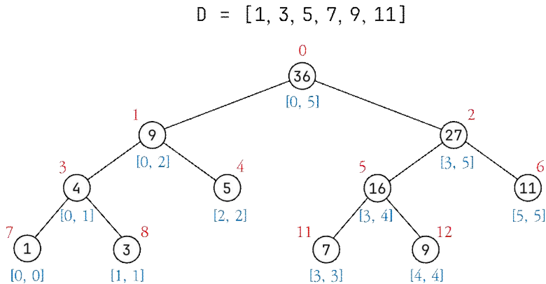
그림 10.15: 세그먼트 트리에서 노드의 구간 정보
