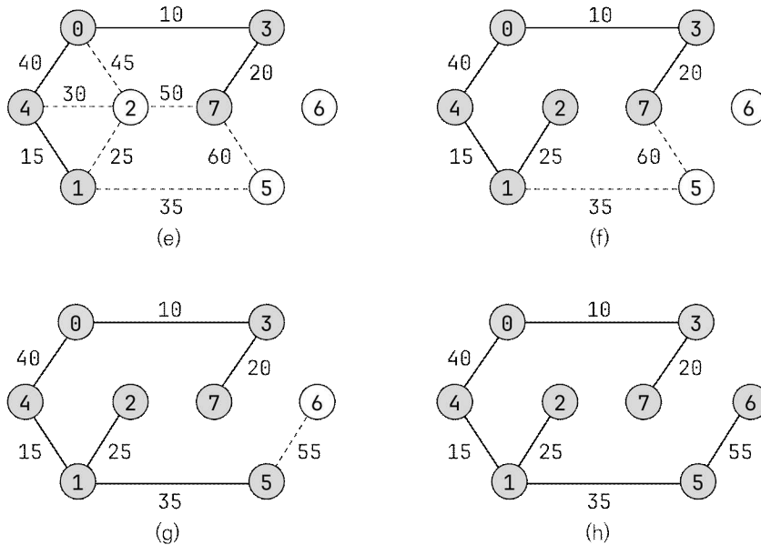
그림 12.7: 그림 12.4의 그래프에 대한 프림 알고리즘의 수행 과정
