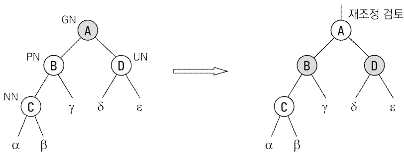
그림 13.11: LLr 유형에 대한 색상 변경
