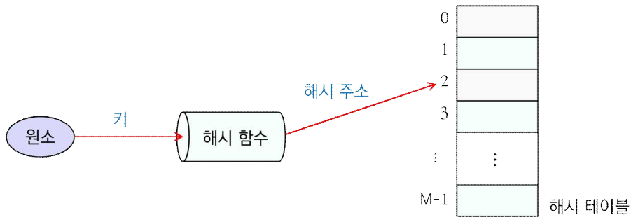
그림 13.23: 해싱의 기본적인 동작 원리
