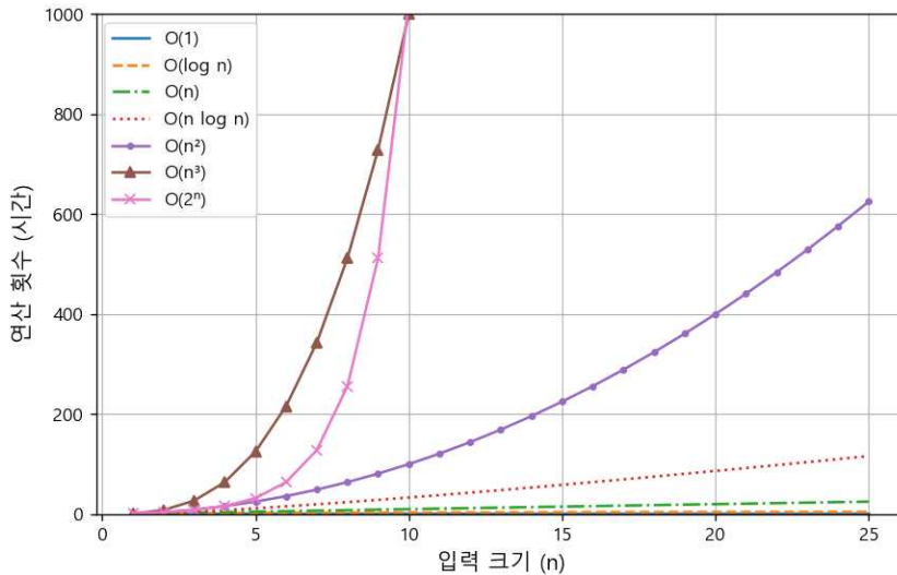
그림 1.3: 시간복잡도 함수의 증가율 비교
