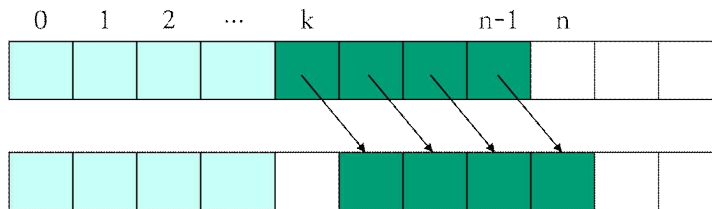
그림 3.5: insert(k, item)의 수행에서 요소들의 이동 작업
