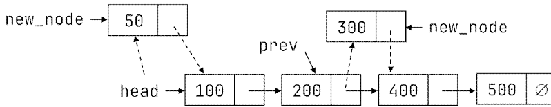
그림 7.3: 연결리스트에서 삽입 연산의 수행
