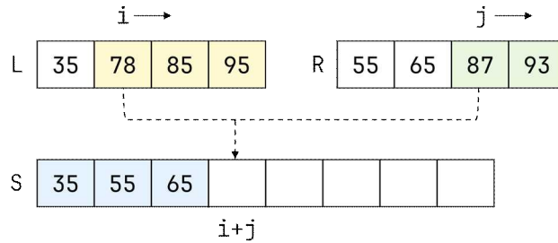
그림 8.2: 합병 진행 과정
