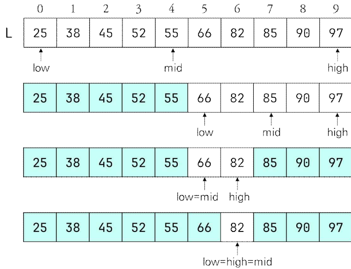
그림 4.6: 리스트 L에서 탐색값 82를 찾는 이진 탐색의 수행 예 (탐색 성공)
