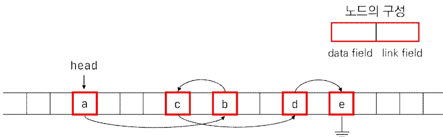
그림 7.1: 메모리에 저장된 연결리스트의 모습
