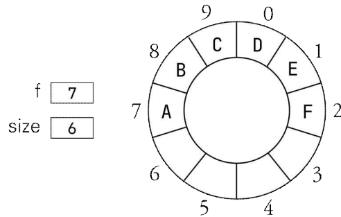
그림 6.6: 원형 큐의 예
