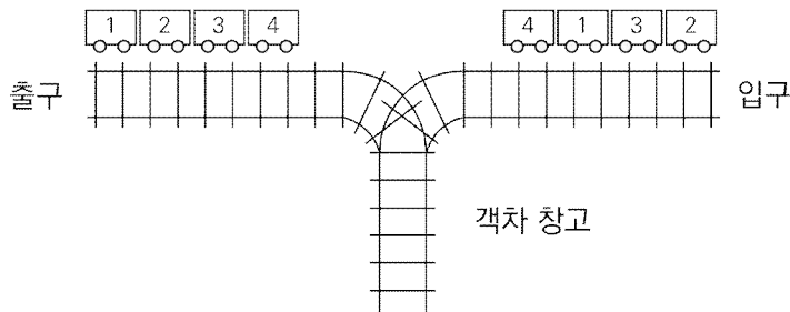
그림 5.4: 객차 재배치 문제
