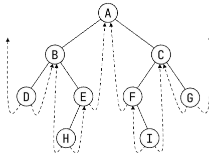
〈스레드 이진 트리〉
