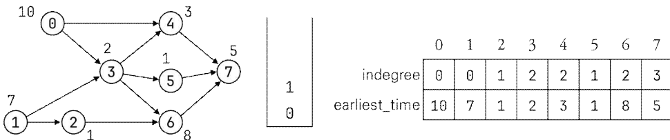
(a) 초기 상태: 스택에 0과 1 삽입
