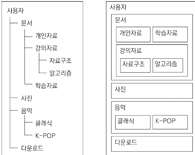
그림 9.3: 계층적인 구조의 표현 예
