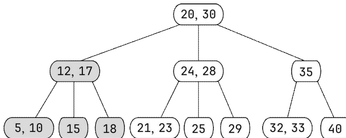
그림 13.21: 두 키 5와 18이 차례로 삽입된 후의 2-3 트리
