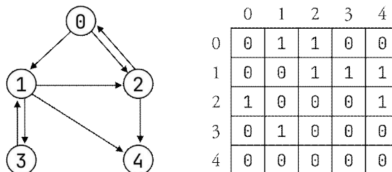
그림 11.10: 방향 그래프의 인접 행렬
