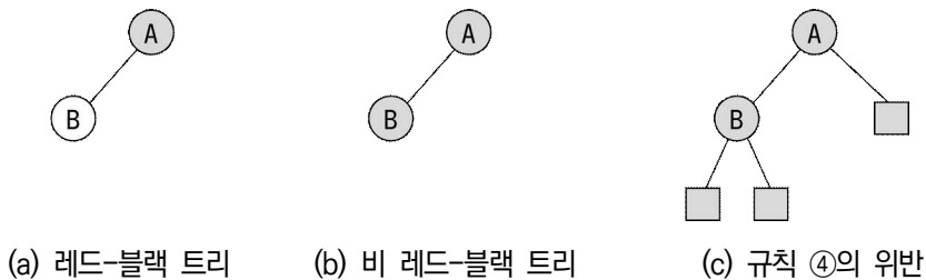
그림 13.10: 레드-블랙 트리에서 NIL 노드 도입
