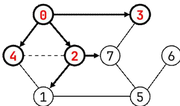
(c) 정점 1, 7을 방문함
