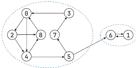
그림 11.6: 그림 11.4의 그래프 G_2 의 강 연결 요소
