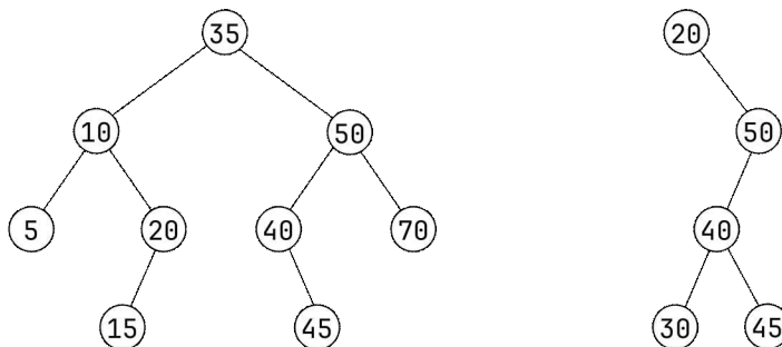
그림 10.1: 이진 탐색 트리의 예
