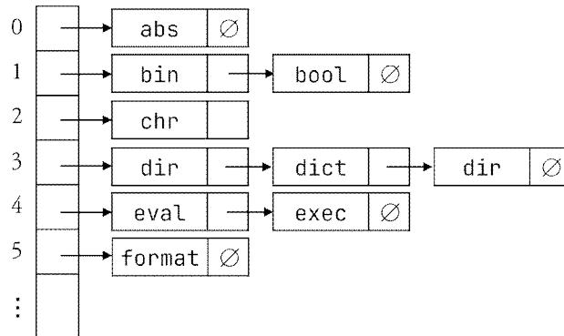
그림 13.24: 해시 체인법의 예 (해시 주소가 키의 첫 문자의 알파벳 순서인 경우)
