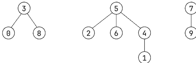
그림 10.10: 분리된 집합의 트리 표현
