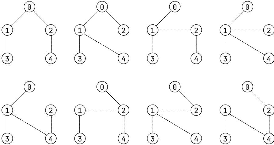
그림 11.15: 그림 11.13 그래프의 모든 신장 트리
