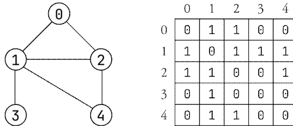
그림 11.9: 무향 그래프의 인접 행렬
