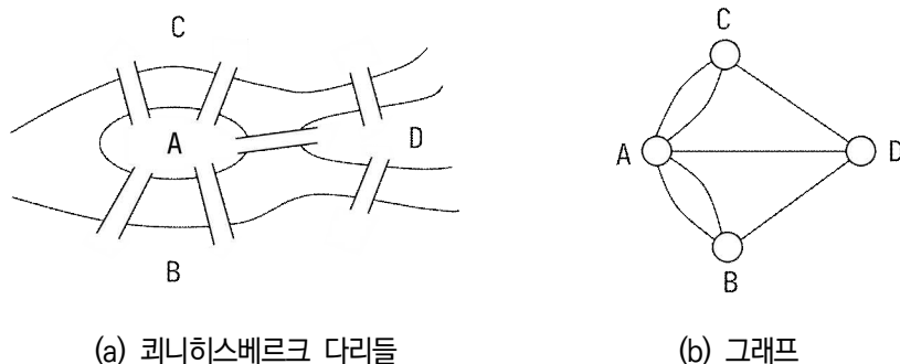
그림 11.1: 코니히스베르크의 다리들과 그래프 모델
