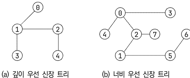
그림 11.16: 표 11.2와 표 11.3의 탐색 순서에 의해 생성된 신장 트리
