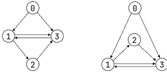
그림 11.3: 방향 에지를 가진 그래프
