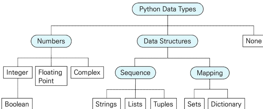
그림 9.2: 파이썬 자료형의 계층 구조
