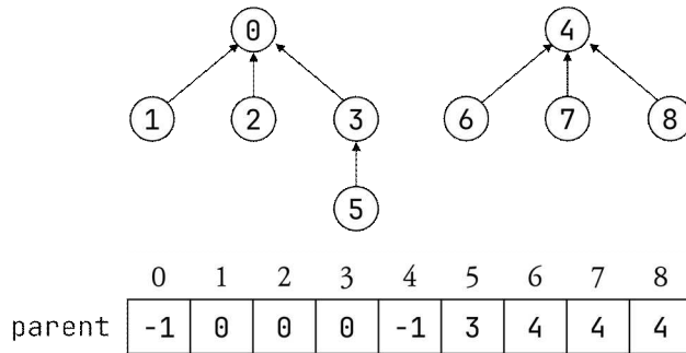
그림 9.18: 부모 포인터 배열
