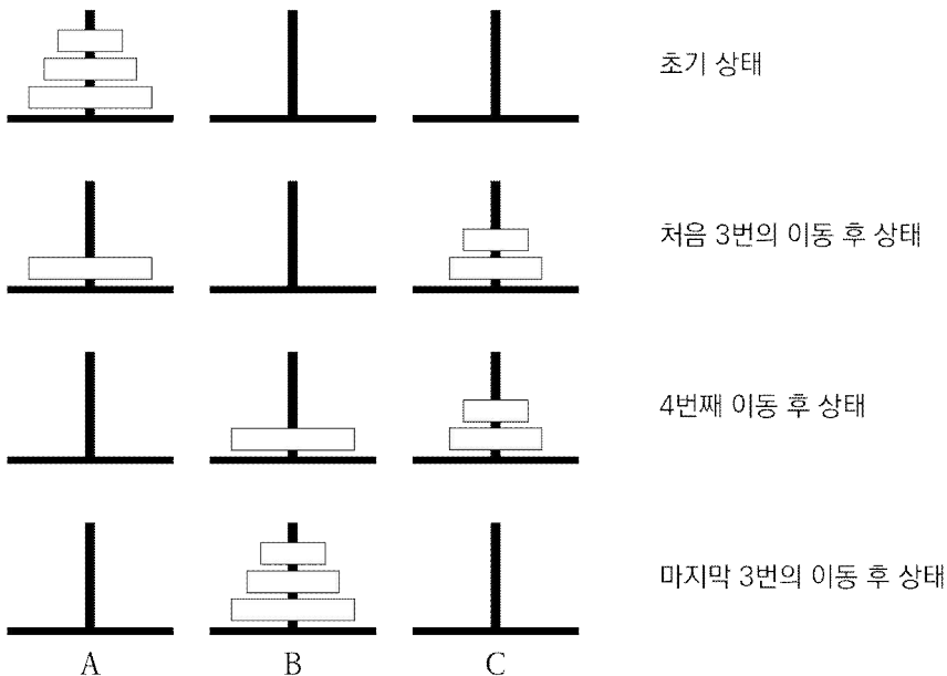
그림 4.5: 3개의 원반을 목표 기둥으로 옮기는 과정
