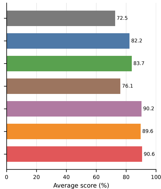
Image-AP
