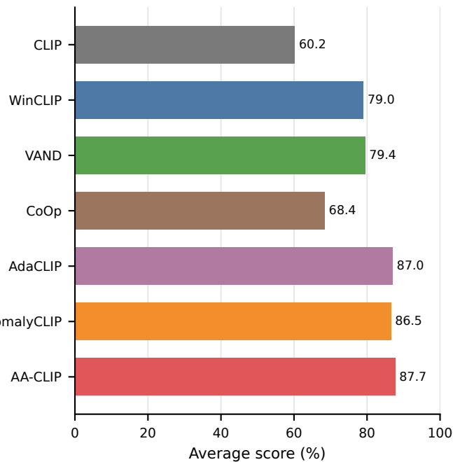
Image-AUROC
