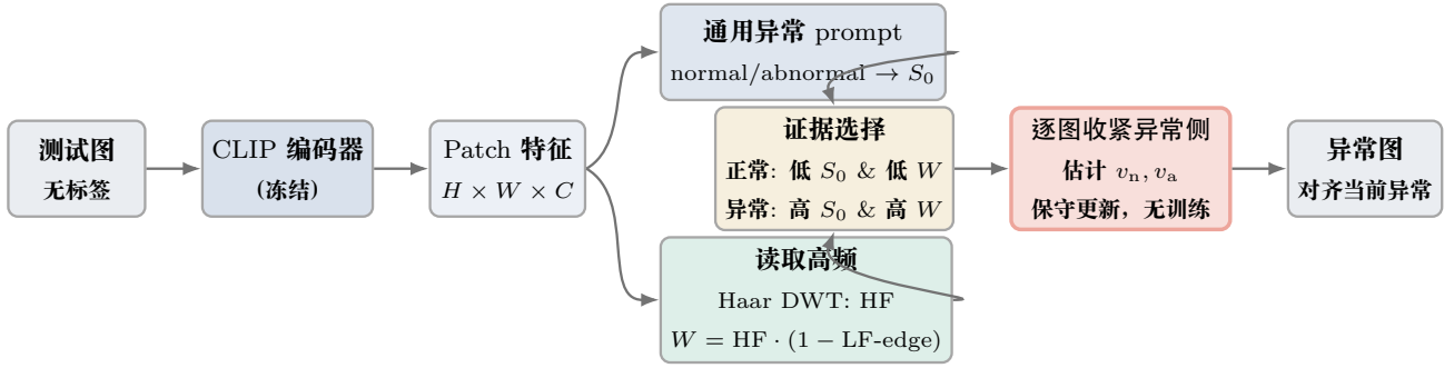
图 2: 整体框架。测试图经冻结的 CLIP 得到 patch 特征; 通用异常 prompt 给出语义分数 S_0 , 频率支经 Haar DWT 给出高频依据 HF/W。两者汇入证据选择, 据此在测试阶段逐图收紧过宽的异常侧文本表示 (保守更新, 无训练), 最后重算得到与当前图像实际异常对齐的异常图。W 提供独立于 CLIP 语义的高频依据。
