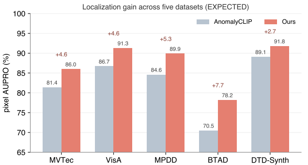
图 3: 五个基准上的像素级 AUPRO: 通用 prompt 基线 vs. Ours (EXPECTED)。逐图收紧异常侧在所有数据集上带来一致的定位增益, 纹理主导的基准 (如 BTAD) 增益最大。
