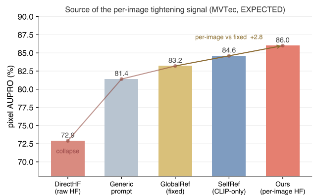
图 4: 收紧信号的来源(MVTec 像素 AUPRO, EXPECTED)。直接读高频 (DirectHF) 崩溃；全局固定参照差于逐图；三档呈单调 \text{GlobalRef} < \text{SelfRef} < \text{Ours} 。
