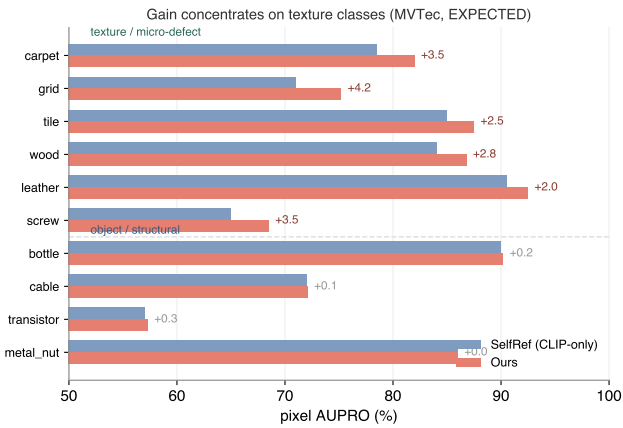
图 5: 分类像素 AUPRO: Ours vs. SelfRef (MVTec, EXPECTED)。增益集中在纹理 / 微缺陷类, 物体类持平。
