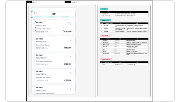
04 화면설계서
