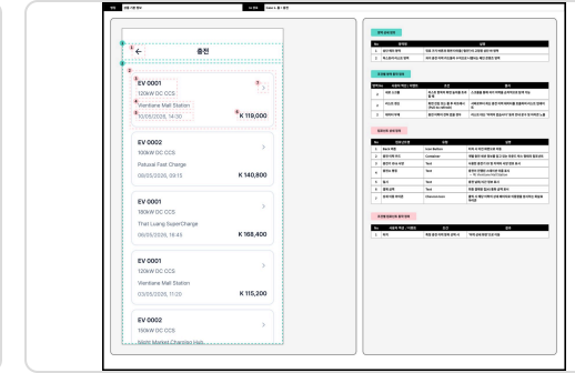
04 화면설계서
