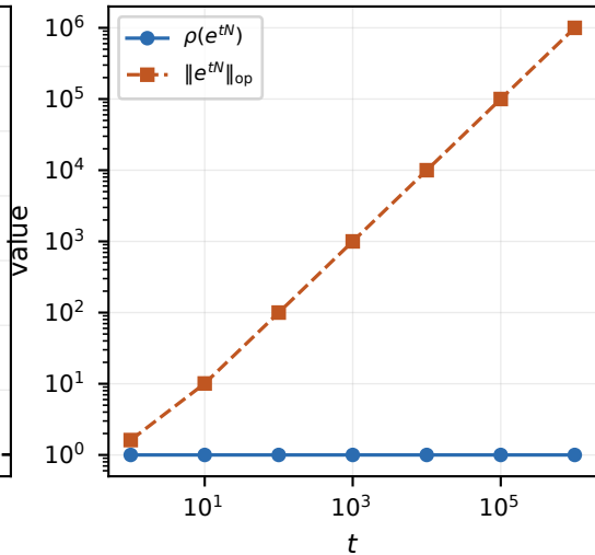
Nilpotent N : \rho = 1 while \|\cdot\|_{\text{op}} \sim t
