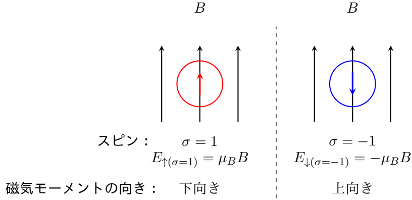
図 3.1: 一様磁場 B 中にある単一のスピンエネルギー固有状態．スピン上向きを \sigma = 1 ，下向きを \sigma = -1 と表す．磁気モーメントが磁場と平行でスピンの磁場と反平行なときエネルギーは安定である．
