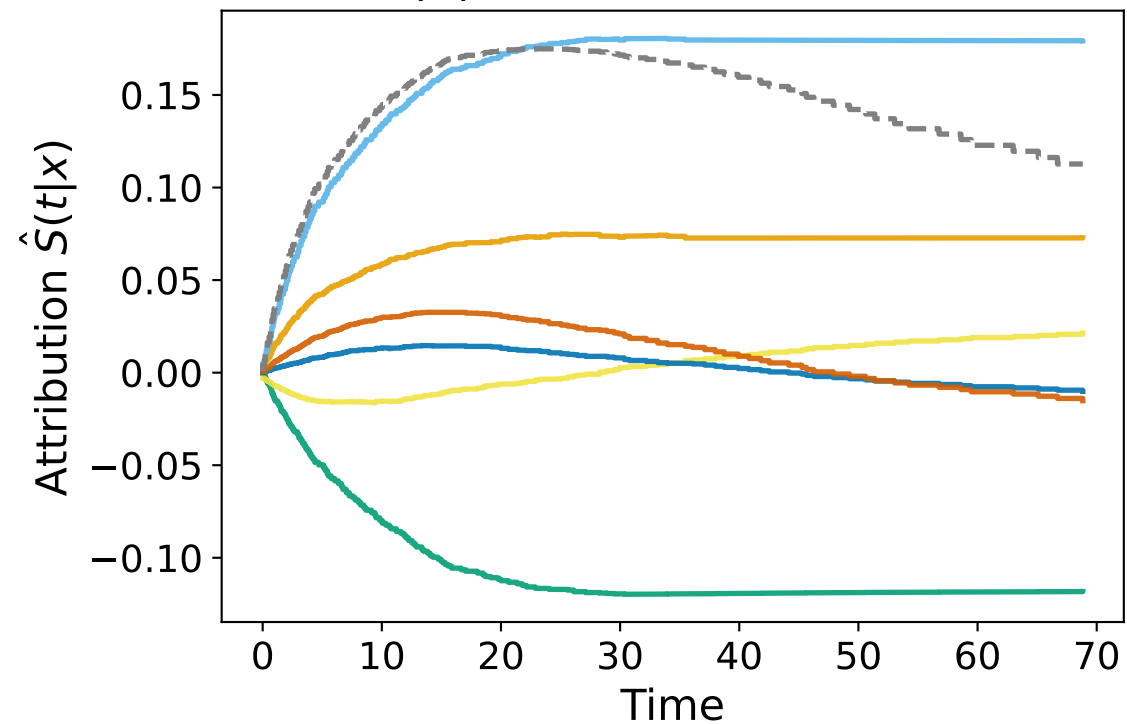
CoxPH: (8) GenAdd TI Inter
