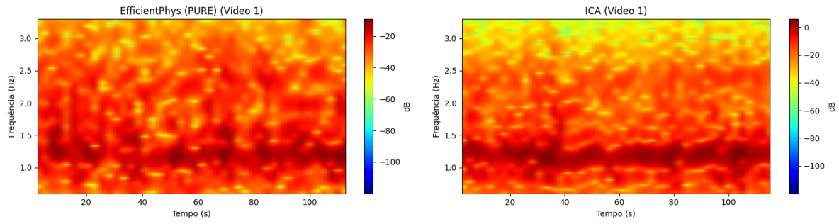
Figura 15: Espectrogramas dos sinais cujas estimativas de frequência cardíaca resultaram no menor erro médio absoluto.
