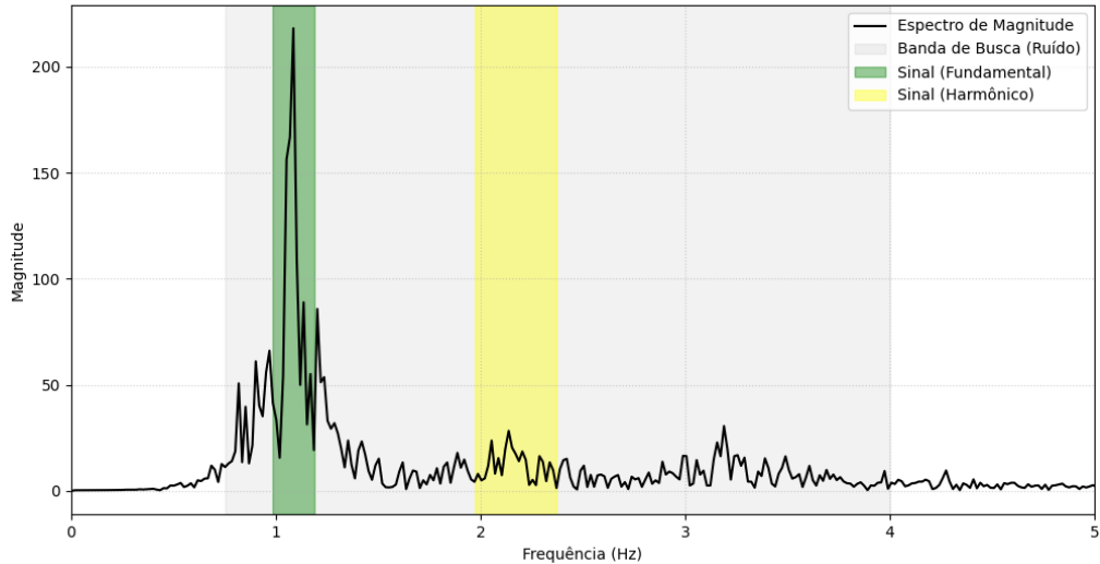
Figura 10: Cálculo da relação sinal-ruído Fonte: autoria própria
